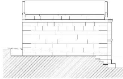
YAN GÖRÜNÜŞ
