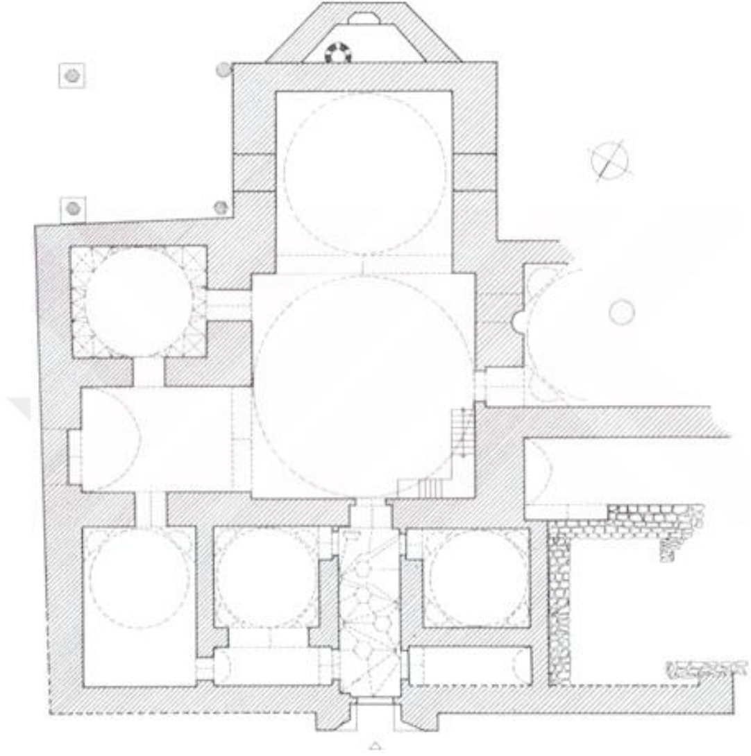
Çizim 3.16. Aksaray Melik Mahmut Gazi Hancahı planı (Parlak, 2004:246 )
