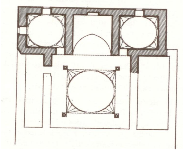
Çizim3.30. Konya Ali Gav Medresesi(Kuran1969:49)
