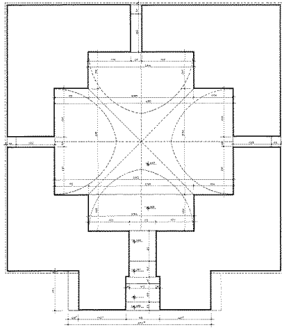
Kriptâ Planı
