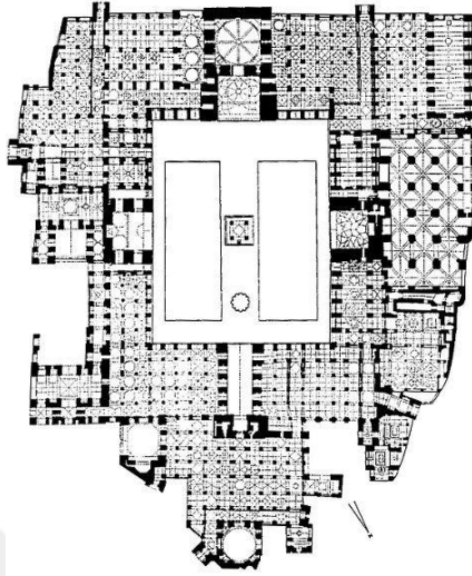
Çizim 3.35. İsfahan Ulu Cami planı
