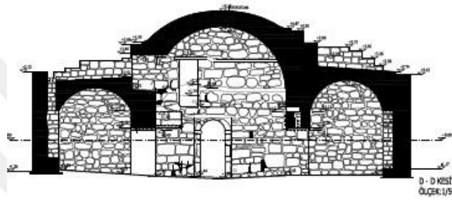
Çizim 3.2. Afyon Boyalıköy Hancahı Kuzey C-C ve D-D Kesiti (VGM arşivden)
