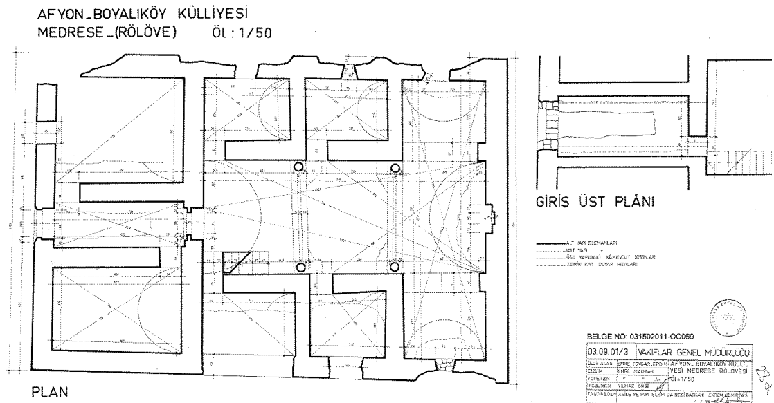
çizim 3.7. Boyalıköy Halkah Planı (VGM arşiv)
