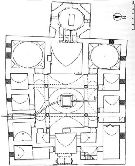
Çizim 3.32. Atabey Ertokuş Medresesi( Kuran 1969:48)
