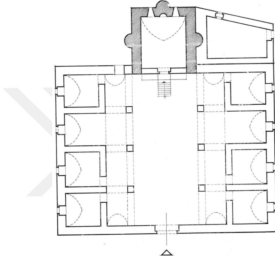
Çizim 3.43. Ümmühan Hatun Türbesi planı (Sözen, 1969:171)
