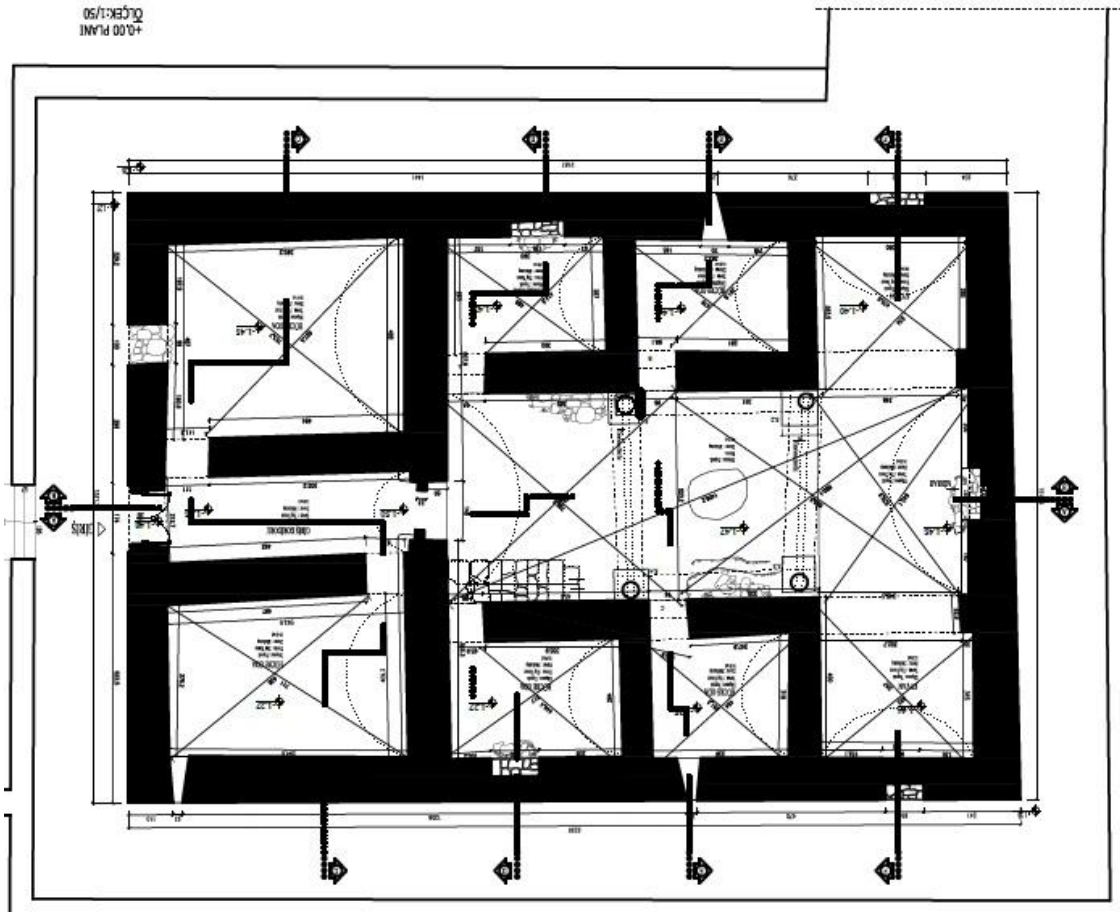
Çizim 3.6. Afyon Boyalıköy Halkah Planı (VGM arşivinden düzenlenerek)
