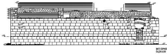
Çizim 3.5. Afyon Boyalıköy Hancahı doğu ve batı cephesi (VGM arşiv)
