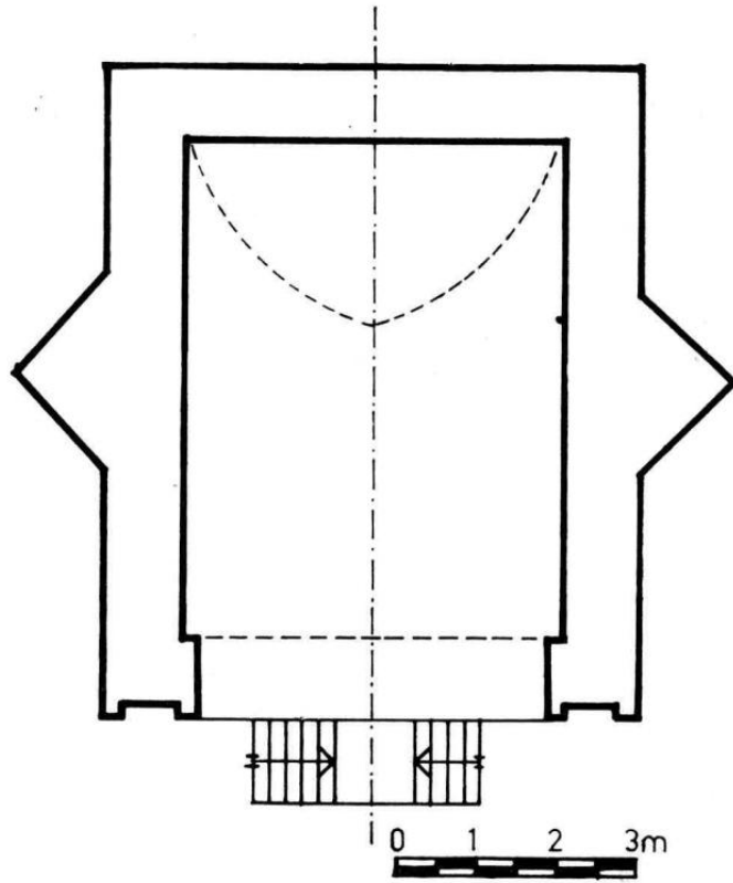
Çizim 3.45. Afyon - Herdena Saya Baba Türbesi Üst Kat Planı (Sözen, 1969:178)
