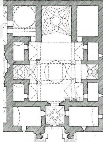
Çizim 3.33. Divriği Darüşşifası planı.
