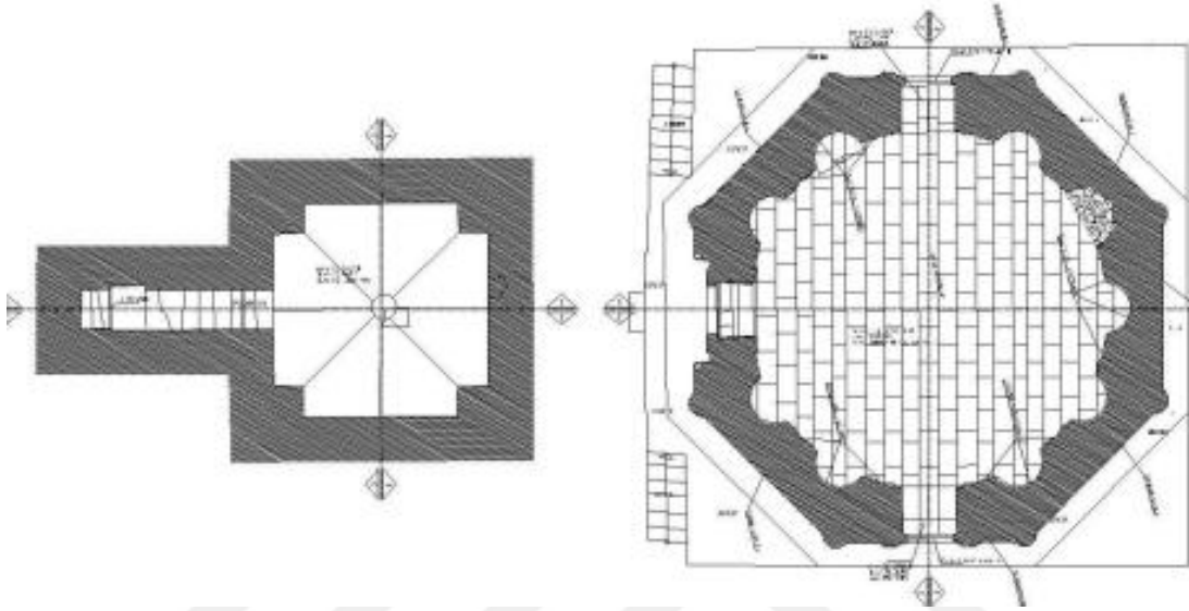
Çizim 3.53. İzzettin Keykavus Kümbet planı (Tanrıverdi, 2018: 103)
