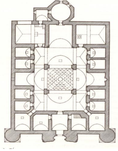
Çizim3.31. Yakutiye Medresesi(Kuran 1969:124)
