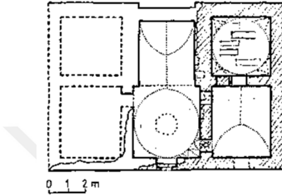
Çizim 3.21. Tokat Ebu Şemş Halkahı Planı
