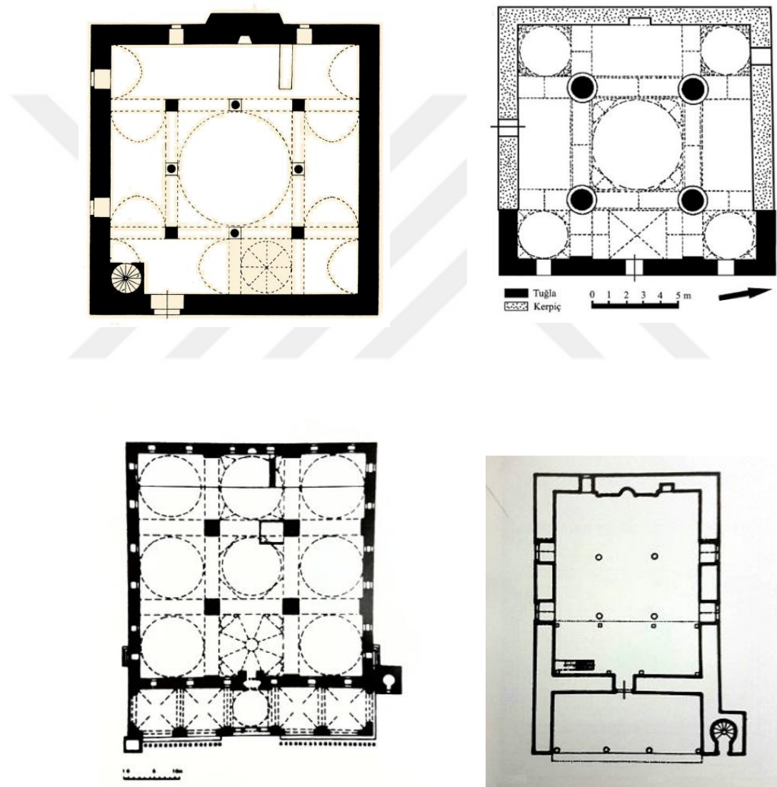
Çizim 3.34. kare içinde dört ayak uygulaması görülen bir grup cami planı
