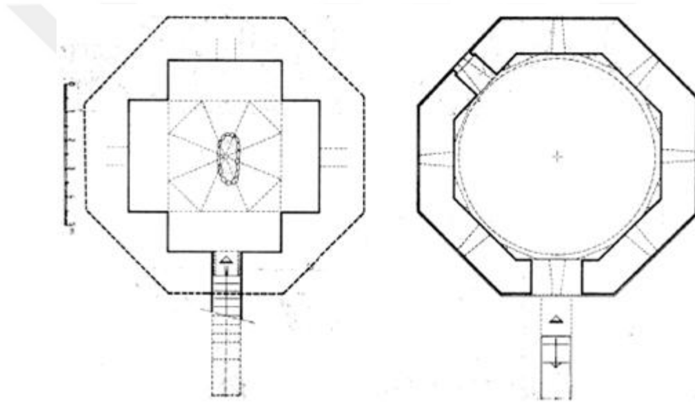
Çizim 3.48. Konya Kalender Baba Kümbeti Üst ve Alt Kat planları(Tuncer, 1986)
