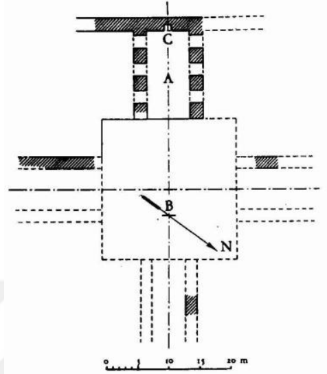
Çizim 3.29. Hargird Medresesi Planı
