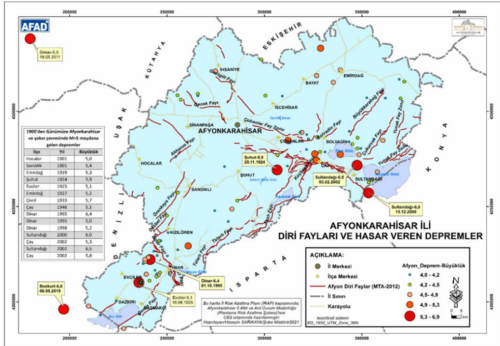
Şekil 2. 9 Afyonkarahisar İlinin Türkiye Diri Fay Haritasındaki Durumu [91].
