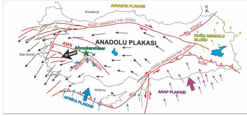
Şekil 2. 8 Türkiye'nin Neotektonik Yapılarını Gösteren Harita [91].
