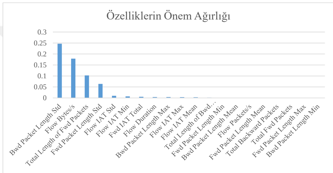
Şekil 3.4. CIC-IDS-2017 için seçilen özellikler ve onların önemi
