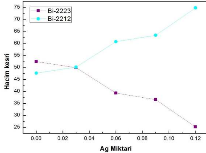
Şekil 8.6 Bi-(2223) ve Bi-(2212) fazlarının hacim kesirleri.
