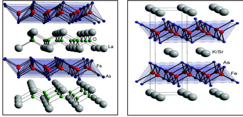
(a) (b) Şekil 3.9 (a) LaOFeAs ve (b) K/sr Fe 2 As 2 kristal yapıları.
