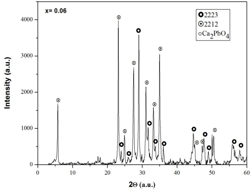
Şekil 8.3 \text{Bi}_{1.7}\text{Pb}_{0.3}\text{Sr}_2\text{Ca}_2\text{Cu}_{2.94}\text{Ag}_{0.06}\text{O}_y ( x=0.06 ) örneği için XRD deseni.
