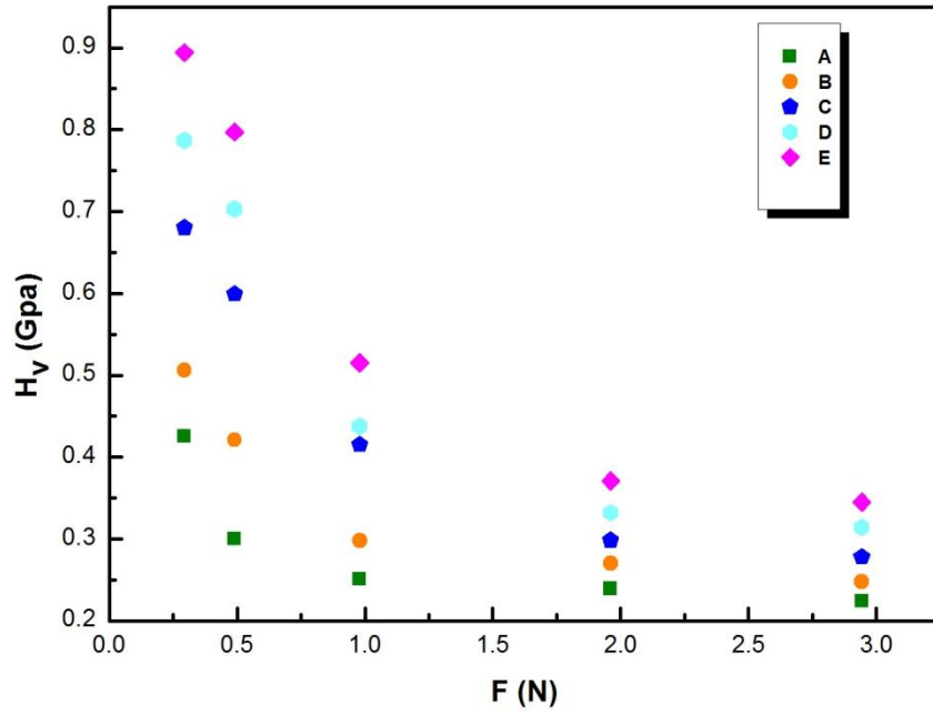
Şekil 8.17 A, B,C, D ve E örnekleri için yükle mikrosertliğin değişim grafiği.
