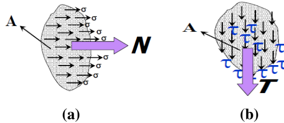
Şekil 4.1 (a) Normal gerilme ve (b) teğetsel gerilmenin şematik gösterimi.
