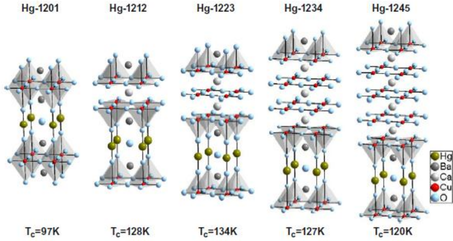
Şekil 3.7 \text{HgBa}_2\text{Ca}_{n-1}\text{Cu}_n\text{O}_{2n+3} sisteminin farklı fazları için kristal yapısı.
