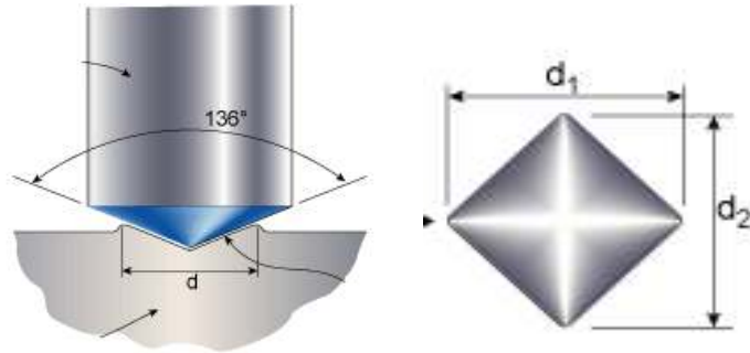
Şekil 5.2 Vickers girinti ucu ve iz şekli.
