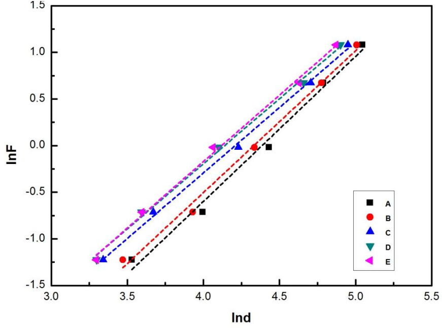
Şekil 8.18 Tüm örnekler için uygulanan yükün (lnF) köşegen (lnD) ile değişimi.
