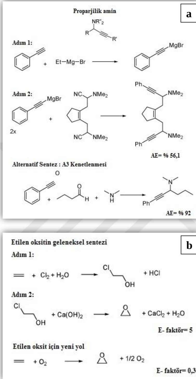
Şekil 2.9. a) Atom ekonomisi (AE) açısından proparjilik amin reaksiyonları b) E-faktör değişimi açısından etilen oksitin geleneksel yolla ve moleküler oksijen üzerinden sentezi (Anastas ve Eghbali 2010)
