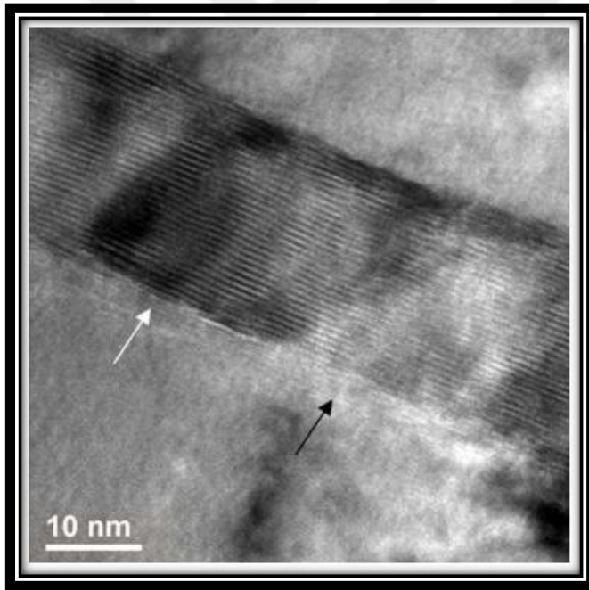
Şekil 2.2. \text{Fe}_3\text{C} nanopartiküllerinin paralel dizilişini gösteren HRTEM görüntüsü, oklar yerleşim kusurlarına işaret etmektedir (Reibold vd. 2009)
