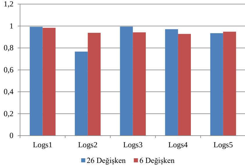
Şekil 5.3. Veri setlerinin 6 ve 26 değişkenli durumlarının precision sonuçları.
