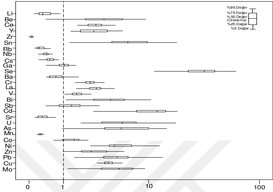
Şekil 22. Ağaçbaşı Yayla Turbalığı'ndaki iz elementlerin toprağa göre zenginleşmesi
