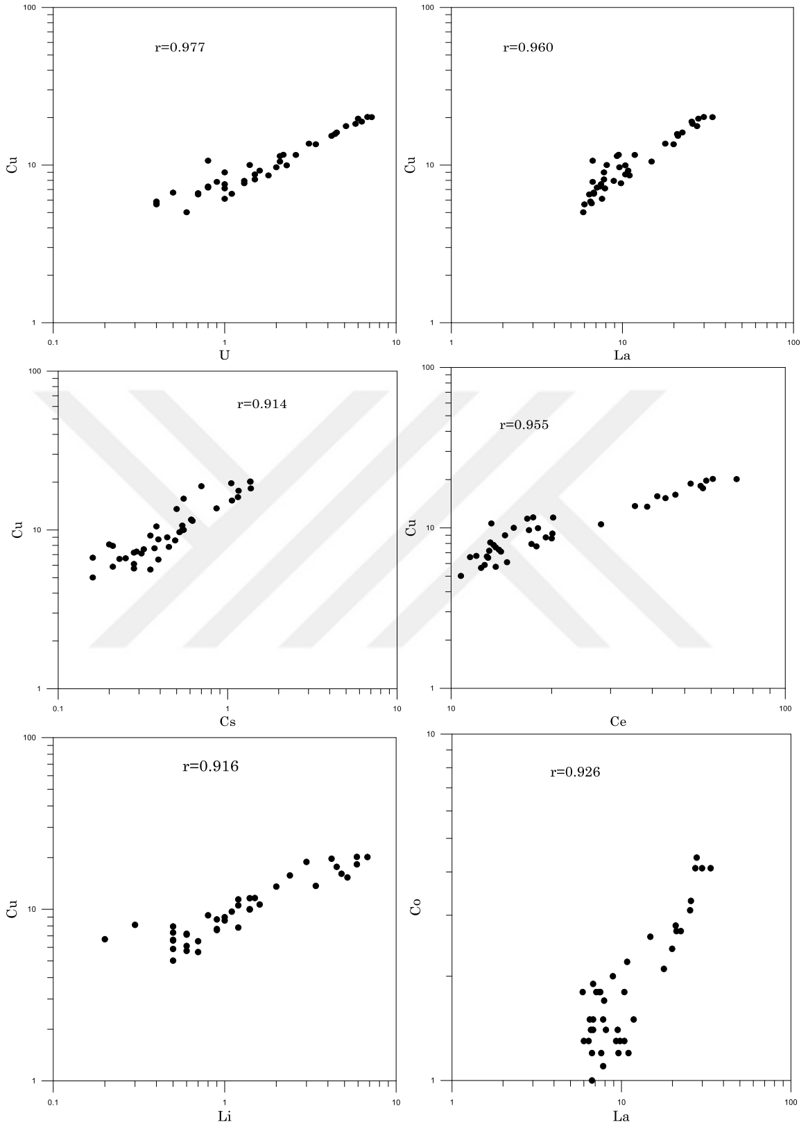
Şekil 17. Ağaçbaşı Yayla Turbalığı'ndaki iz elementler arasındaki ilişki (Cu, U, La, Cs, Ce, Li, Co)
