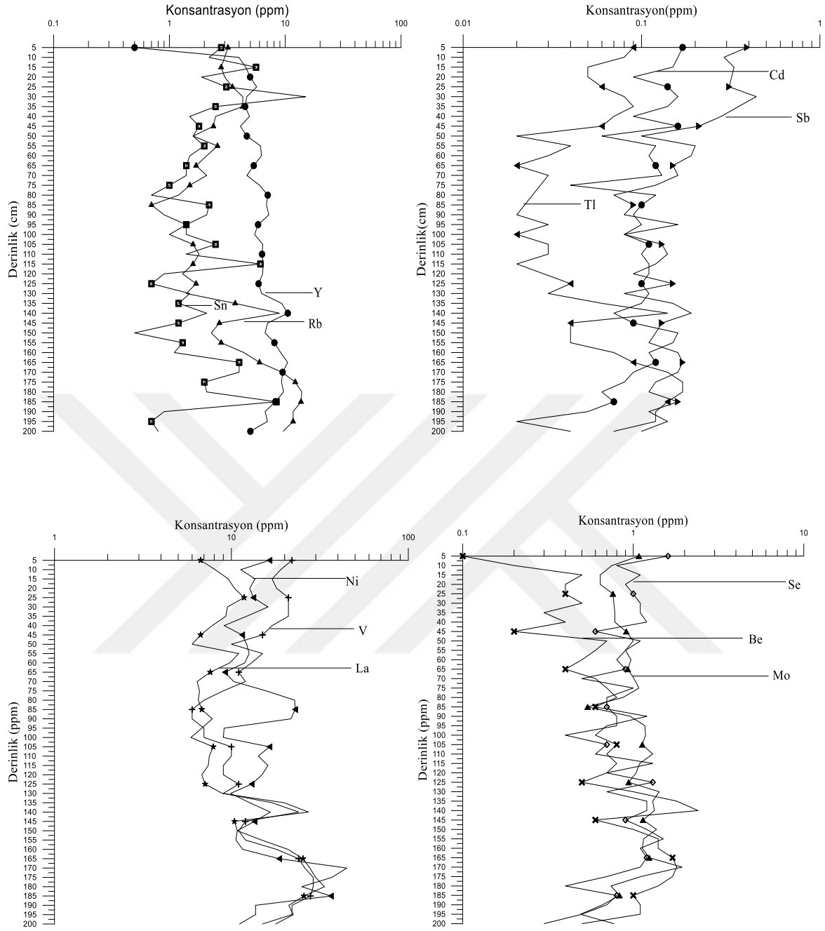
Şekil 15. Ağaçbaşı Yayla Turbalığı'ndaki iz element konsantrasyonu (Sn, Y, Rb, Cd, Sb, Tl, Ni, V, La, Se, Be, Mo)
