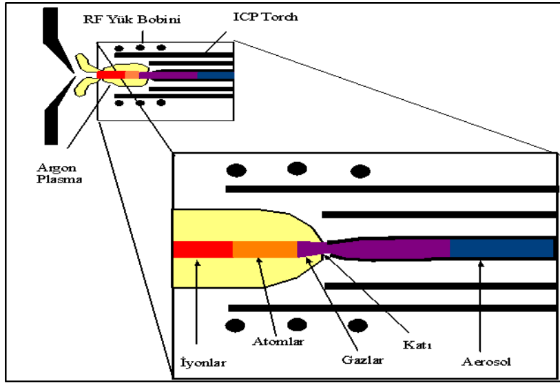
Şekil 6. Örneklerin ICP-MS Torch'ndaki durumunu gösteren kesit
