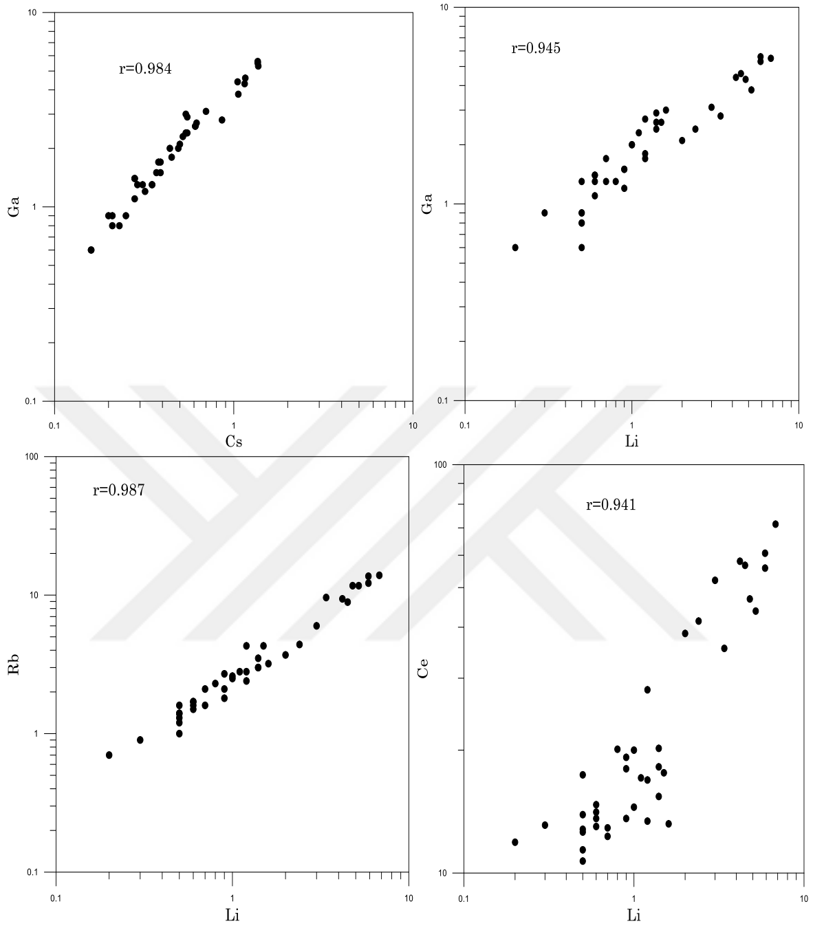
Şekil 20. Ağaçbaşı Yayla Turbalığı'ndaki iz elementler arasındaki ilişki ( Cs, Ga, Li, Rb, Ce)
