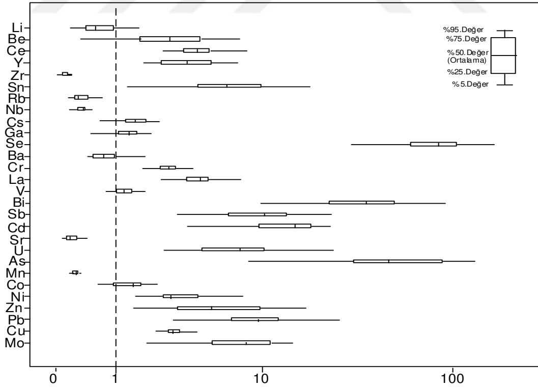
Şekil 23. Ağaçbaşı Yayla Turbalığı'ndaki iz elementlerin yerkabuğuna göre zenginleşmesi
