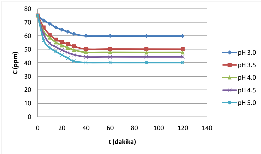
Şekil 5.3. Farklı pH değeriinde Cu(II) biyosorpsiyonu için zamana bağılı olarak derişim değışimleri ( T = 30\text{ }^{\circ}\text{C} ; C_0 = 75\text{ ppm} ; C_b = 3\text{ g/L} ; Karıştırma hızı = 140\text{ rpm} )
