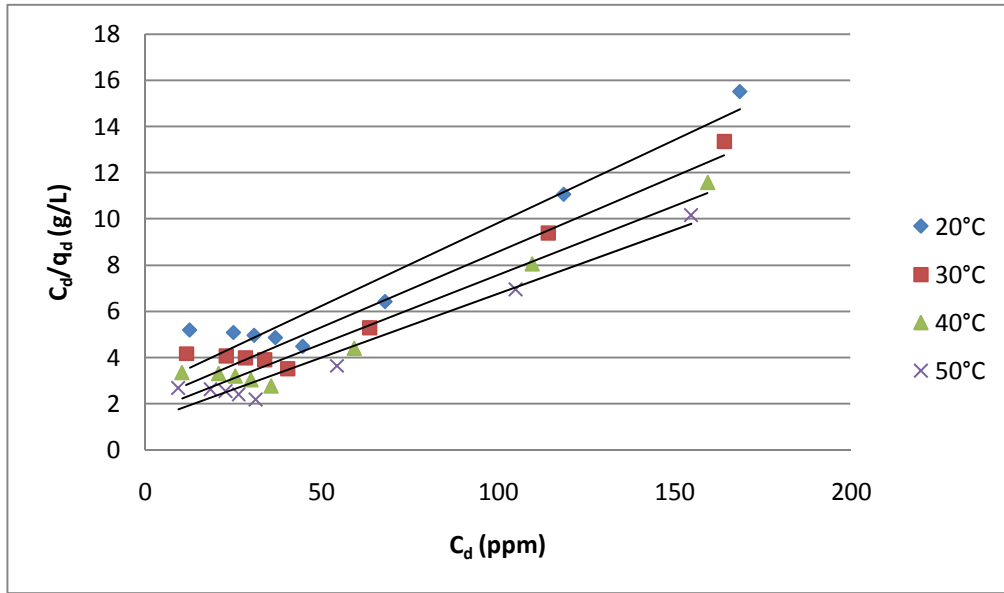
Şekil 5.12. Cu(II) iyonu için farklı sıcaklıklardaki (20, 30, 40 ve 50 °C) Langmuir izotermi
