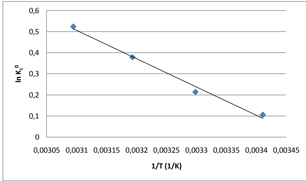
Şekil 5.33. Cr(VI) iyonu için denge sabitleri kullanılarak çizilen biyosorpsiyon ısısı grafiği
