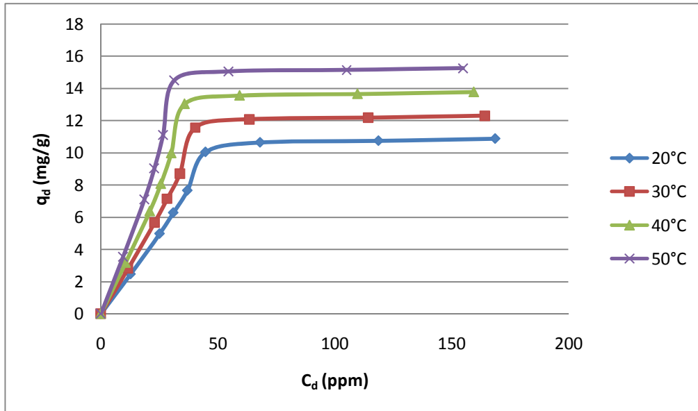
Şekil 5.11. Cu(II) iyonu için farklı sıcaklıklardaki (20, 30, 40 ve 50 °C) adsorpsiyon izotermi
