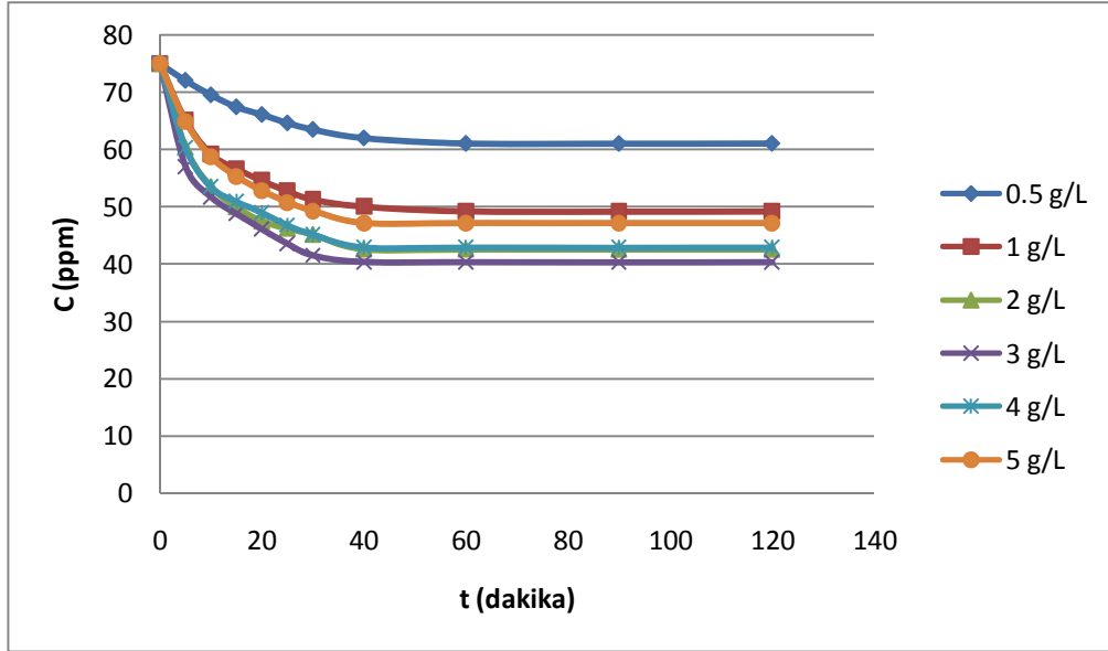
Şekil 5.9. 30 °C’de farklı biyokütle derişimi değerlerinde Cu(II) biyosorpsiyonu için zamana bağı olarak derişim değışimleri (pH = 5,0; T = 30 °C; C_0 = 75 ppm; Karıştırma hızı = 140 rpm)
