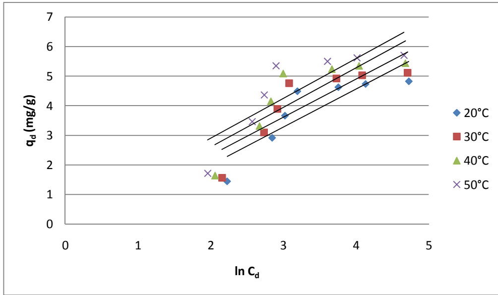
Şekil 5.31. Cr(VI) iyonu için farklı sıcaklıklardaki (20, 30, 40 ve 50 °C) Temkin izotermeleri
