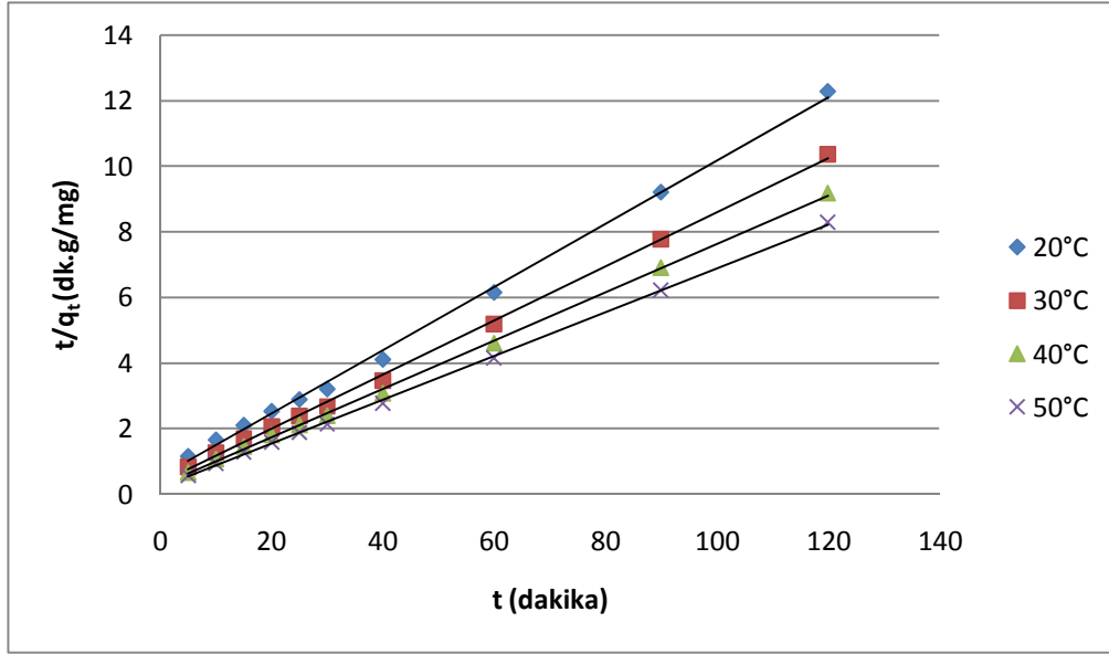
Şekil 5.18. Cu(II) iyonu için farklı sıcaklık değerlerinde ikinci derecemi kinetik modeli
