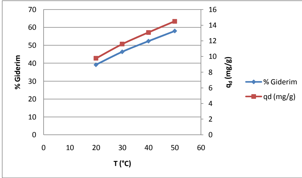
Şekil 5.6. Farklı sıcaklık değerlerinde Cu(II) biyosorpsiyonu için maya üzerine % giderim ve metal kazanım ( q_d ) değerleri
