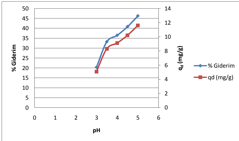
Şekil 5.4. Farklı pH değeriinde Cu(II) biyosorpsiyonu için maya üzerine % giderim ve metal kazanım ( q_d ) değeri
