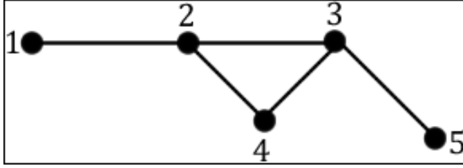
Şekil 4.7. G grafi
