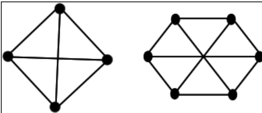
Şekil 2.9. 3-Regüler graf
