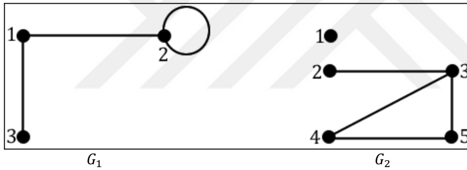
Şekil 2.1. Graf örnekleri
