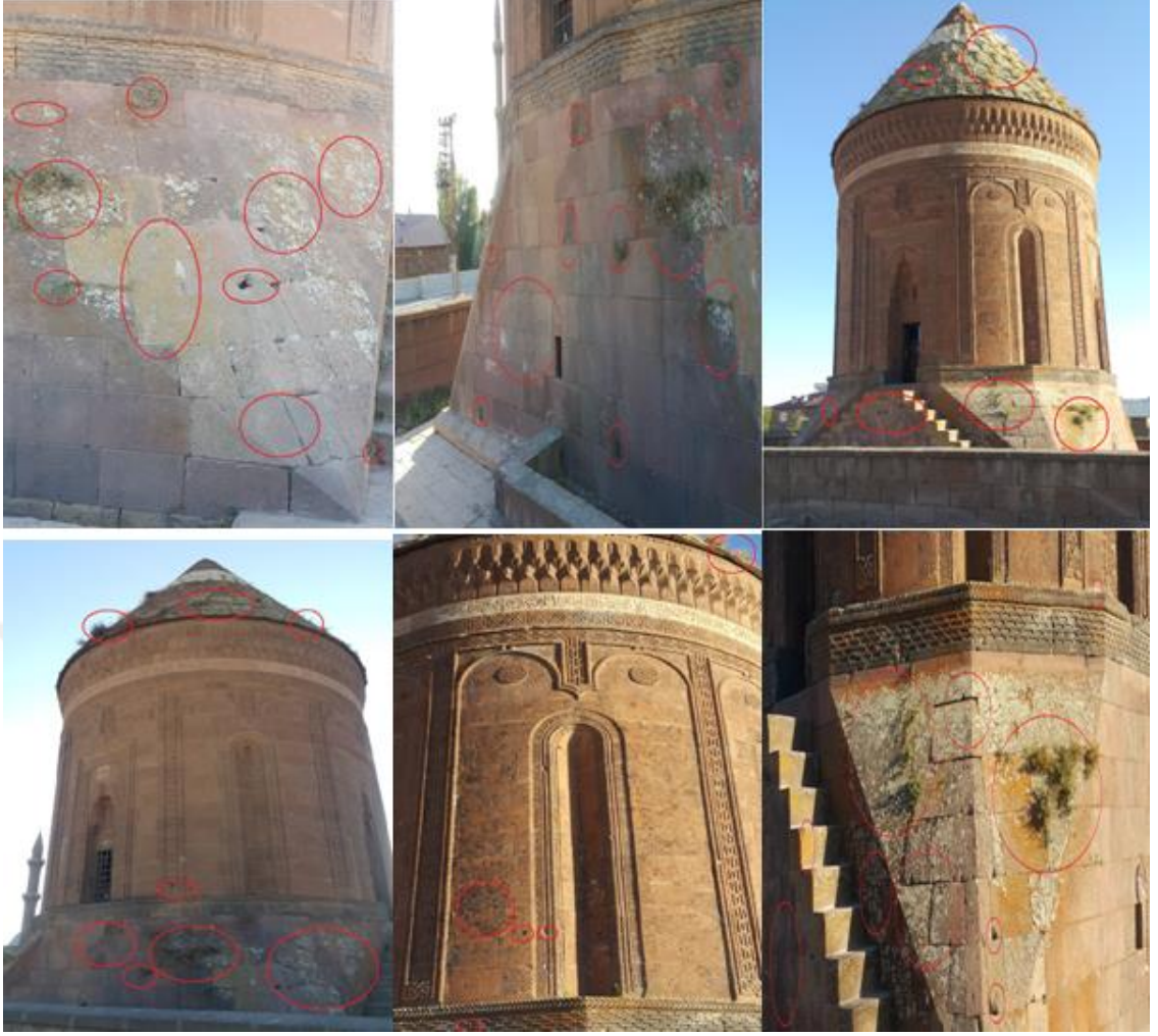
Şekil 4.14. Usta Şagird Kumbetinde gözlemlenen hasarlar
