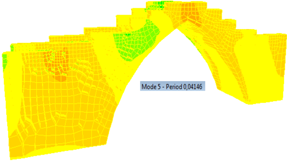
Şekil 4.64c. Köprü modeli için elde edilen 5. mod şekli ve periyot değeri
