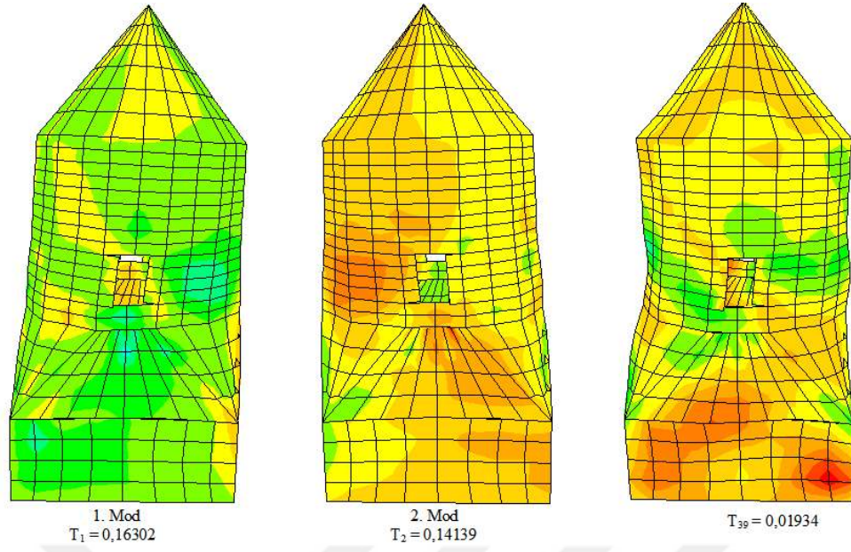
Şekil 4.50. Kümbet modeli için elde edilen mod şekilleri ve periyot değerleri
