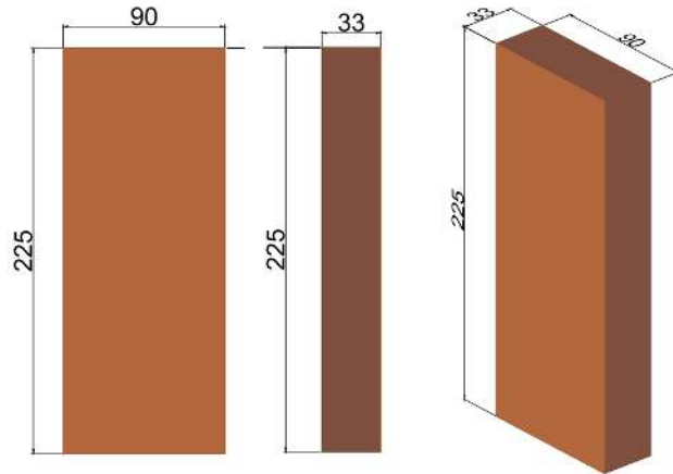
Şekil 4.34. İncelenen mezar taşına ait boyutlar
