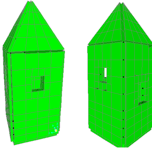
Şekil 4.70. Yazılım programında oluşturulan türbenin modeli
