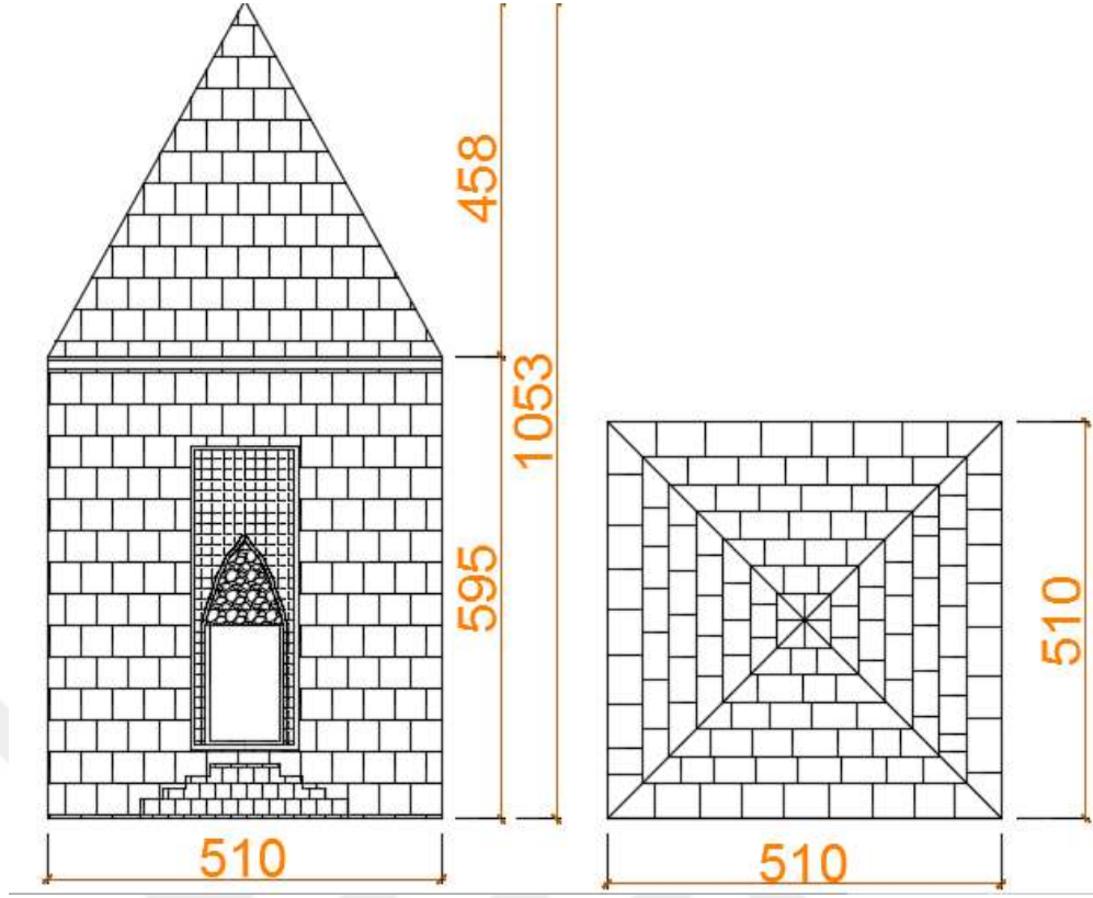
Şekil 4.69. İncelenen kümbete ait boyutlar
