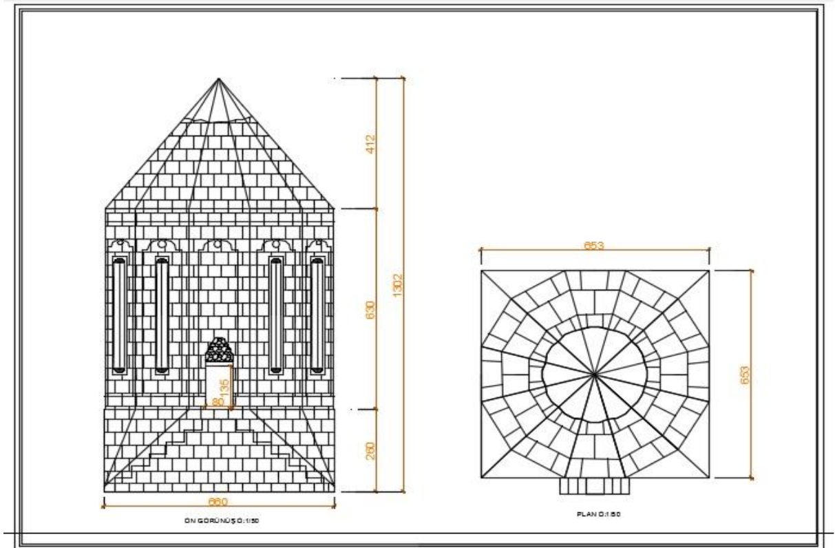
Şekil 4.48. İncelenen kümbete ait plan ve boyutlar
