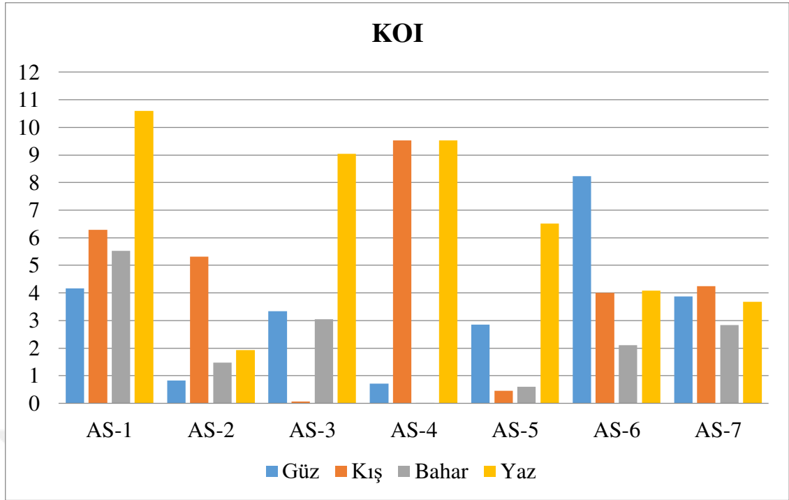
Şekil 4.47. Örneklem noktalarına göre KOİ' nin mevsimsel değişimi
