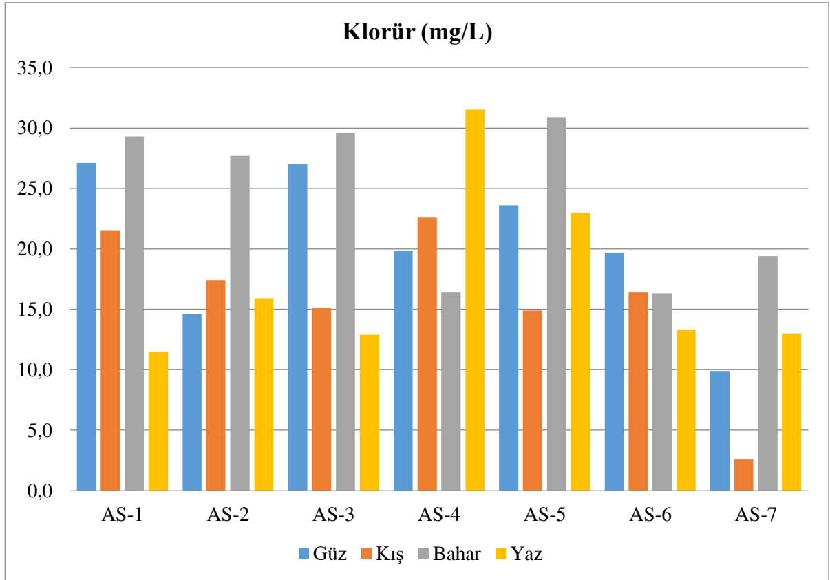
Şekil 4.17. Örneklem noktalarındaki Cl'nin mevsimsel değişimi
