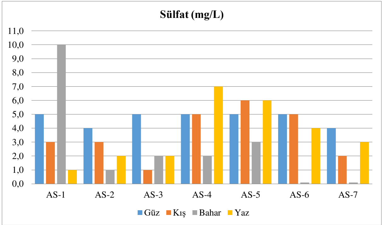
Şekil 4.15. Örneklem noktalarındaki \text{SO}_4^{-2} 'nin mevsimsel değişimi
