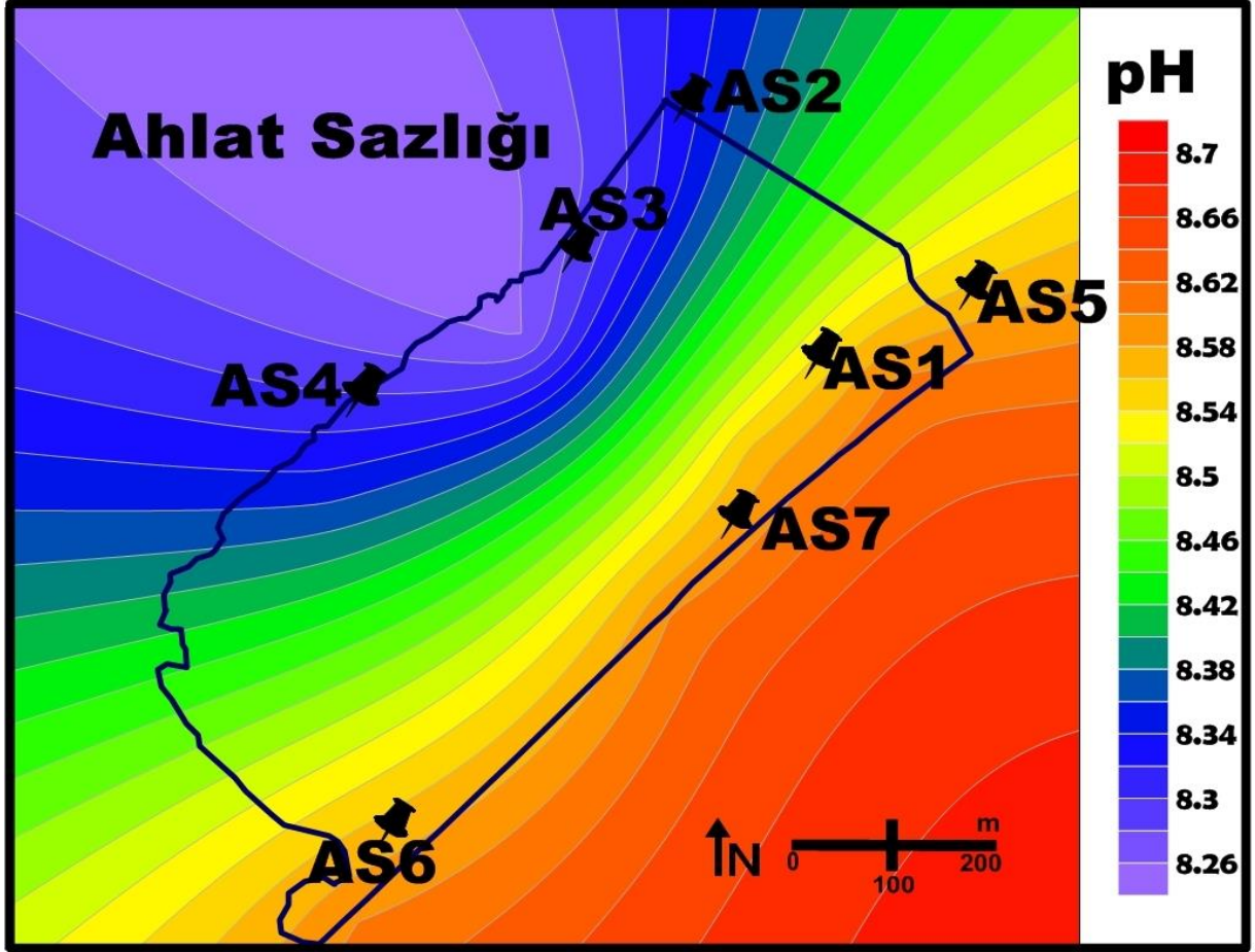
Şekil 4.6. pH'nın mevsimlik ortalamasına ait alansal dağılım haritası
