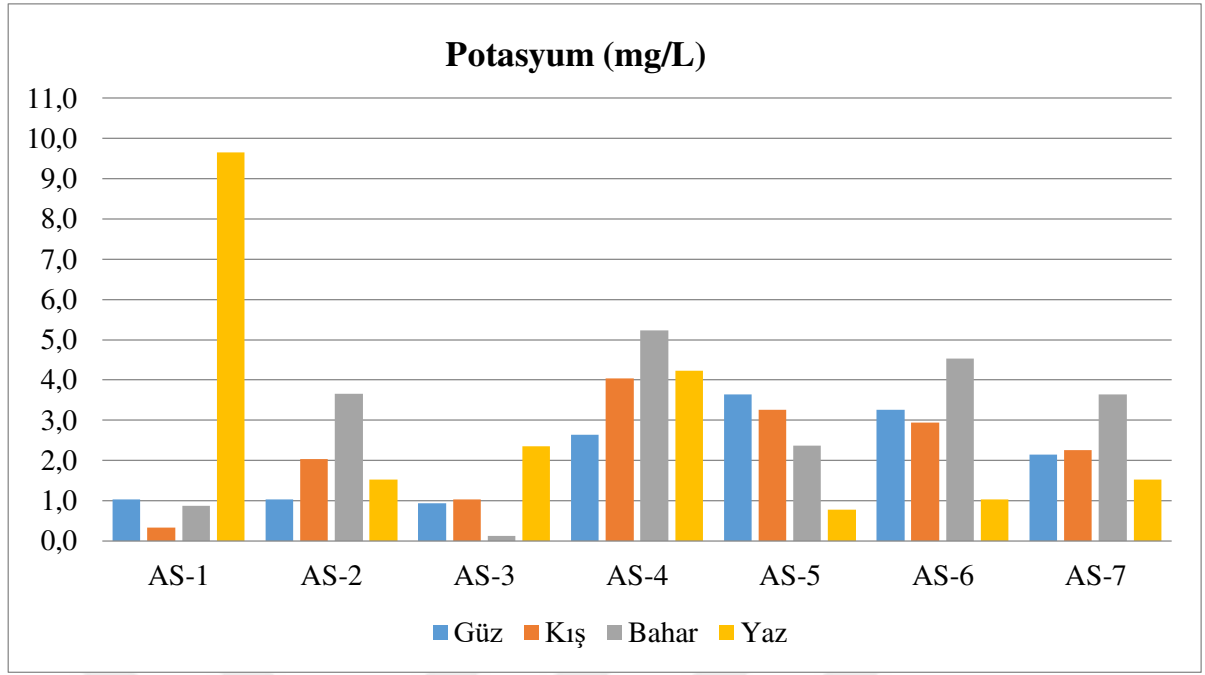
Şekil 4.27. Örneklem noktalarına göre K'nın mevsimsel değişimi
