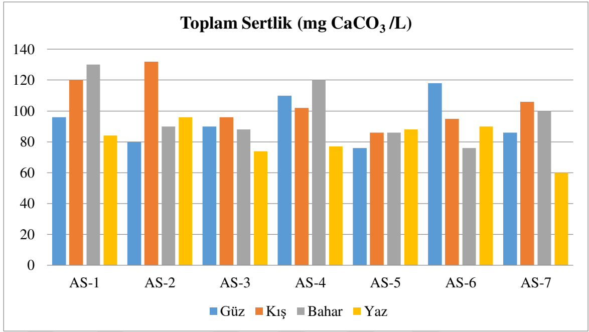
Şekil 4.29. Örneklem noktalarına göre Toplam sertliğin mevsimsel değişimi
