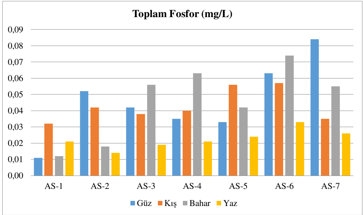
Şekil 4.43. Örneklem noktalarına göre TP' nin mevsimsel değişimi
