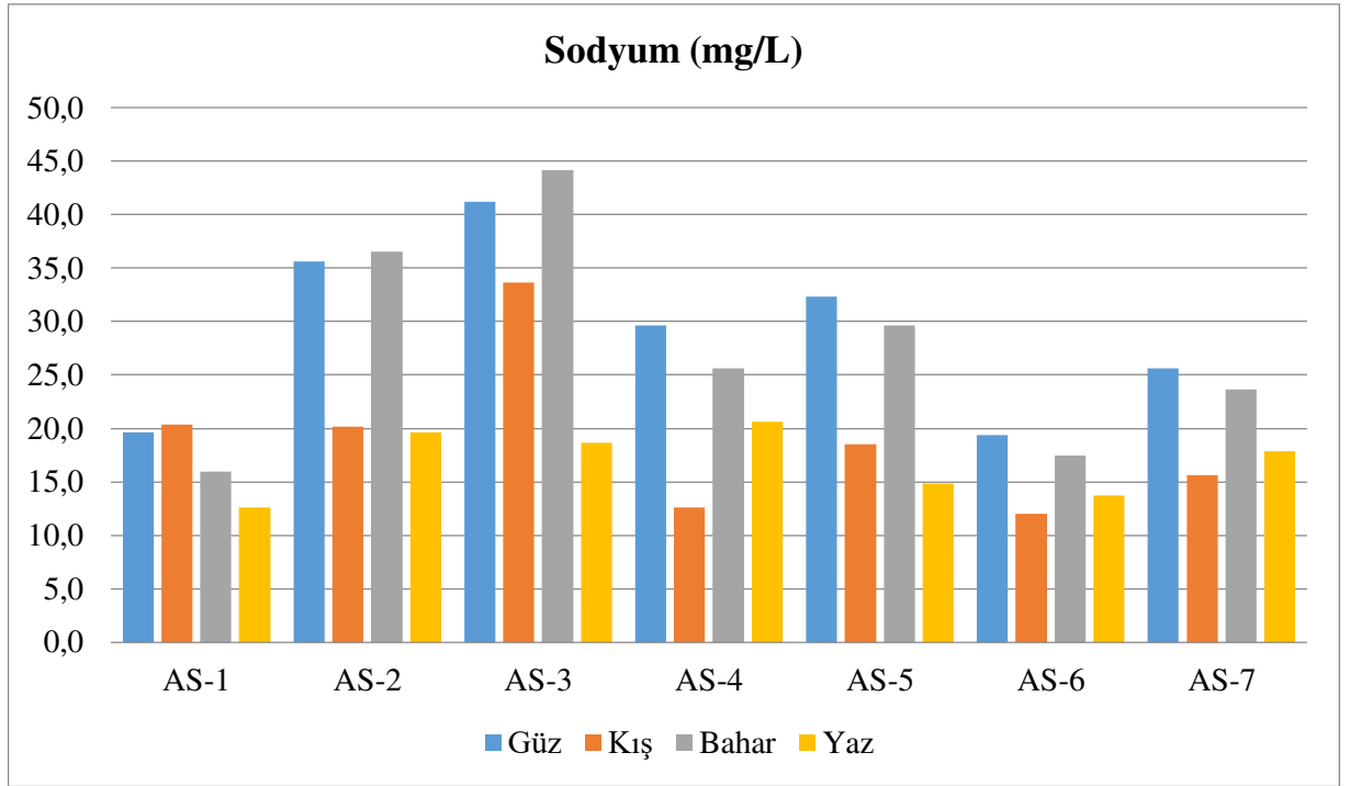
Şekil 4.25. Örneklem noktalarına göre Na'nın mevsimsel değişimi
