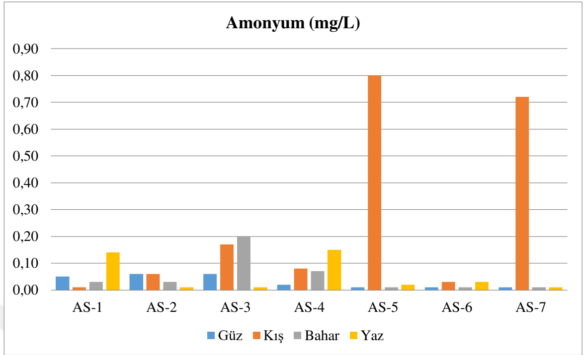
Şekil 4.35. Örneklem noktalarına göre \text{NH}_4 'ün mevsimsel değişimi
