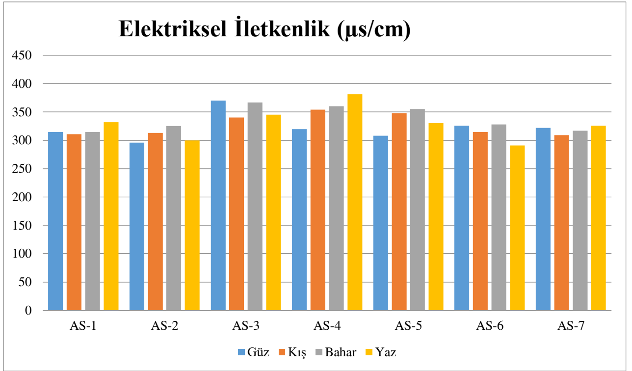
Şekil 4.9. Örneklem noktalarındaki elektriksel iletkenliğin mevsimsel değişimi
