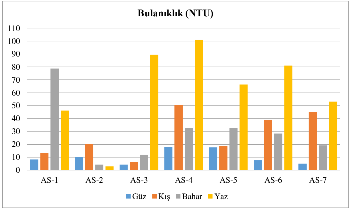
Şekil 4.31. Örneklem noktalarına göre bulanıklığın mevsimsel değişimi
