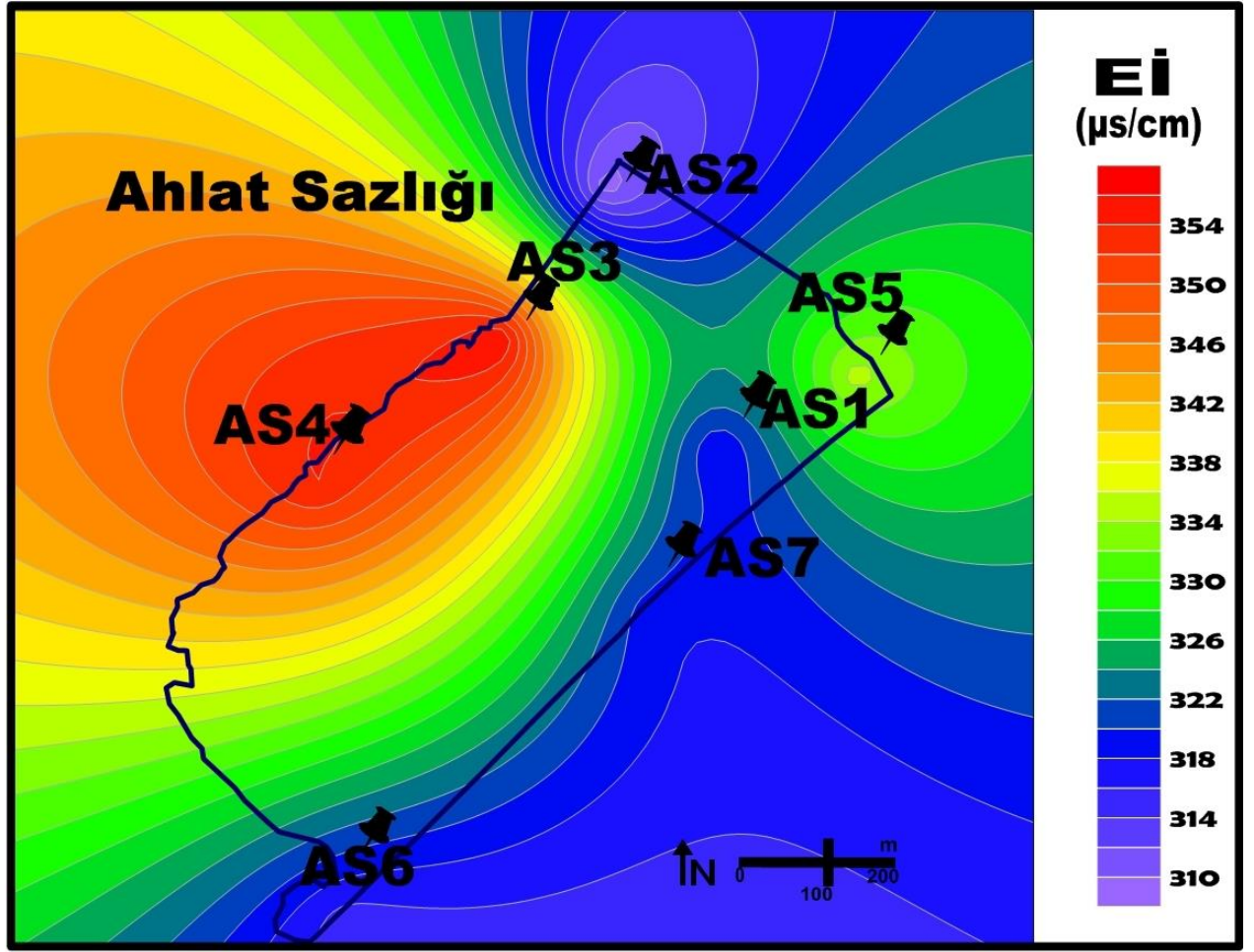
Şekil 4.10. Elektriksel iletkenliğin mevsimlik ortalamasına ait alansal dağılım haritası
