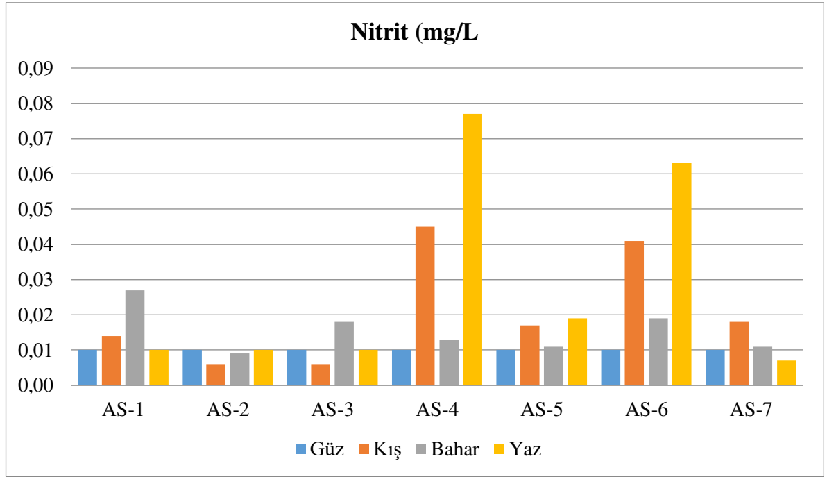
Şekil 4.37. Örneklem noktalarına göre \text{NO}_2^- mevsimsel değişimi
