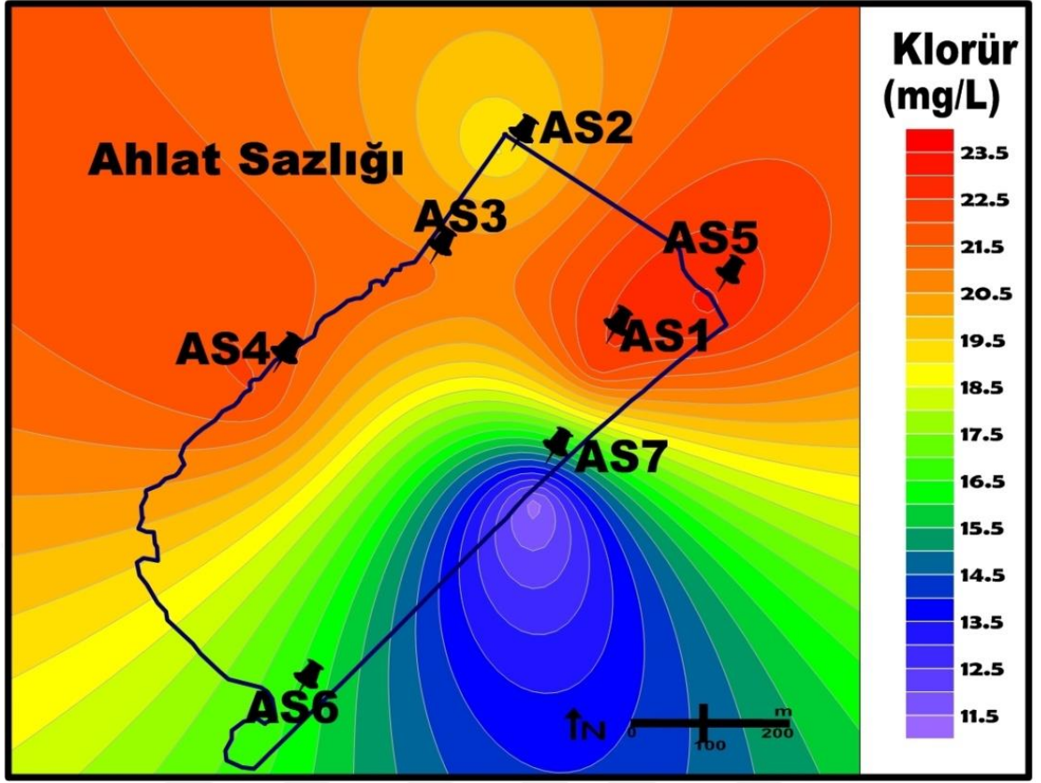
Şekil 4.18. Cl mevsimlik ortalamasına ait alansal dağılım haritası
