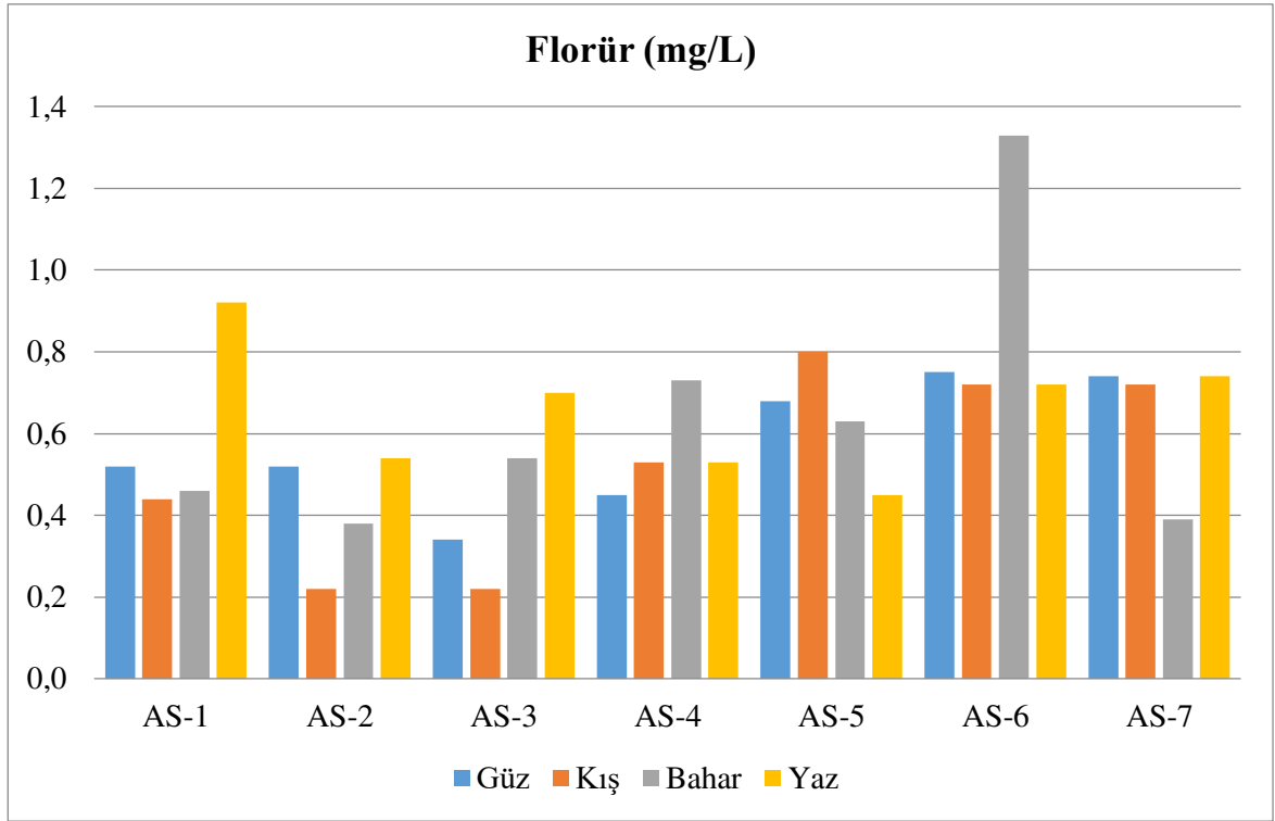
Şekil 4.19. Örneklem noktalarındaki F'nin mevsimsel değişimi
