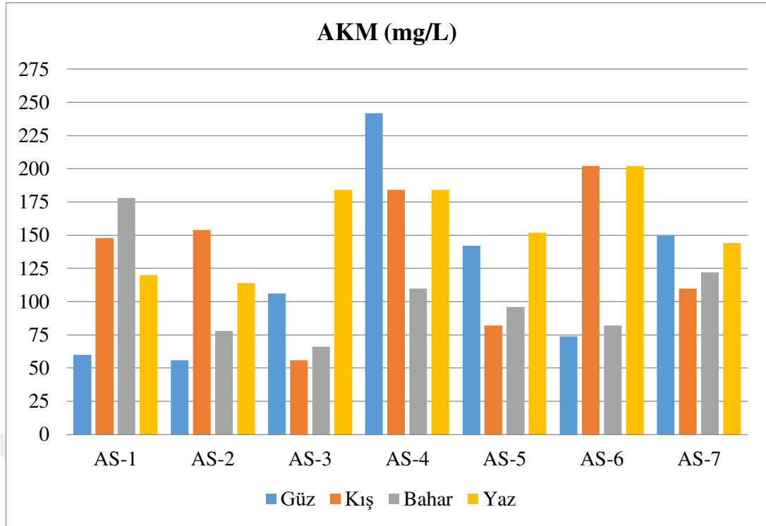
Şekil 4.33. Örneklem noktalarına göre AKM' nin mevsimsel değişimi
