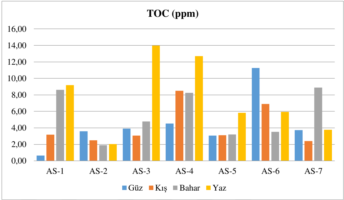
Şekil 4.45. Örneklem noktalarına göre TOC' un mevsimsel değişimi
