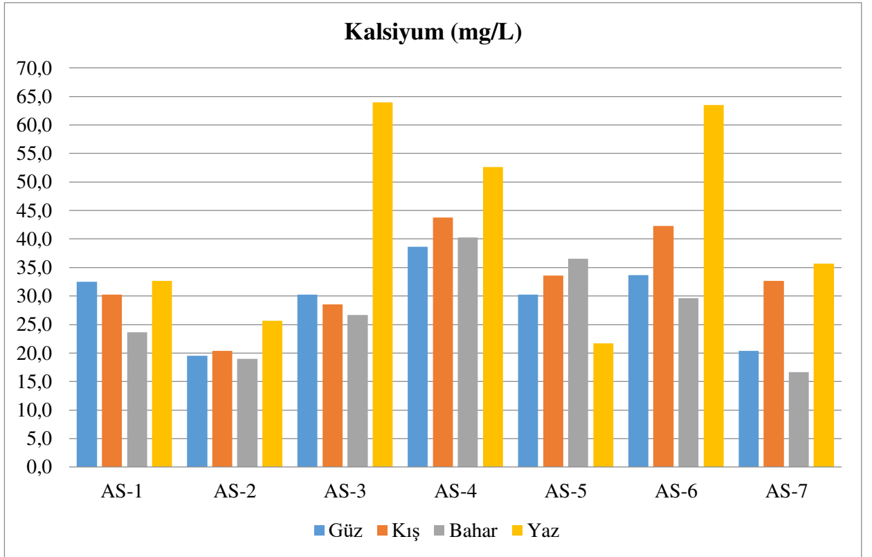
Şekil 4.21. Örneklem noktalarına Ca'nın mevsimsel değişimi
