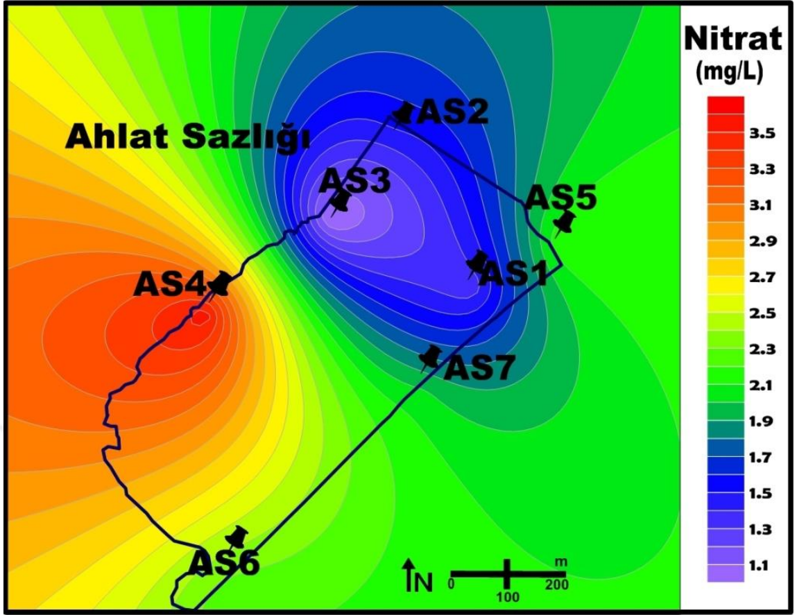
Şekil 4.40. Nitrat'ın mevsimlik ortalamasına ait alansal dağılım haritası
