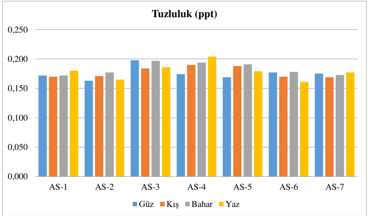
Şekil 4.11. Örneklem noktalarındaki tuzluluğun mevsimsel değişimi
