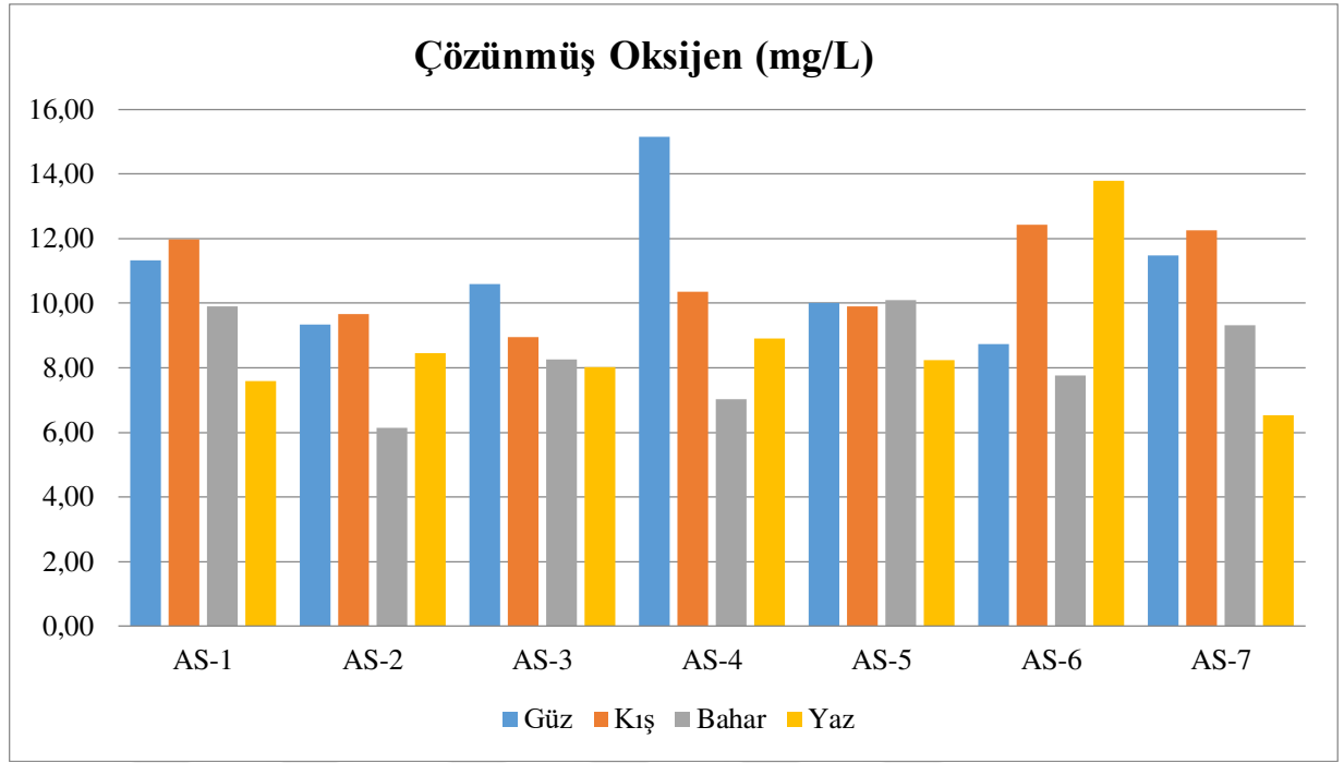
Şekil 4.3. Örneklem noktalarındaki çözünmüş oksijenin mevsimsel değişimi
