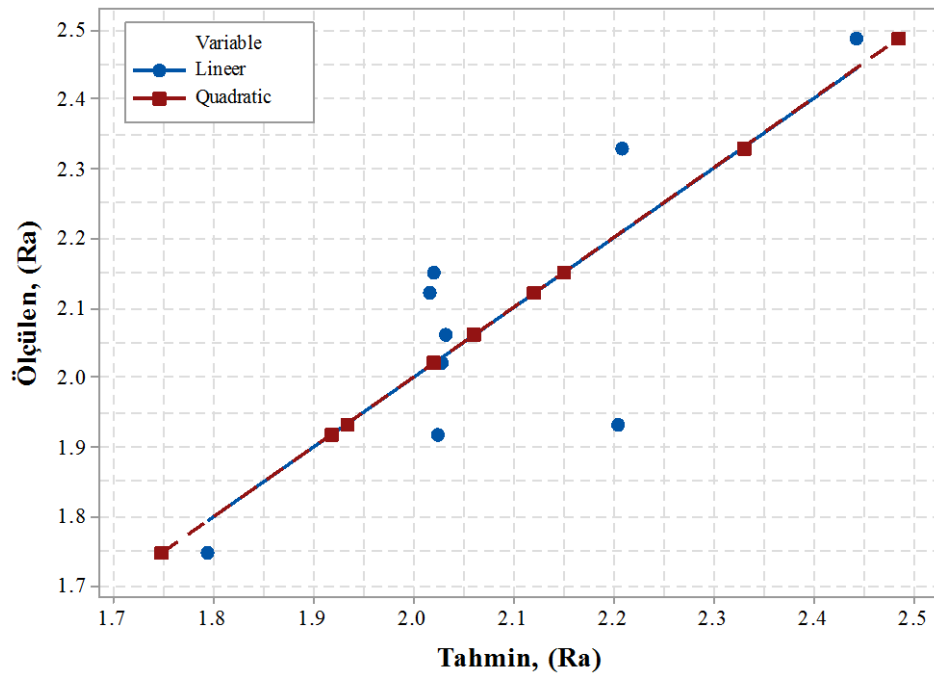
Şekil 8.3. Yüzey pürüzlülüğünün deney sonuçları ile tahmin değerlerinin karşılaştırılması.
