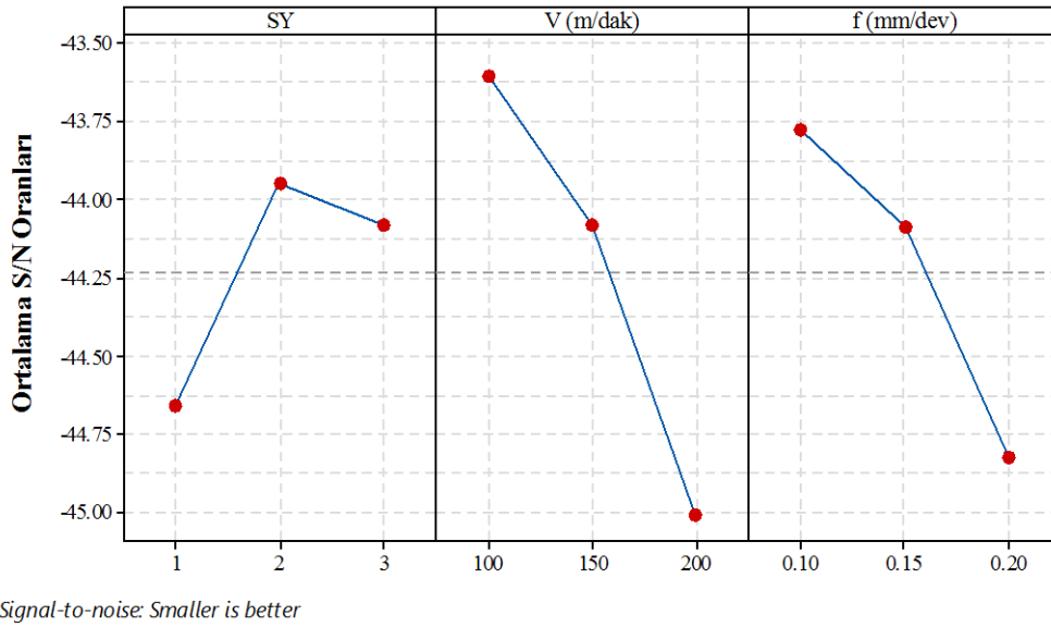
Şekil 8.10. L_{27} Kesme sıcaklığı için ortalama S/N oranları grafiği.
