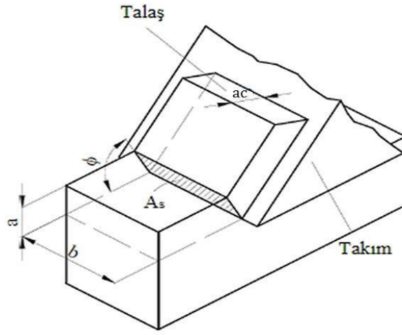
Şekil 3.7. Ortogonal kesmede kayma düzlemi [50].
