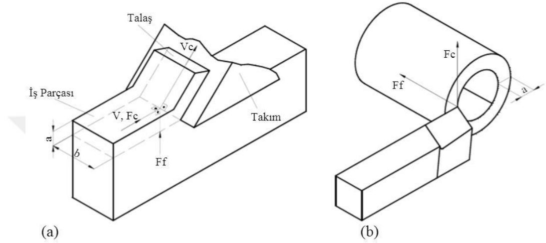
řekil 3.4. Ortogonal kesme geometrisi [(a) Dzlemsel, (b) silindirik [49].
