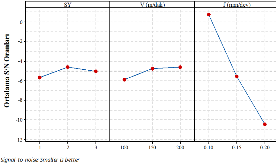
Şekil 8.9. L_{27} Yüzey pürüzlülüğü için ortalama S/N oranları grafiği.
