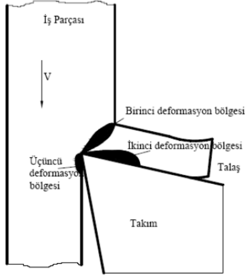
Şekil 3.5. Ortogonal kesmede oluşan deformasyon bölgeleri [50].
