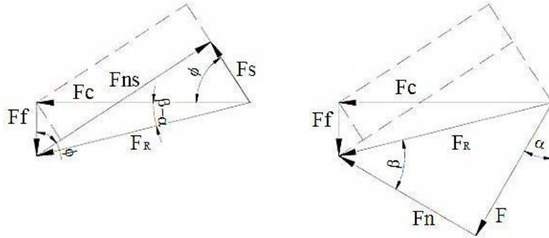
Şekil 3.6. Ortogonal kesme mekaniği [50].
