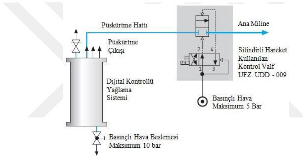
Şekil 4.4. SKF firması tarafından üretilen MMY sistemine ait pnömatik şema [93]. MMY sisteminin olumlu yönleri aşağıdaki şekilde sıralanabilir;
