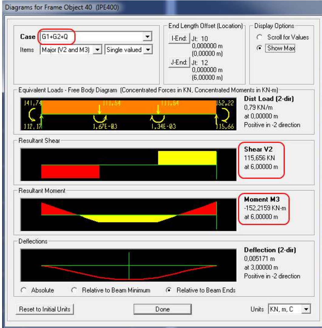
Şekil 5.5: Düşey yüklemeden hesaplanan iç kuvvetler
