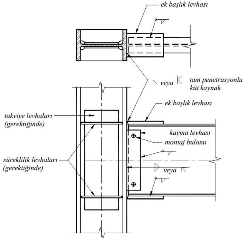
Şekil 4.5 : Ek başlık levhali kaynaklı birleşim detayı
