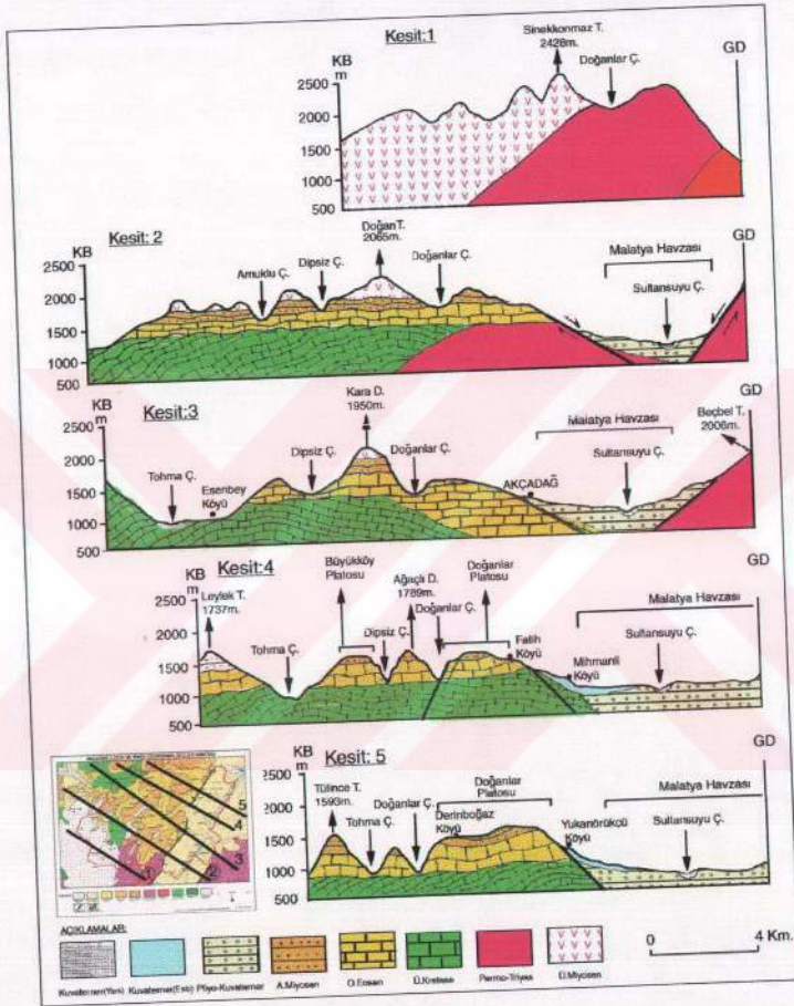
Şekil:2 İnceleme Alanında KB-GD Doğrultusunda Alınmış Jeolojik Kesitler
