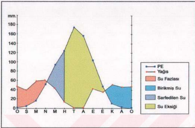
Grafik 10: Akçadağ'ın Su Balançosu Diyagramı
