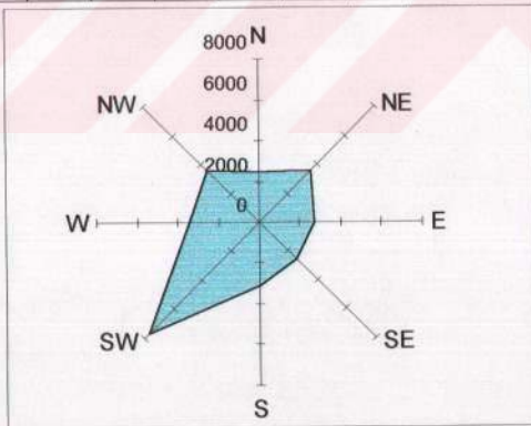
Grafik 5: İnceleme Alanının Yıllık Ortalamalara Göre Hakim Rüzgar Gülü Diyagramı (1929 - 1990)
