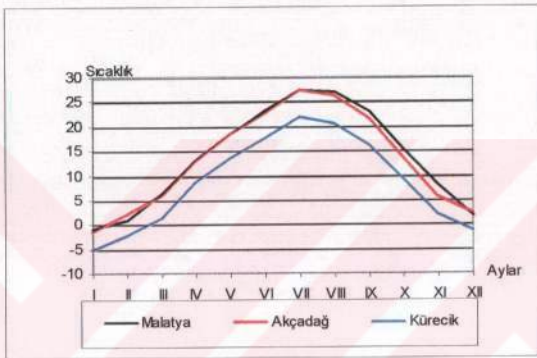
Grafik 1: Malatya, Akçadağ ve Küreçik'te Aylık Ortalama Sıcaklıkların Yıl İçindeki Seyrini Gösterir Grafik
