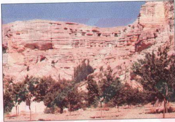
Foto 2: Denizel Miyosen Tortulları – Yataya Yakın Özellik Gösteren Miyosen Tortulları Üzerindeki Şekiller(Küçükkürne köyünden).
