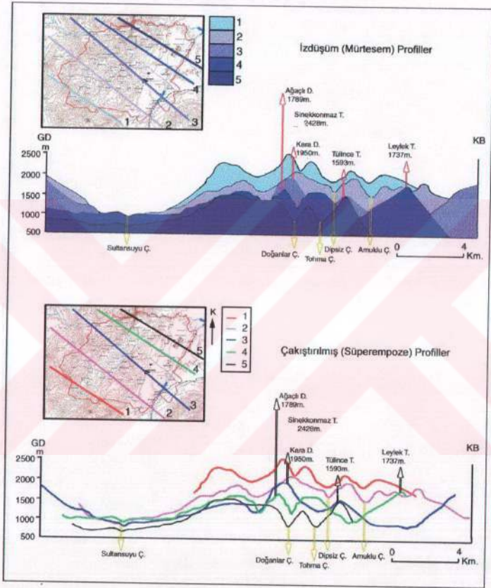
Şekil 4: İnceleme Alanında KB-GD Doğrultusunda Alınmış Topografik Profil Serileri
