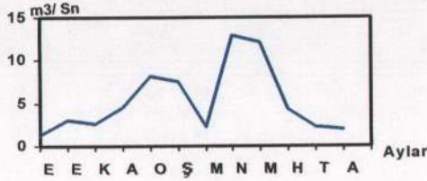
Grafik 12: Hara akım istasyonunda müteferrik (ayların belirli günlerinde yapılan ölçüm) rasatlara göre Sultansuyu'nun ortalama akım gidişi
