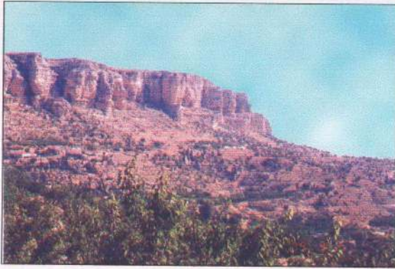
Foto 14: Farklı Dirençteki Kayaçların Farklı Aşınmalarıyla Meydana Gelen Kornişli Yamaçlar. Şekilde Eosen Kalkerlerinin Dik Bir Korniş Oluşturduğu Görülmektedir. (Sarıhacı Ve Yalınkaya Koylerine Doğru)
