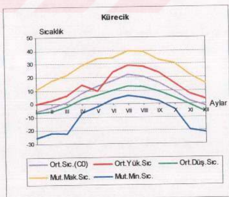
Grafik 3: Malatya'da Aylık ve Ortalama Ekstrem Sıcaklıklar
