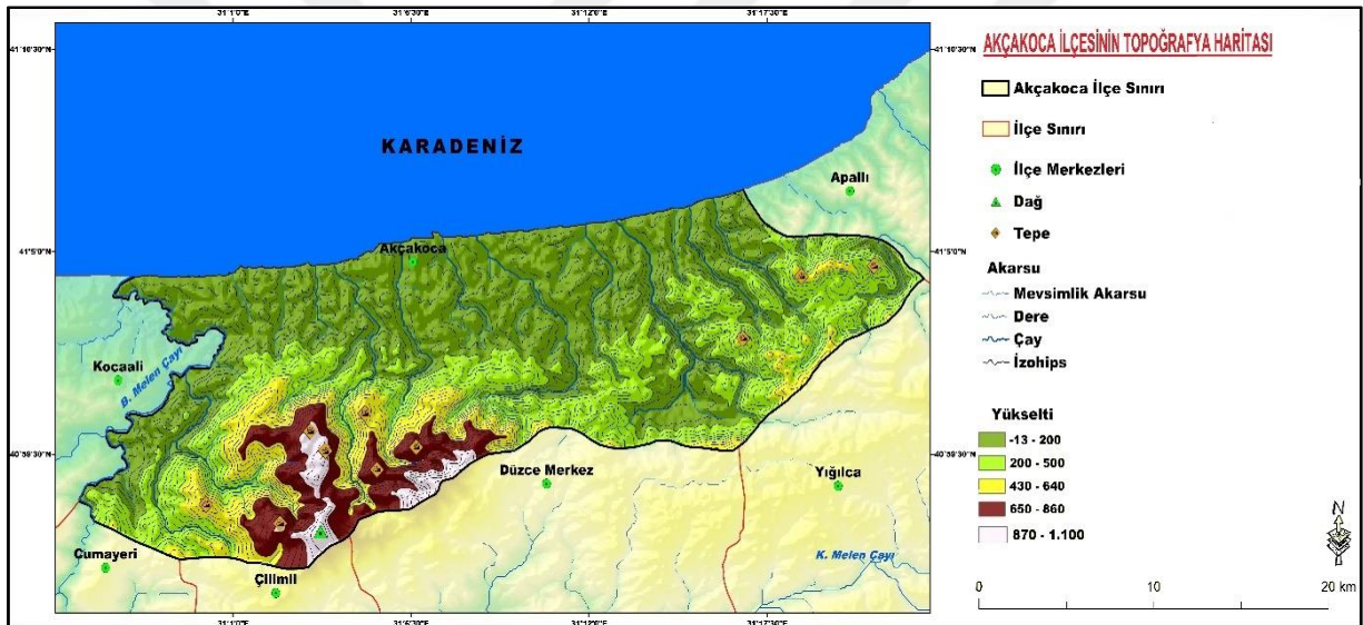
Harita 4.1. Akçakoca İlçesinin Topografya Haritası
