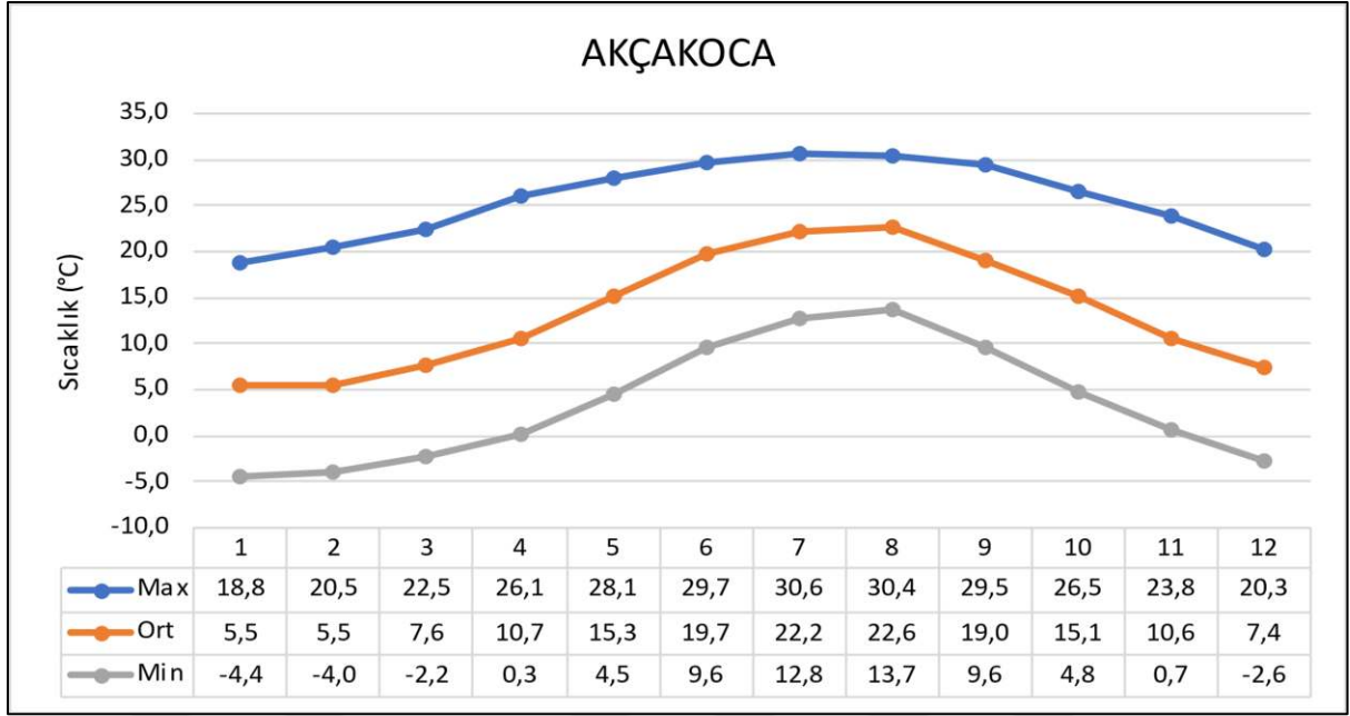
Grafik 3.2. Akçakoca 1980-2020 Yılları Ortalama Maximum, Orta, Minimum Sıcaklık Değerleri
