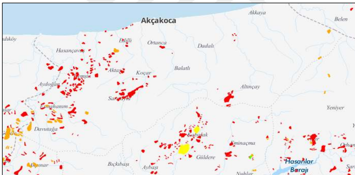
Harita 4.2. Akçakoca İlçesi Heyelan Haritası
