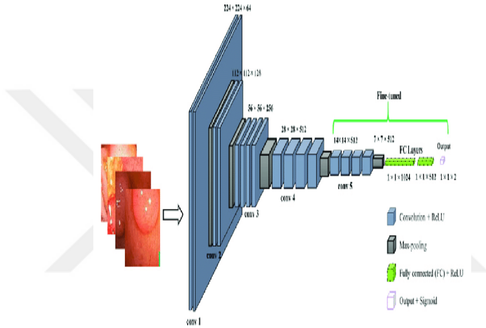
Şekil 3.5. VGG19 mimarisi (Hasan ve ark., 2022).
