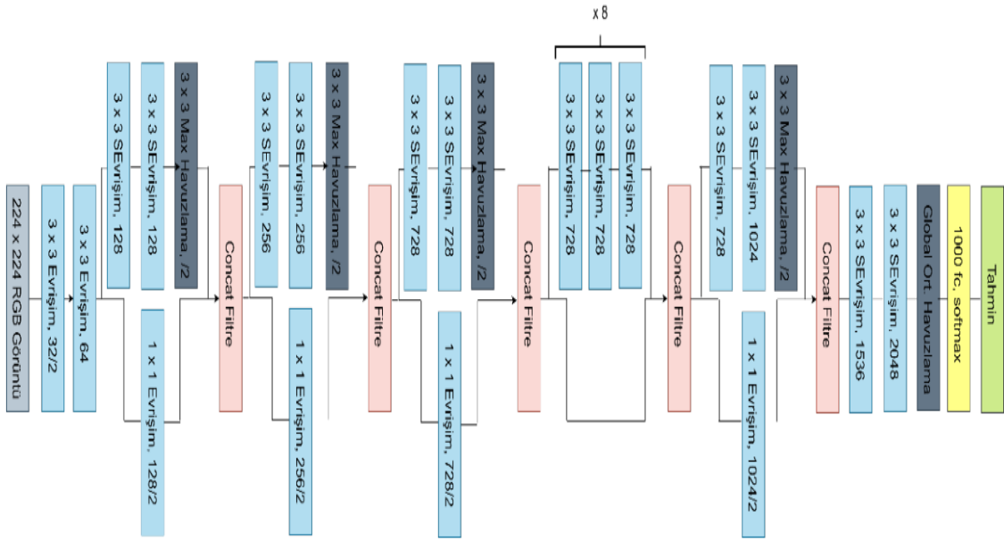
Şekil 3.6. Xception ağ mimarisi (Şener, A., & Ergen, 2022).
