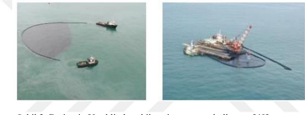
Şekil 2. Bariyerin U şeklinde çekilmesi ve sıyrıcı kullanımı [40]
