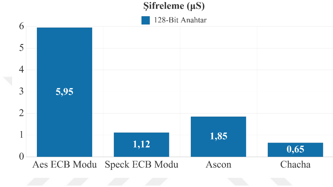
Şekil 3.25. 128 Bit Anahtar Şifreleme
