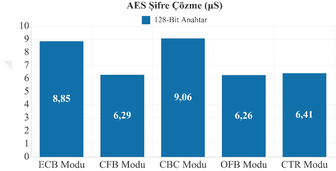
Şekil 3.10. Aes 128 Bit Anahtar Şifre Çözme
