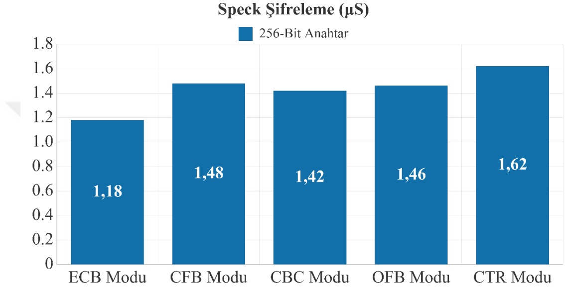
Şekil 3.19. Speck 256 Bit Anahtar Şifreleme
