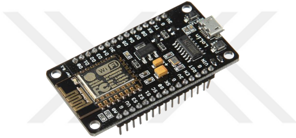
Şekil 3.2. NodeMCU Cihazı
