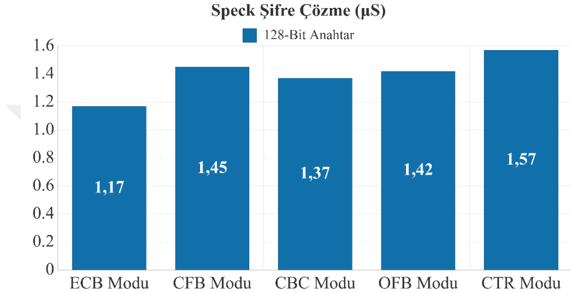
Şekil 3.16. Speck 128 Bit Anahtar Şifre Çözme
