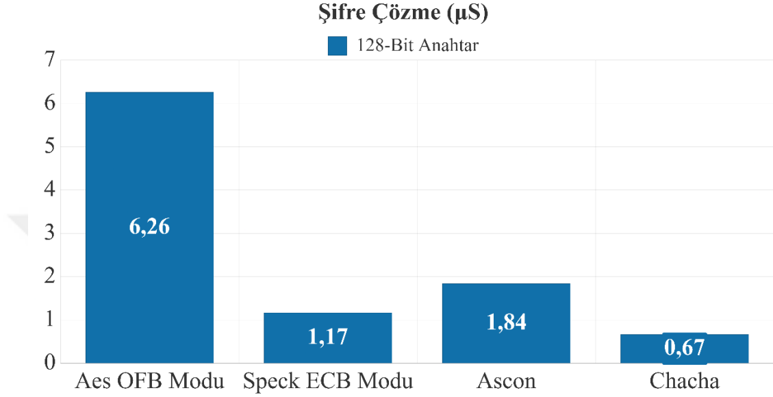
Şekil 3.28. 128 Bit Anahtar Şifre Çözme
