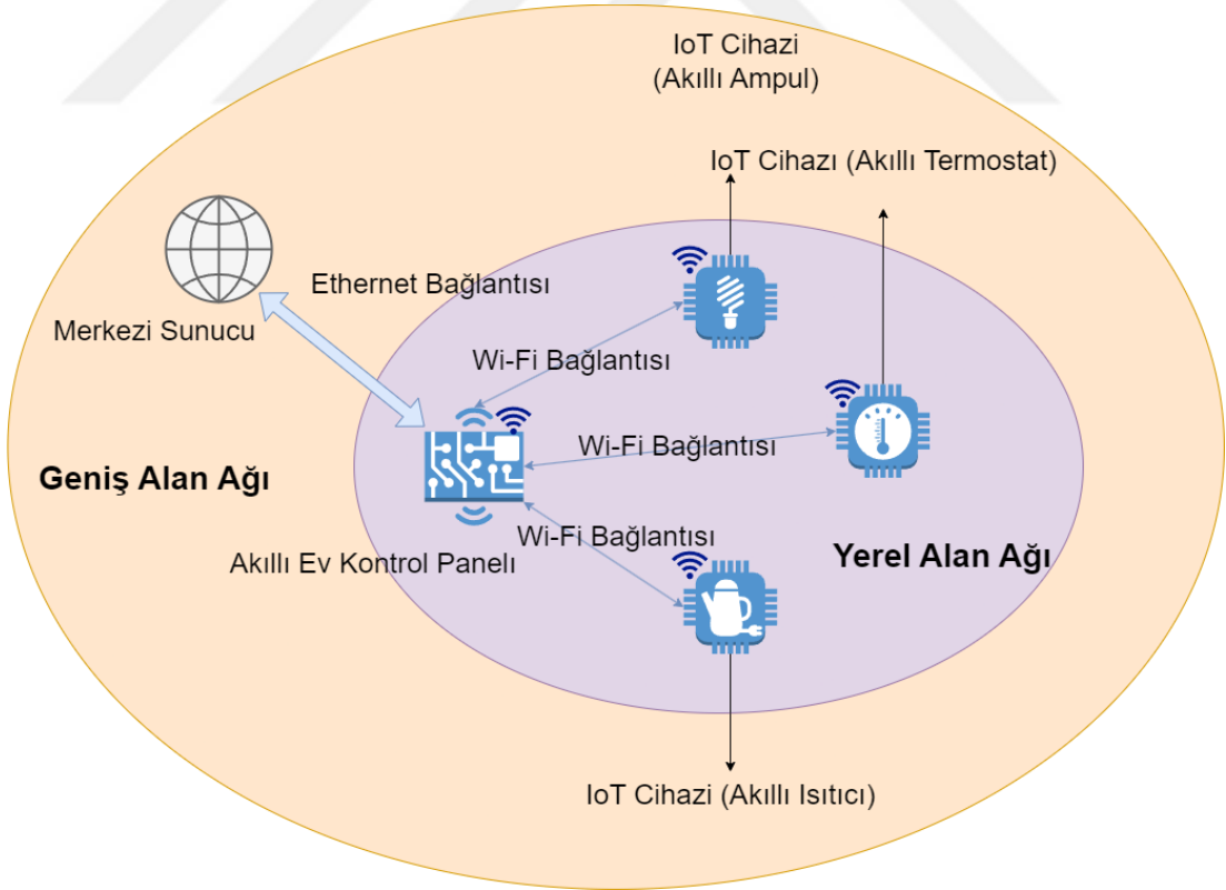
Şekil 2.1. Örnek Akıllı Ev Sistem Mimarisi
