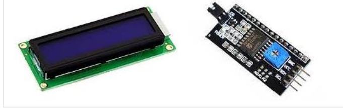
Şekil 2. 7. 16X2 LCD ekran üst ve alt görünümü
