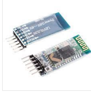
Şekil 2. 8. HC-05 modülü
