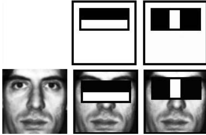
Şekil 2.8: Viola-Jones, Haar Feature Tekniği
