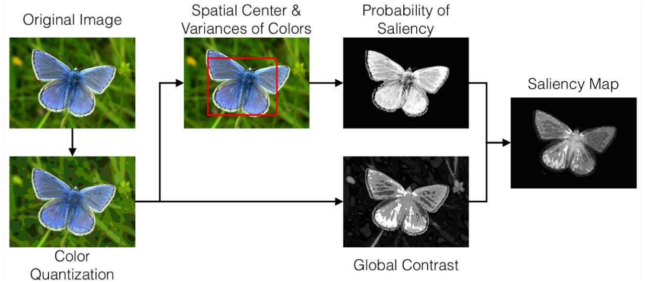
Şekil 3.3: Saliency Masks
