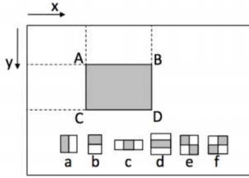
Şekil 2.12: Viola-Jones, İntegral Görüntülerin Haar Feature Dikdörtgenleri
