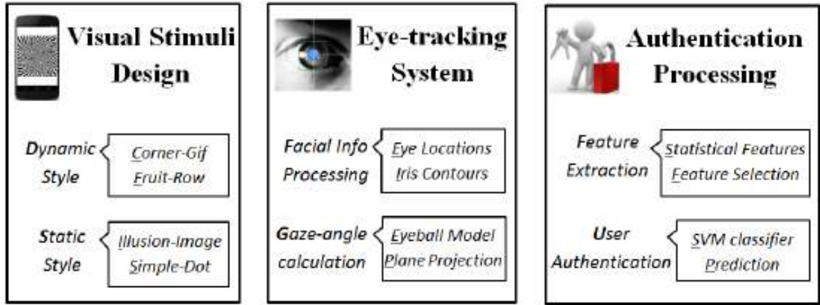
Şekil 6.3: Framework Modülleri
