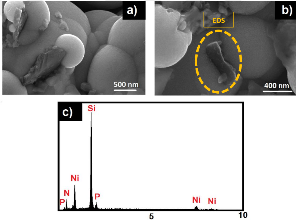
Şekil 6.17. Kaplama banyosunda 20 g/L \text{Si}_3\text{N}_4 konsantrasyonunda elde edilen kompozit NiBP- \text{Si}_3\text{N}_4 (SiN20) kaplanmış numuneye ait a-b) farklı büyütme ölçeklerinde FESEM resimleri ve c) işaretli alanın EDS analizi.
