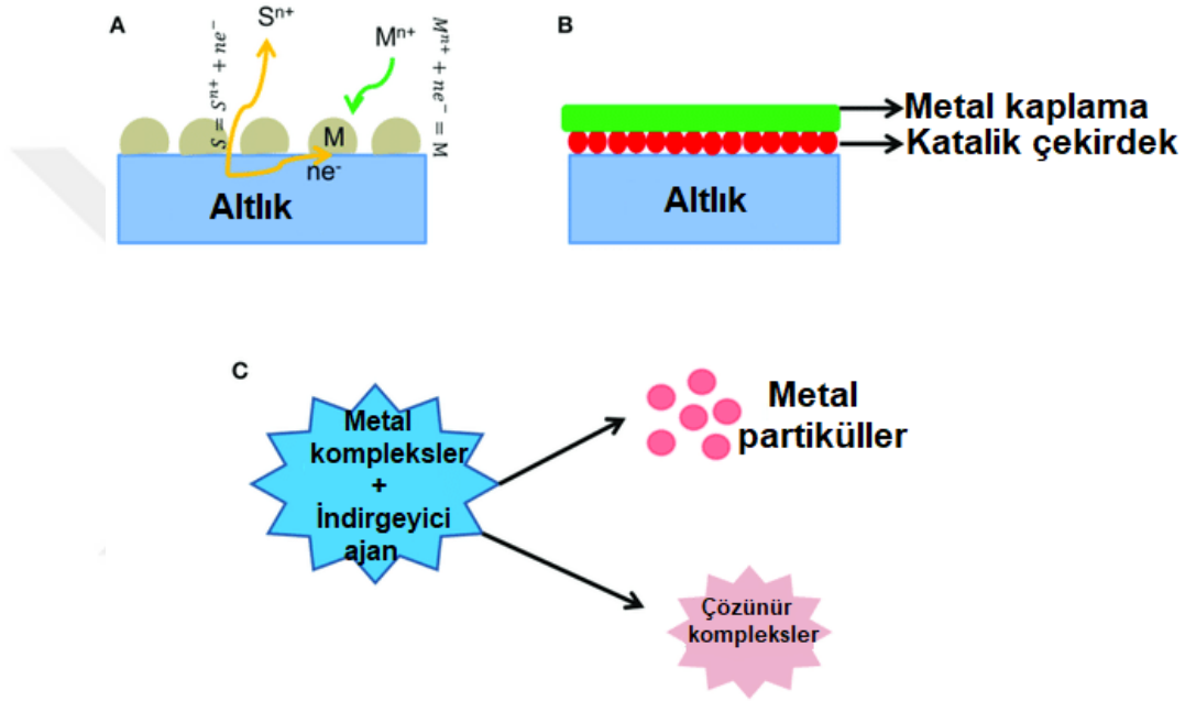
Şekil 3.1. Çeşitli kaplama proseslerinin şematik gösterimi: a) Galvanik yer değiştirme reaksiyonu, b) indirgeyici ajan kullanılarak indirgeme ve c) disproporsiyonlaşma reaksiyonu [48].
