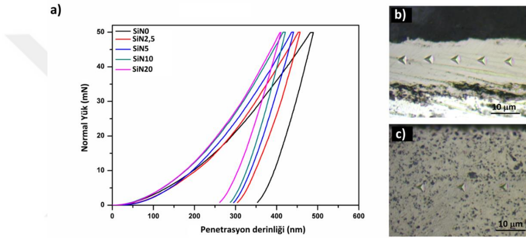
Şekil 6.21. Akımsız \text{Si}_3\text{N}_4 takviyeli NiBP kompozit kaplamaların a) yük-penetrasyon derinliği eğrileri, b) SiN0 ve c) SiN20 nanoindentasyon testleri sonucu meydana gelen izlerin optik görüntüleri.
