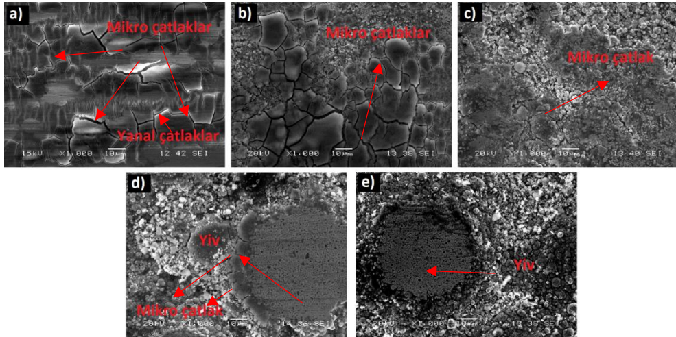
Şekil 6.24. Akımsız NiBP ve NiBP- \text{Si}_3\text{N}_4 kompozit kaplamalarda aşınma izlerinin yüksek büyütme görüntüleri; a) \text{SiN}_0 , b) \text{SiN}_{2,5} , c) \text{SiN}_5 d) \text{SiN}_{10} ve e) \text{SiN}_{20} .
