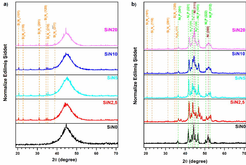
Şekil 6.19. Akımsız \text{NiBP} ve farklı konsantrasyonlarda \text{Si}_3\text{N}_4 takviyeli banyolardan elde edilen numunelere ait a) ısıtıl işlem öncesi ve b) ısıtıl işlem sonrası XRD paternleri.
