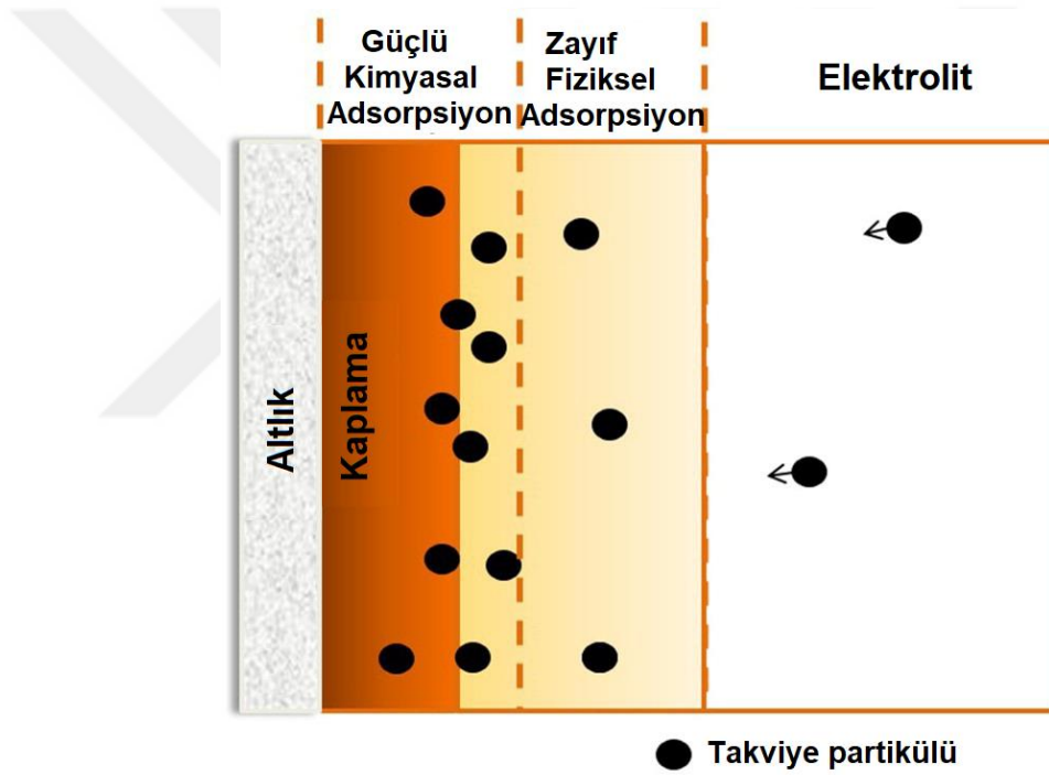
Şekil 4.1. Akımsız kompozit kaplamalar için Guglielmi modelinin şematik gösterimi [75].
