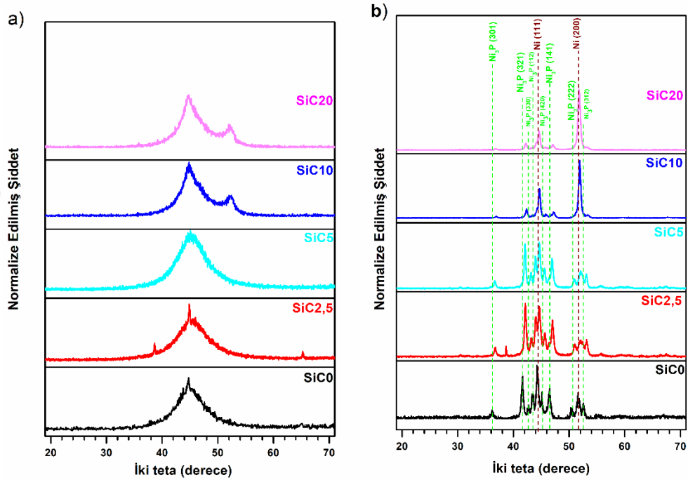
Şekil 6.31. Akımsız NiBP ve farklı konsantrasyonlarda SiC takviyeli banyolardan elde edilen numunelere ait a) ısıtıl işlem öncesi ve b) ısıtıl işlem sonrası XRD paternleri.
