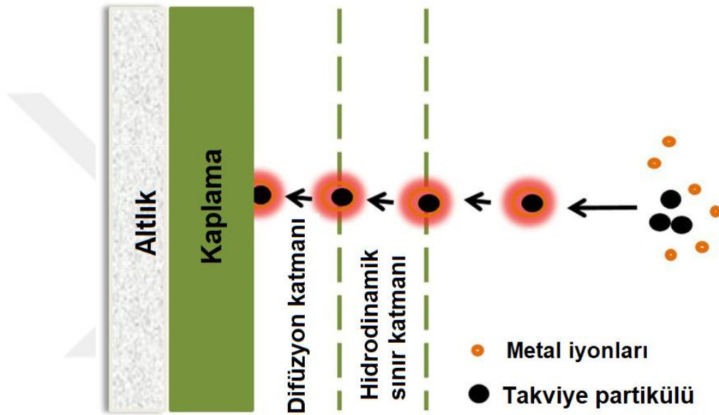
Şekil 4.2. Akımsız nano kompozit kaplamaların çeşitli aşamalarının şematik gösterimi [75].
