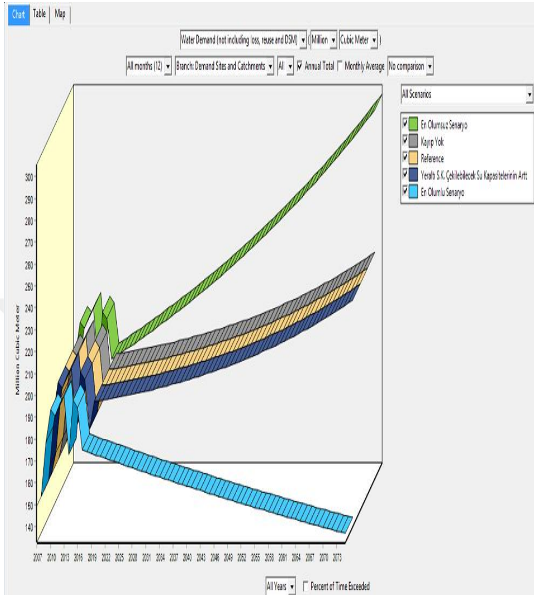
Şekil 4.8. Havzadaki tüm senaryolar için 2007-2075 yılları arasındaki toplam su talebi miktarları (hm 3 ).
