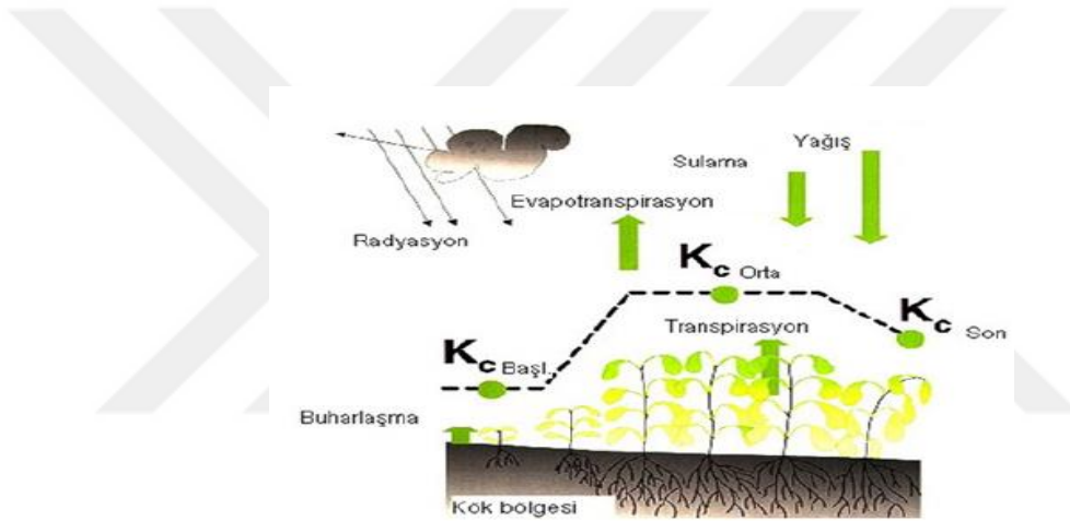
Şekil 1.5. Bitki katsayısının bitki gelişme dönemlerine göre değişimi [18].
