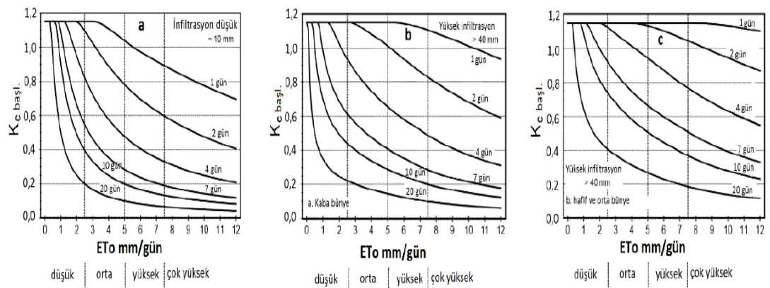
Şekil 1.6. ETo, sulama aralığı, ortalama sulama derinliği ve toprak bünyesine göre ortalama K_c başlangıç değerleri [18].
