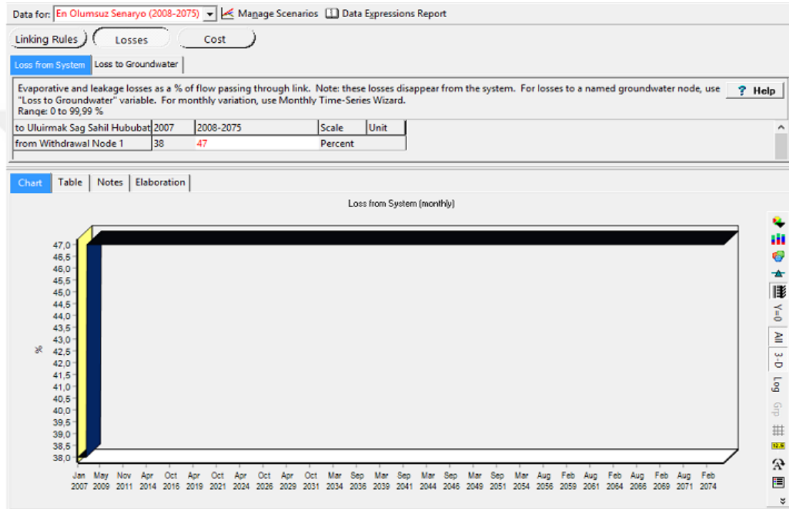
Şekil 3.33. Uluirmak sağ sahil tarım alanı iletim kanalındaki kayıp oranı (en olumsuz senaryo, %).
