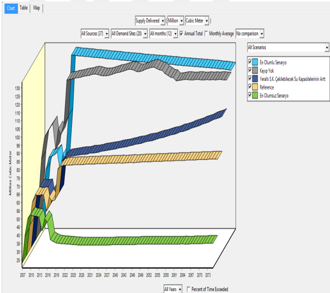
Şekil 4.16. Havzadaki bütün senaryolar için 2007-2075 yılları arasında tüm talep noktalarına kaynaktan tedarik edilen su miktarları (hm 3 ).
