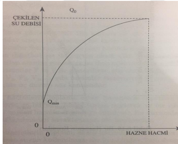
Şekil 1.2. Biriktirme verimlilik eğrisi [7].
