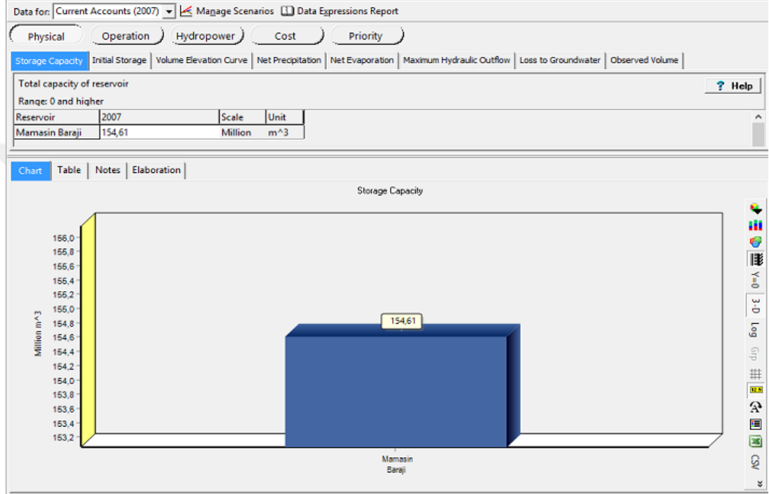
Şekil 3.4. Mamasın barajı depolama kapasitesi (güncel hesaplama senaryosu, hm 3 ).
