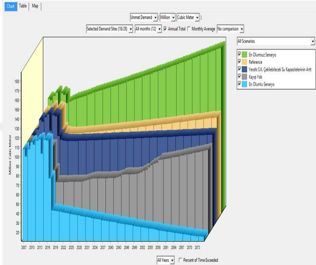
Şekil 4.3. Tarım alanlarının tümünün her bir senaryo için 2007-2075 yılları arasındaki karşılanmamış talep miktarları (hm 3 ).
