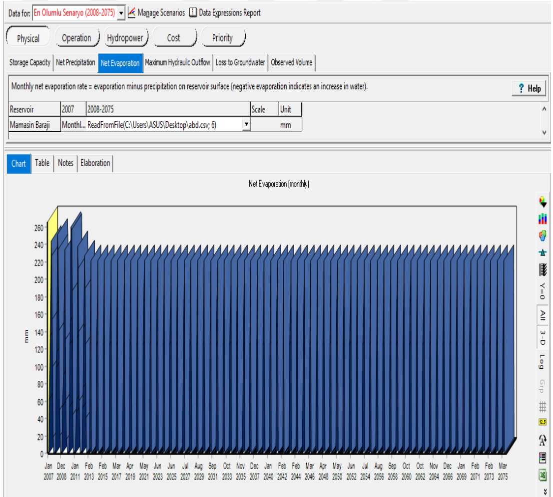
Şekil 3.35. Mamasın barajının 2007-2075 yılları arasındaki buharlaşma miktarları (en olumlu senaryo, mm).
