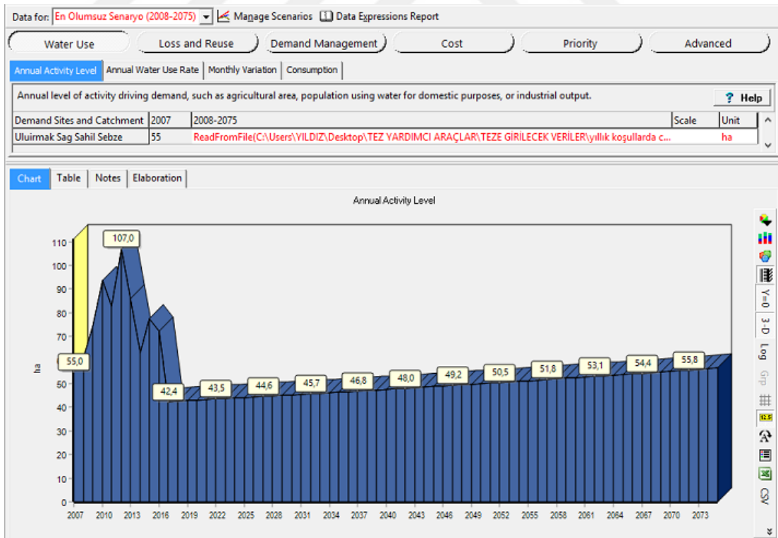
Şekil 3.32. Ulurmak tarım alanı 2007-2075 yılları arasındaki sebze ekim miktarları (en olumsuz senaryo, ha).
