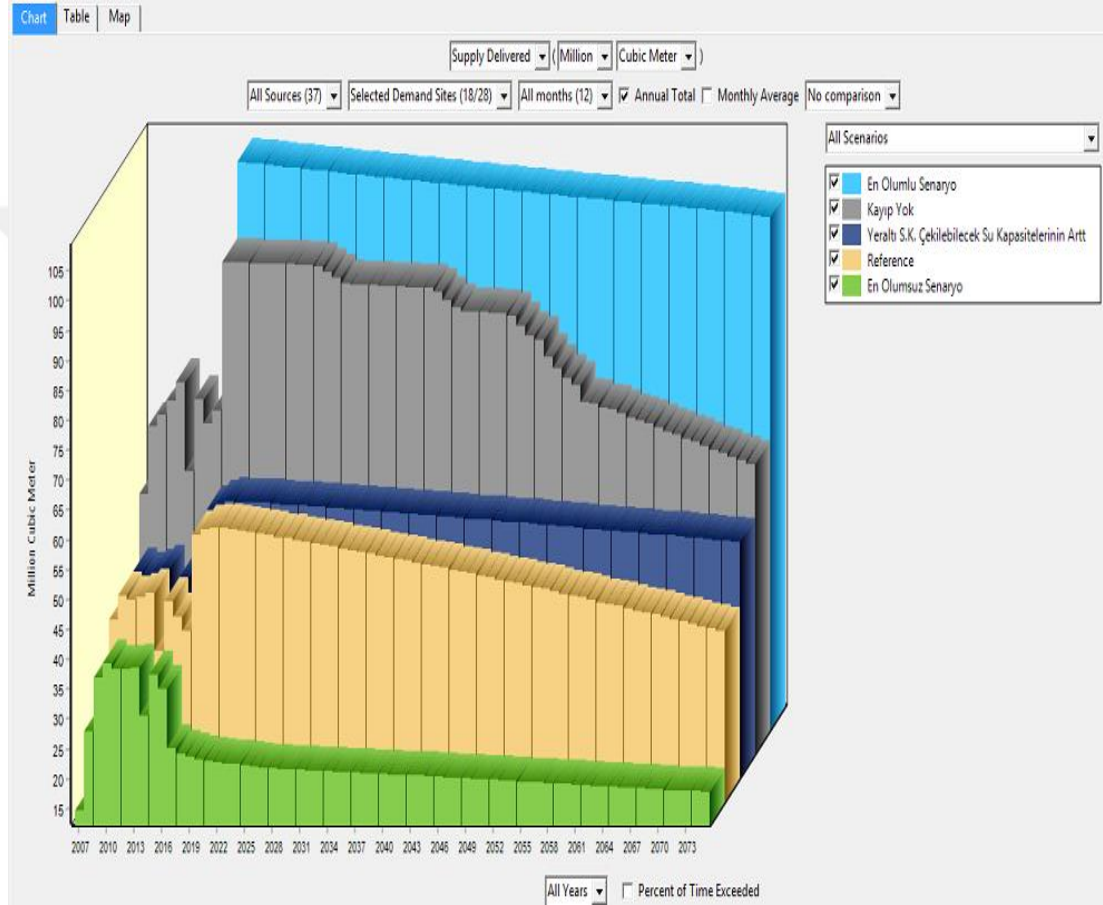
Şekil 4.21. Tarım alanlarının tümüne her bir senaryo için 2007-2075 yılları arasında kaynaktan tedarik edilen su miktarları (hm 3 ).
