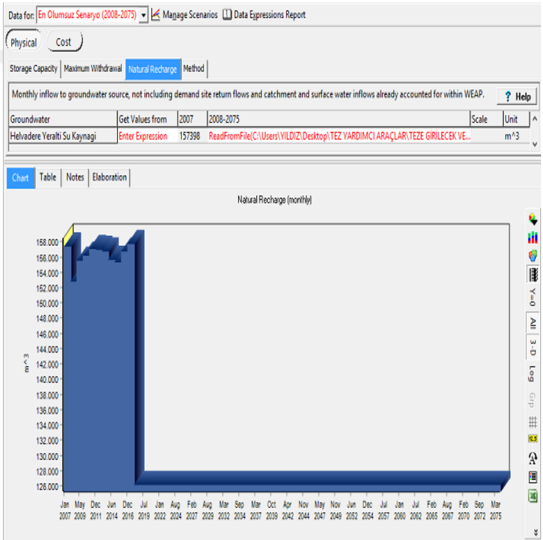
Şekil 3.28. Helvadere yeraltı su kaynağı 2007-2075 yılları arasındaki yeniden dolum miktarları (en olumsuz senaryo, m 3 ).
