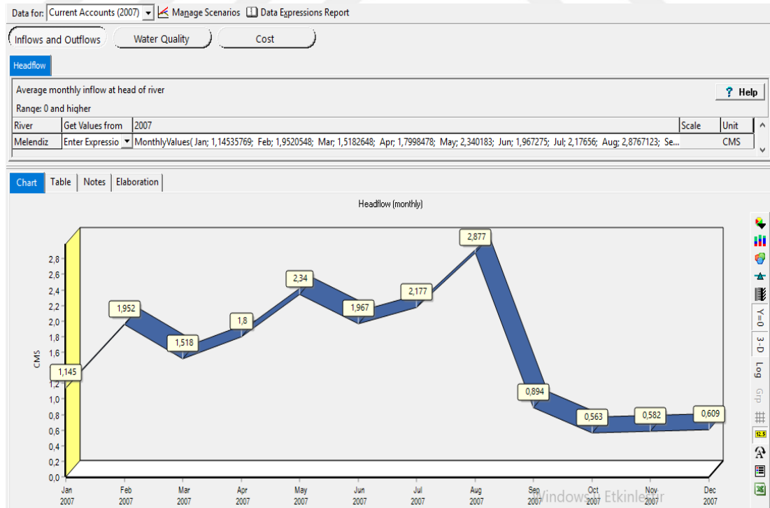
Şekil 3.3. Melendiz çayına ait 2007 yılındaki debi değeri (güncel hesaplama senaryosu, m 3 /s).
