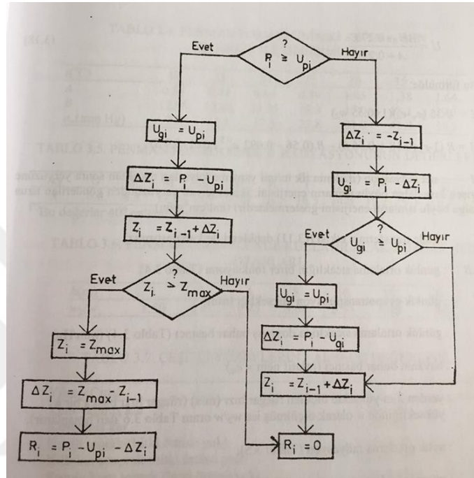
Şekil 1.4. Gerçek evapotranspirasyon hesabı için akım şeması [11].
