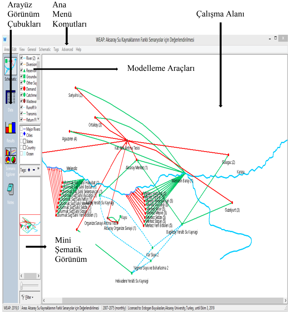
Şekil 2.1. WEAP programı arayüz görünümü.
