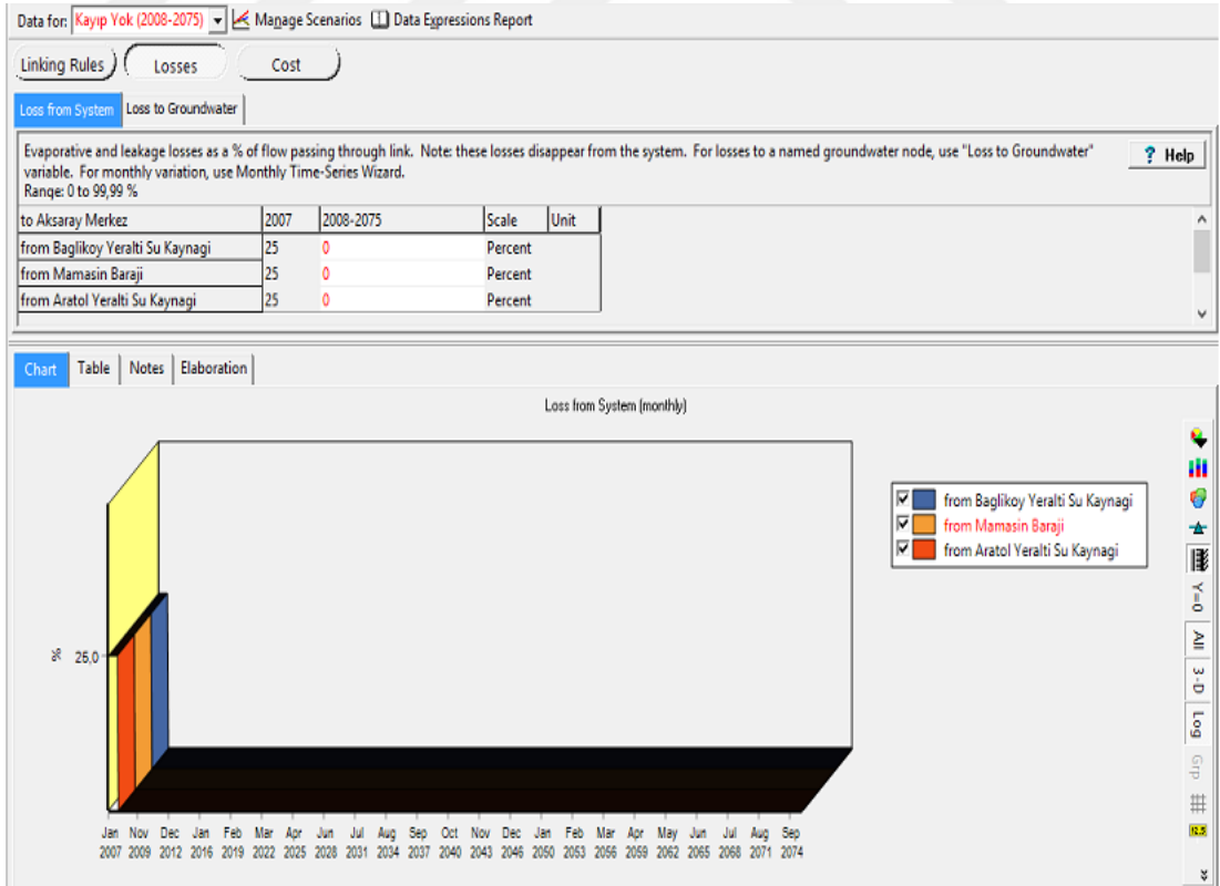
Şekil 3.45. Şehir isale hattındaki kayıp oranı (kayıp yok senaryosu, %).
