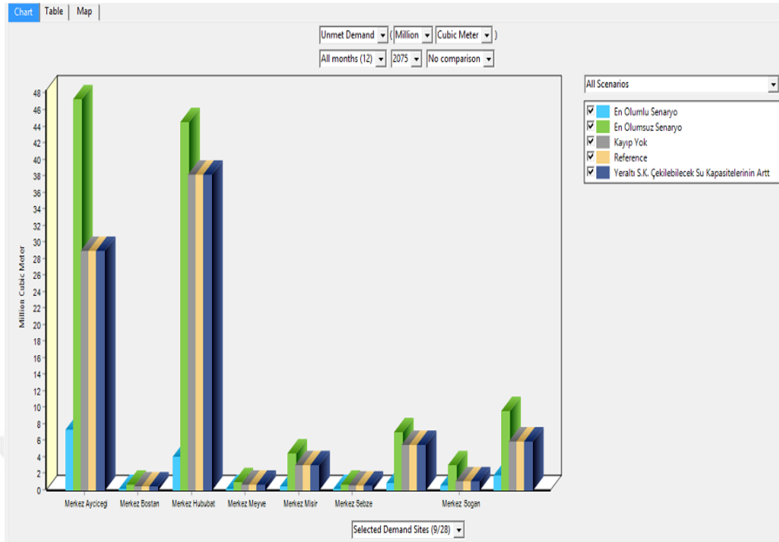
Şekil 4.4. Merkez tarım alanında tüm senaryolar için 2075 yılındaki karşılanmamış talep miktarları ( \text{hm}^3 ).
