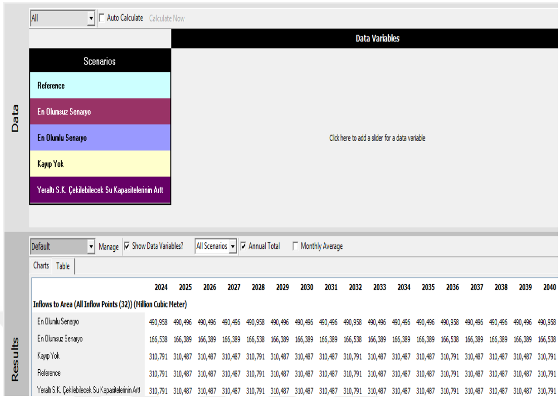
Şekil 4.32. Tüm senaryolar için 2024-2040 yılları arasındaki toplam havza giriş akımları (hm 3 ).
