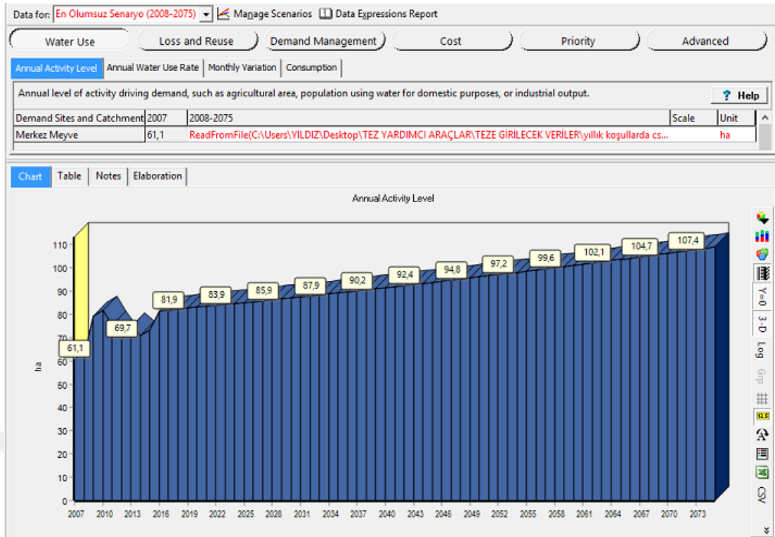
Şekil 3.31. Merkez tarım alanı 2007-2075 yılları arasındaki meyve ekim miktarları (en olumsuz senaryo, ha).
