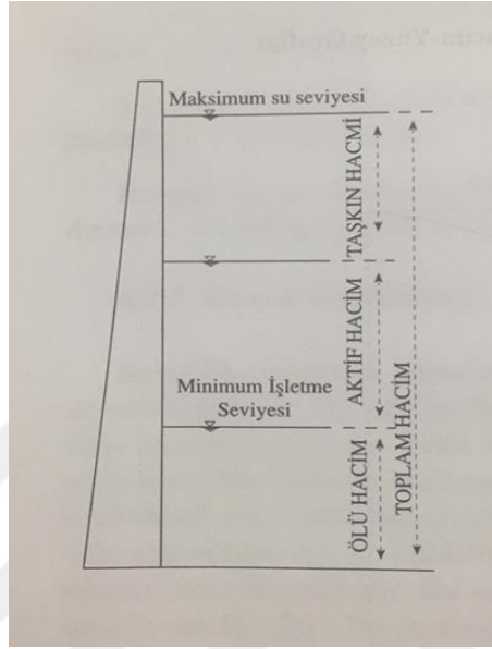
Şekil 1.3. Bir haznenin kısımları [7].
