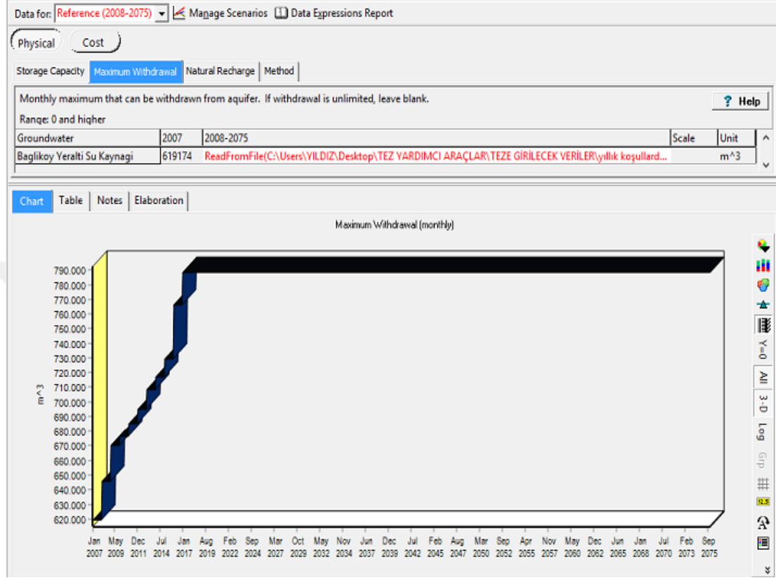
Şekil 3.19. Bağlıköy yeraltı su kaynağından 2007-2075 yılları arasında çekilebilecek maksimum su miktarları (referans senaryo, m³).
