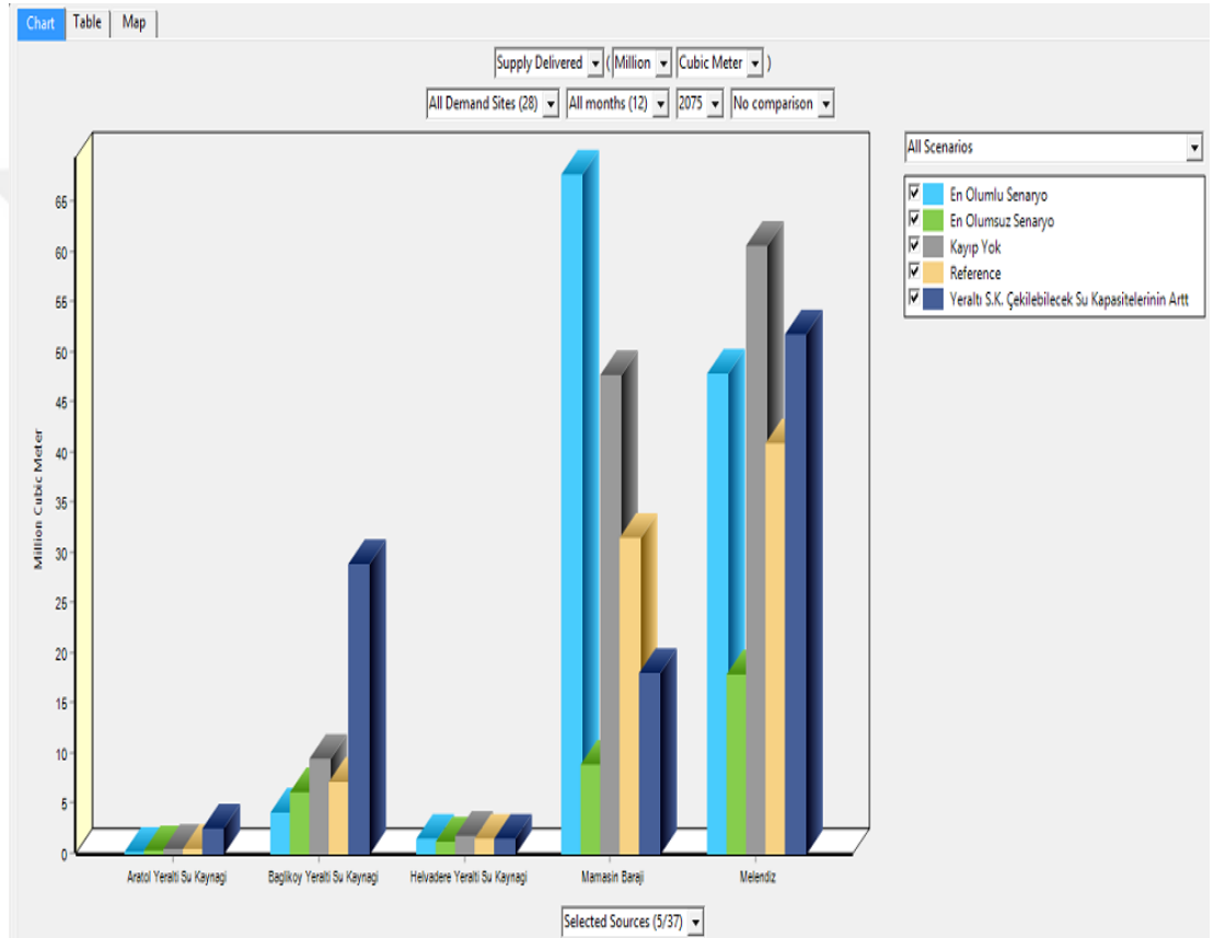
Şekil 4.17. Havzadaki tüm senaryolar için 2075 yılında her bir su kaynağından talep noktalarına tedarik edilen su miktarları (hm 3 ).
