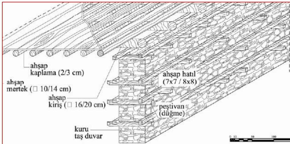
Şekil 2.6. Çift Yönlü Döşeme Detayı [50]
