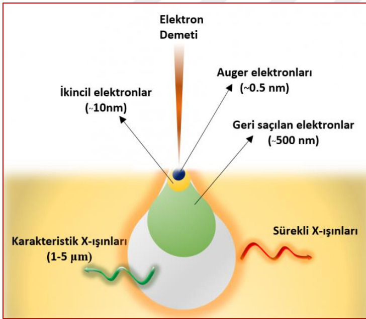
Şekil 3.6. Sem Çalışma Prensibi [54].
