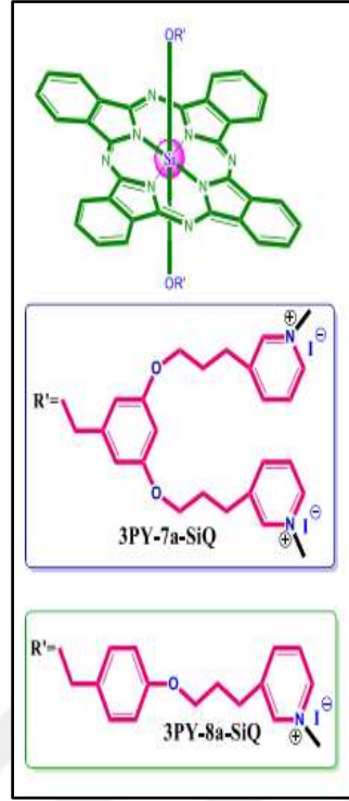
Şekil 20. Aksiyal piridin süstitüeli silisyum ftalosiyanınler ve suda çözüdür türevleri
