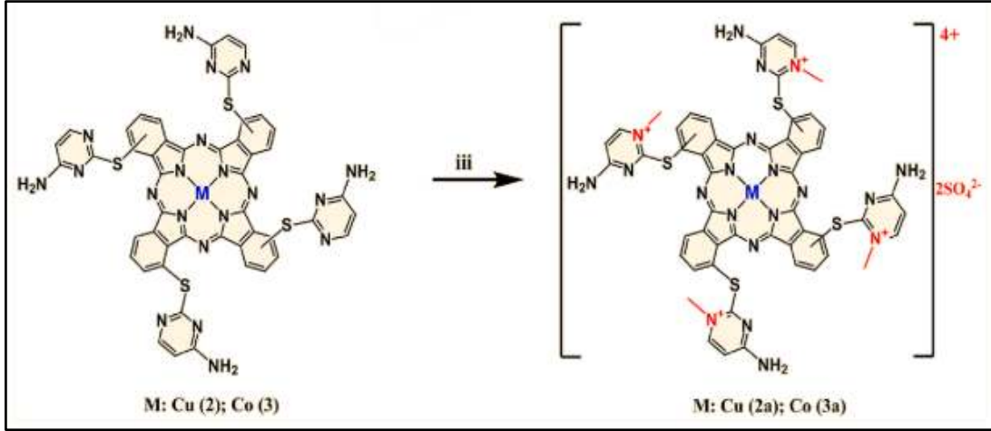
Şekil 23. Periferal tetra 3-[4-(aminopirimidin-2-tyo)] süstitüeli metalli ftalosiyeninler ve suda çözüdür türevleri
