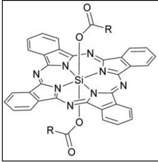
Şekil 11. Aksiyal süstitüe ftalosiyanin örneđi
