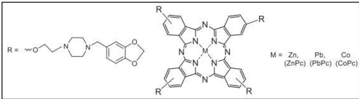
Şekil 25. Periferel tetra 1-(benzo[d][1,3]dioksol-5-metil)piperazin sübstitüeli metalli ftalosiyaninler
