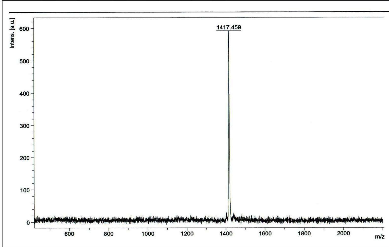
Ek Şekil 6. DFP-Cu Bileşiğinin MALDI-TOF MS KütLe Spektrumu
