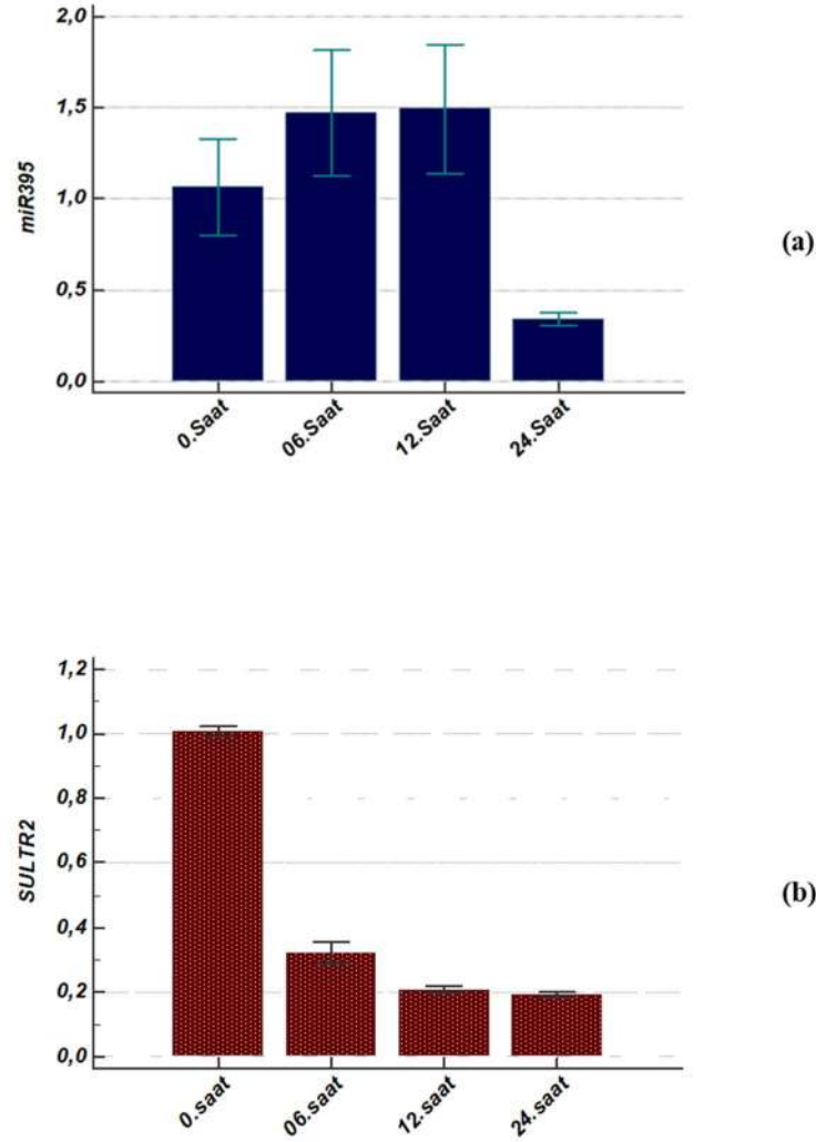
Şekil 4.19: miR395 Bar Grafiği (a) ATP Sülfirilaz Bar Grafiği (b)
