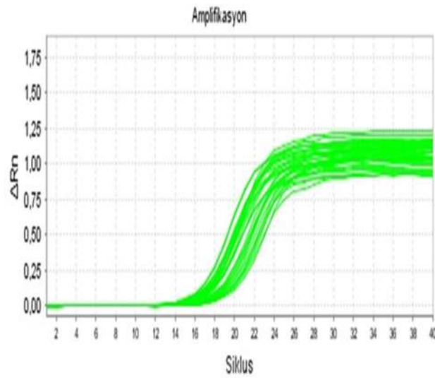
Şekil 4.8: miR161 Erime Piki (a) miR161 Amplifikasyon Eğrisi (b)
