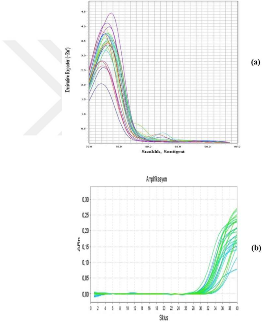
Şekil 4.14: Büyüme Düzenleyen Transkripsiyon Faktörü (GRF) Erime Piki(a) Büyüme Düzenleyen Transkripsiyon Faktörü Amplifikasyon Eğrisi(b)
