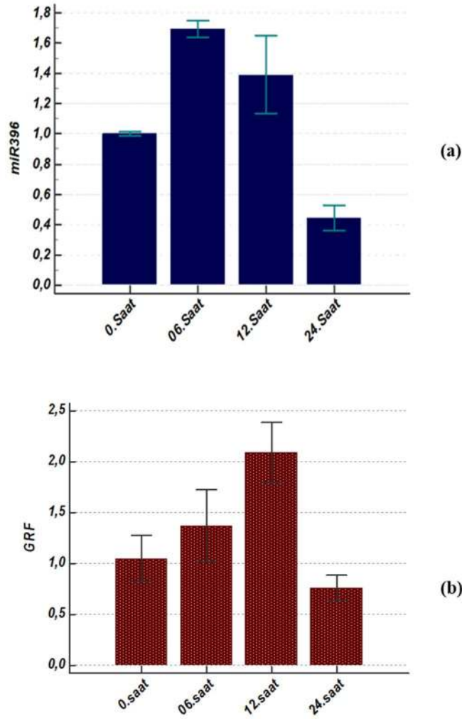
Şekil 4.20: miR396 Bar Grafiği (a) Büyümei Düzenleyen Transkripsiyon Faktörü (GRF) Bar Grafiği (b)
