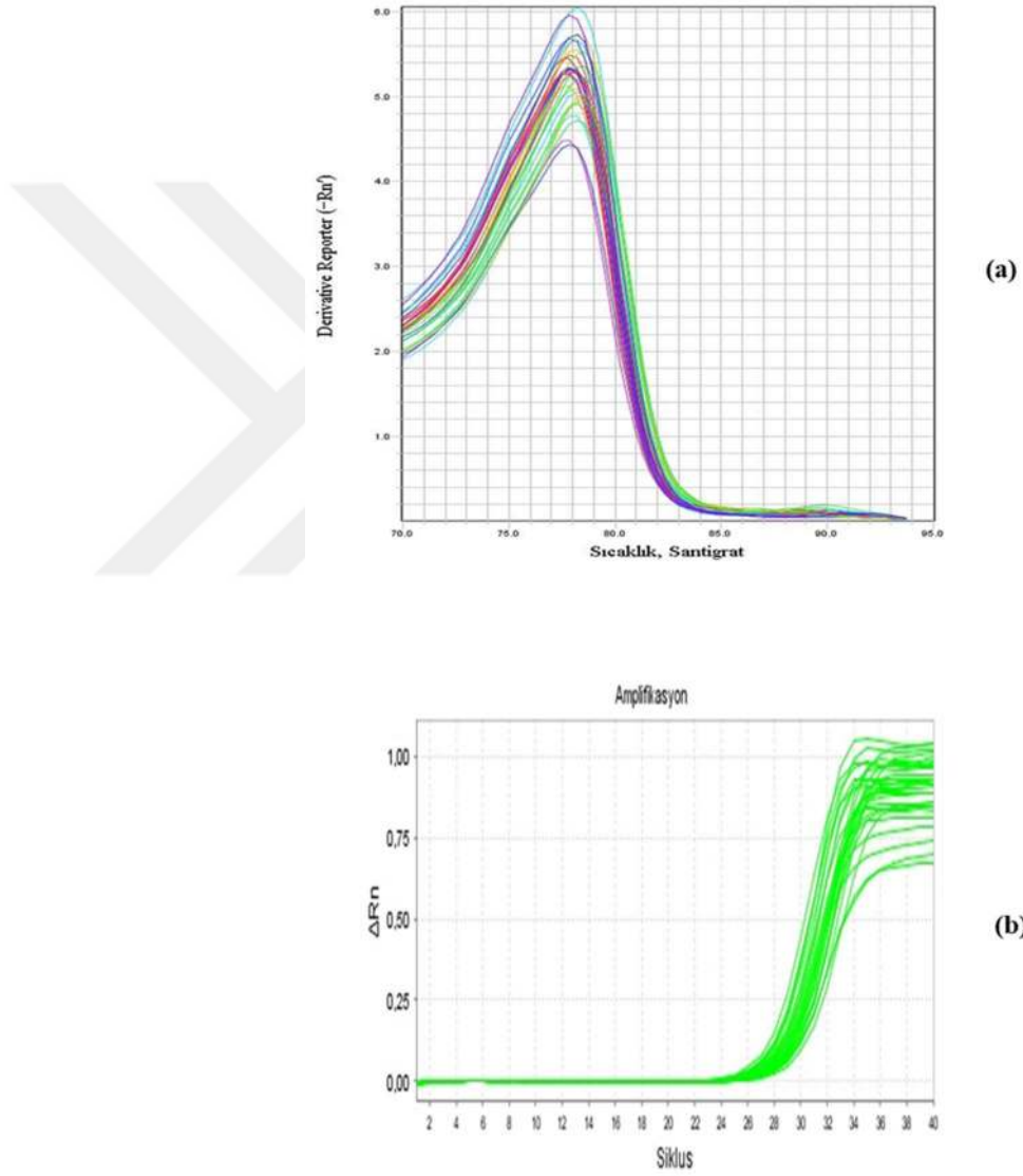
Şekil 4.10: Squamosa promotör bağlanma benzeri protein Erime Piki (a) Squamosa promotör bağlanma benzeri protein Amplifikasyon Eğrisi (b)
