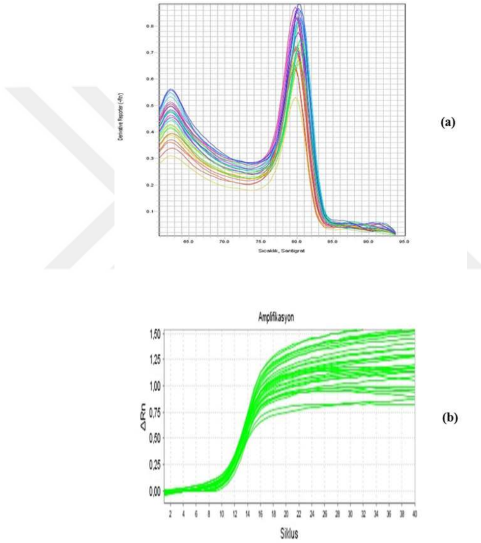
Şekil 4.4: miR159 Erime Piki (a) miR159 Amplifikasyon Eğrisi (b)
