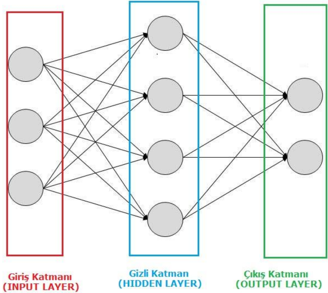
Şekil 2.15. YSA Modeli
