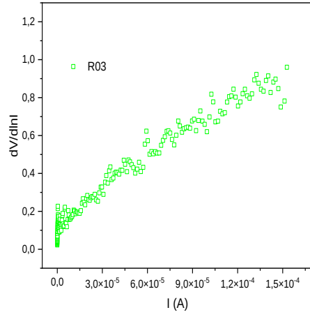
Şekil 4.4. Al/p-Si, katkısız ve arayüzü Al katkılı Al/ZrO 2 /p-Si (MOS) yapılarının dV/d(\ln I) - I grafikleri.
