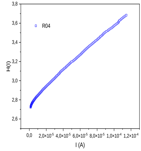
Şekil 4.5. Al/p-Si, katkısız ve arayüzü Al katkılı Al/ZrO 2 /p-Si (MOS) yapılarının H(I) - I grafikleri.
