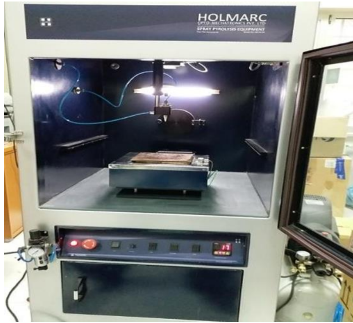
Şekil 2.16. Püskürtme sistemi (Batman Üniversitesi)
