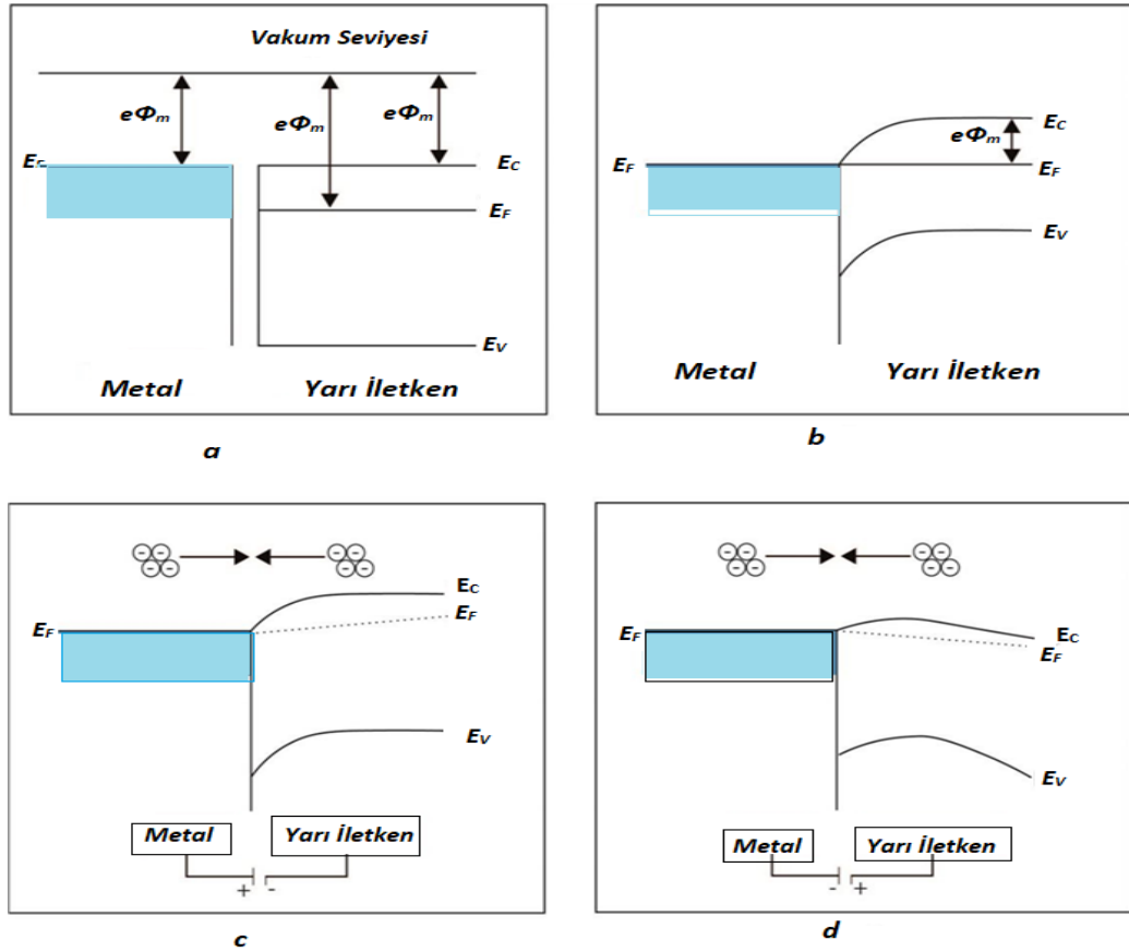
Şekil 2.2. \Phi_M < \Phi_S olması durumunda metal/n-tipi yarıiletken omik kontaklarda, a) Metal/yarıiletken kontak yapılmadan önce, b) Metal/yarıiletken kontakta yapıldıktan sonra, c) Gerilim değeri V < 0 olduğunda d) Gerilim değeri V > 0 olduğunda
