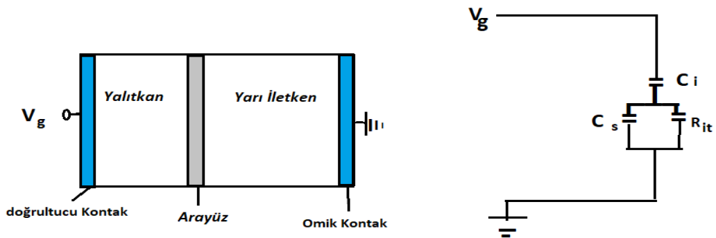
Şekil 2.3. Metal/Oksit/Yarıiletken (MOS) eklemi ve eşdeğer devresi.
