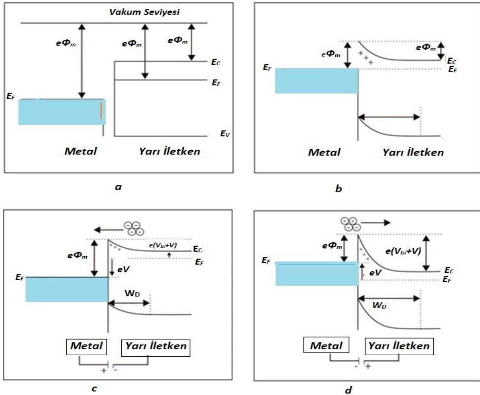
Şekil 2.1. ( \phi_M > \phi_S ) değeri ise metal/n-tipi yarıiletken doğrultucu kontak için; a) kontaktan yapılmadan önce b) kontaktan yapıldıktan sonra termal dengede c) uygulanan gerilim V < 0 d) uygulanan gerilim V > 0
