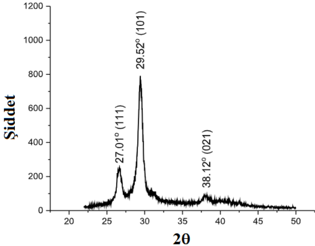
Şekil 4.1. p-Si yüzeyi kaplanmış \text{ZrO}_2 ince film yapısının XRD desenleri.
