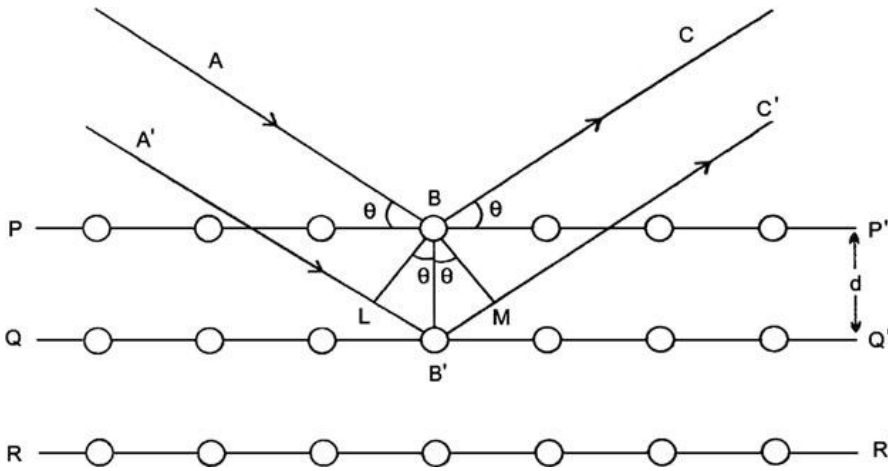
řekil 3.3. X ışınlarının atomlar arası düzlemde kırılması. PP' , QQ' ve RR' bir kristalde birbirini takip eden birbirinden d kadar uzakta paralel atom düzlemlerini göstermektedir.
