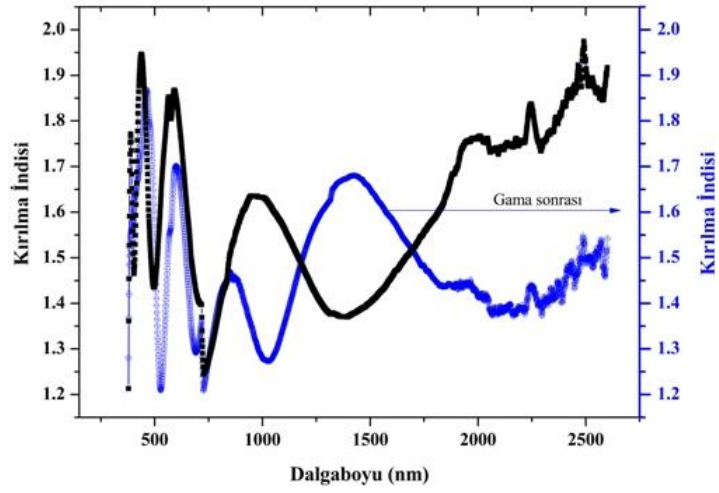
Şekil 4.11. ZnO filmi dalga boyuna karşı kırılma indisleri grafiği
