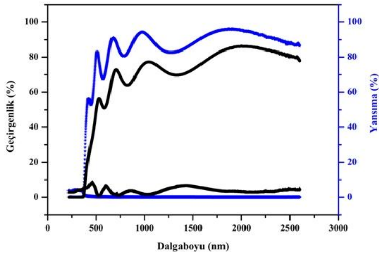
Şekil 4.10. 2AZO geçirgenlik ve yansımada grafiği
