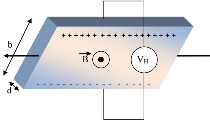
Şekil 3.6. Akım taşıyan iletkene etkiyen manyetik alan ve yüklerin durumu
