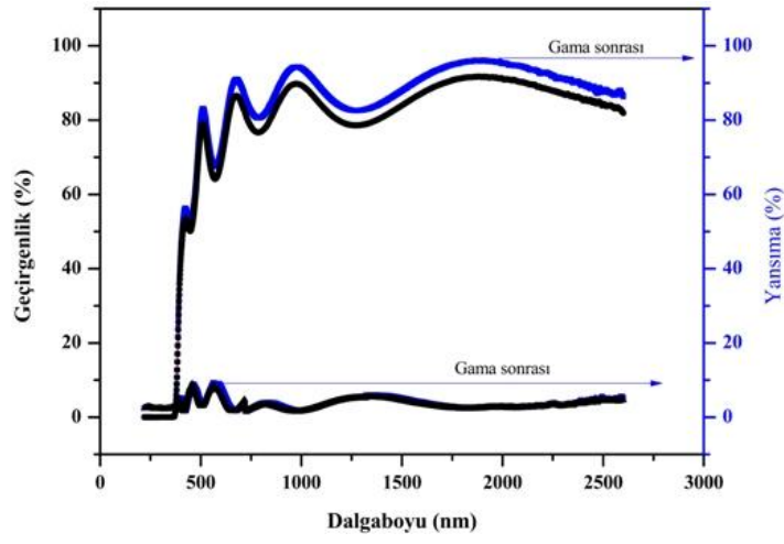
Şekil 4.9. 1AZO geçirgenlik ve yansımada grafiği
