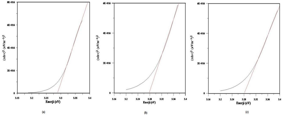
Şekil 4.7. İnce filmlerin için (\alpha h\nu)^2 –enerji grafikleri. (a) Katkısız ZnO filmi yasak enerji bant aralığı (b) 1AZO filmi yasak enerji bant aralığı (c) 2AZO filmi yasak enerji bant aralığı.
