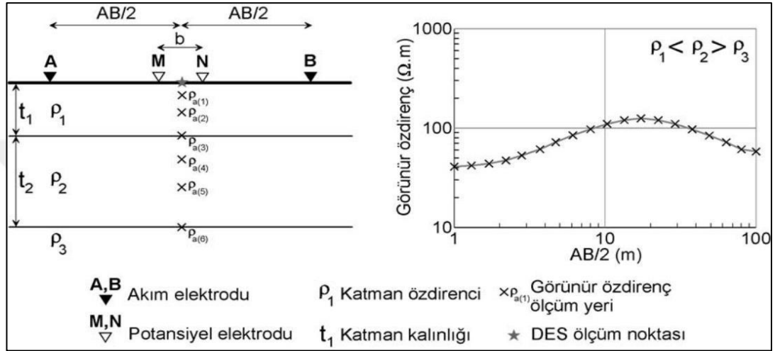
Şekil 4.7. Düşey elektrik sondaj (DES) ölçüm sistemi (üç katmanlı yer altı modeli ve görünür öz direnç eğrisi) [32]
