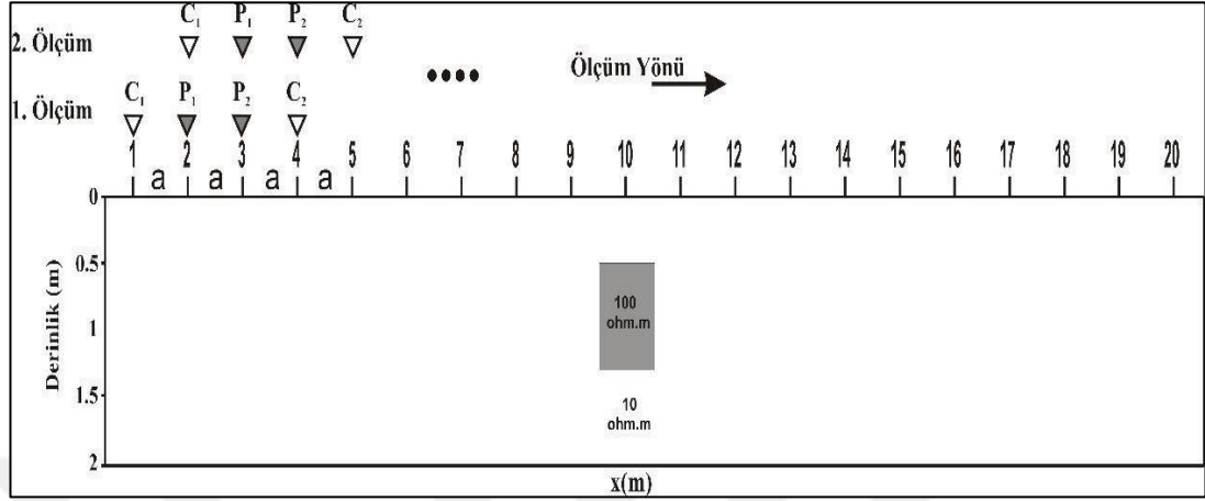
Şekil 4.8. Wenner elektrot dizilimi ile profil ölçümü planı
