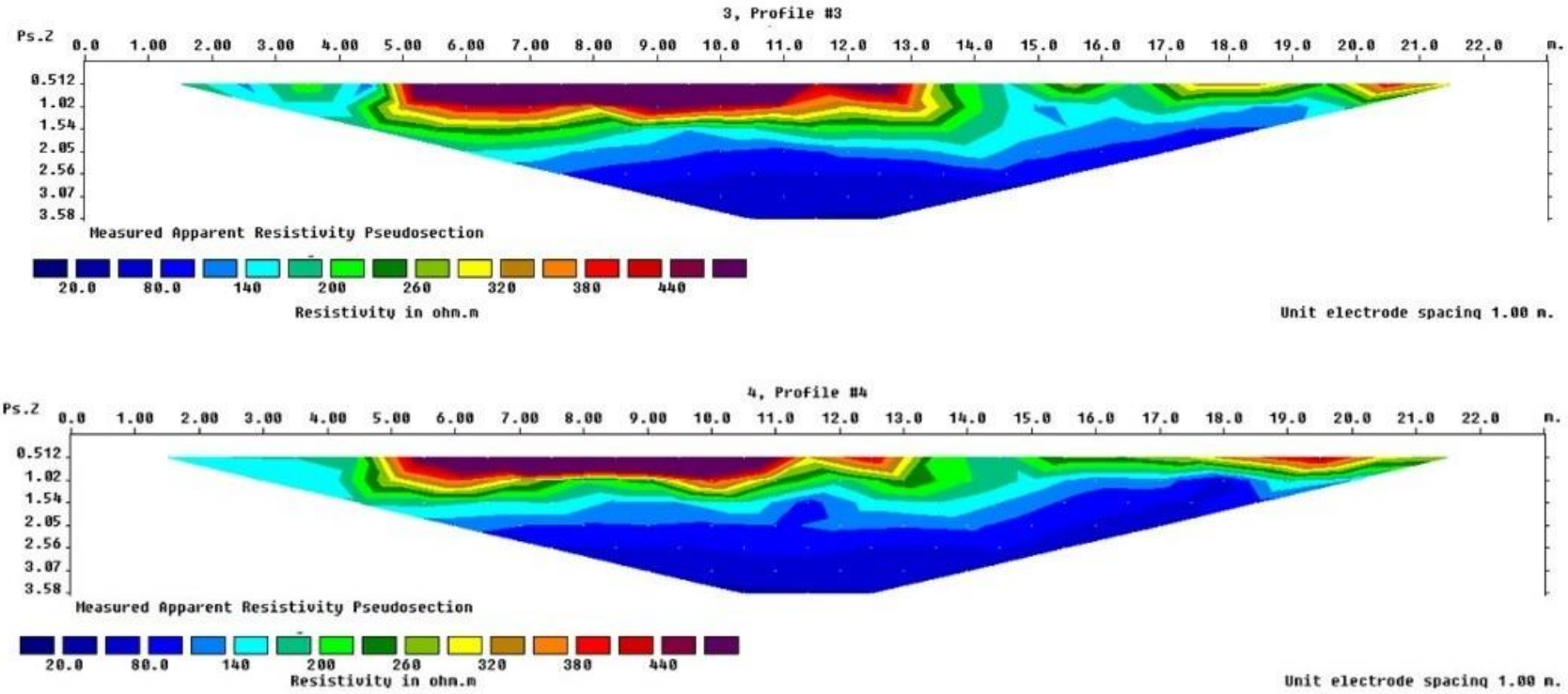
Şekil 6.6. Kilise alt kısım Wenner elektrot dizilimi (yukarıdan aşağı 3. ve 4. Profillere ait ham veriler)
