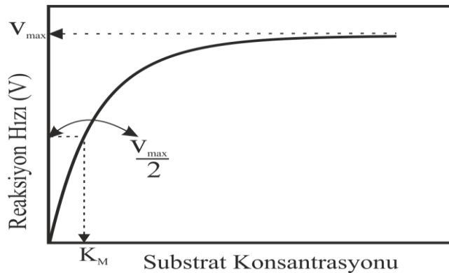
Şekil 1.3. Michaelis-Menten grafiği
