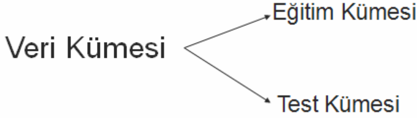
Şekil 3.6.1.1- Veri Kümesi
