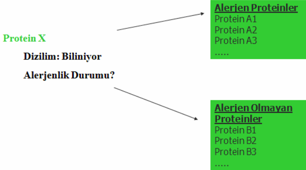
Şekil 3.6.3.1 Sınıflandırma
