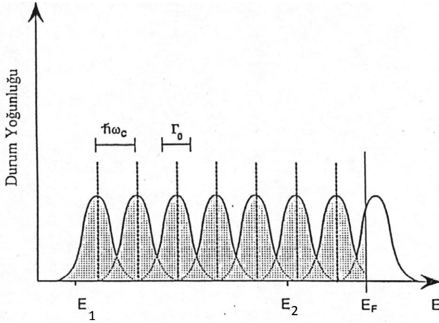
Şekil.2.6. (a) Sıfır magnetik alanda ve (b) 2DEG düzlemine dik olarak magnetik alan uygulandığında durum yoğunluğunun enerjiyle değişimi. Düşey kesikli çizgiler \delta -fonsiyonu tipi Landau düzeylerini göstermektedir. Gaussian eğriler ise çarpışmalar nedeniyle genişlemiş Landau düzeylerini göstermektedir E_1 ve E_2 altband enerjileri, E_F Fermi enerjisi ve \Gamma_0 Landau düzeyinin yarı yüksekliğindeki tam genişliğidir [58].
