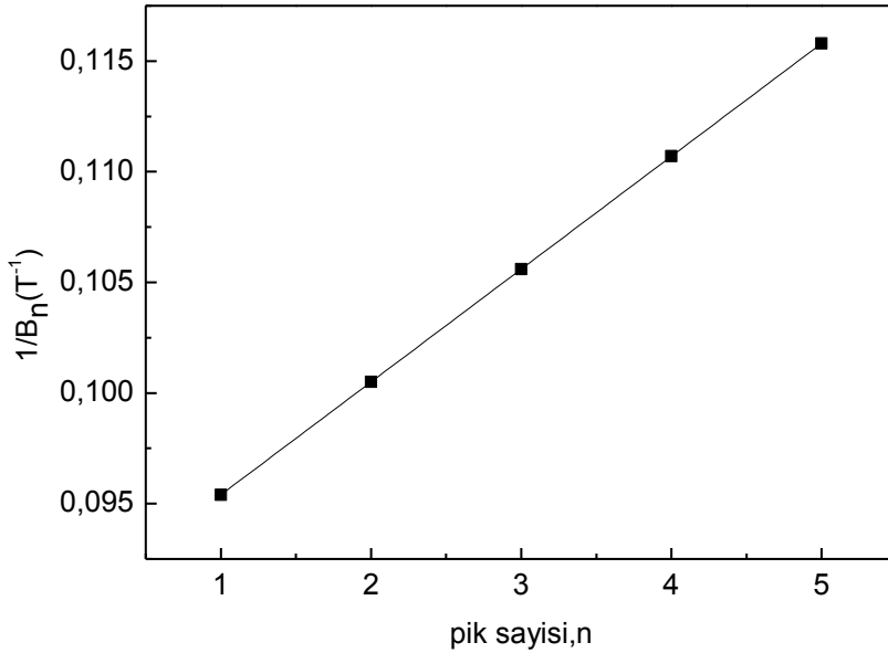
Şekil.5.9. \text{Al}_{0,25}\text{Ga}_{0,75}\text{N}/\text{GaN} heteroeklem örnekte SdH osilasyonları periyodunun elde edilmesi.
