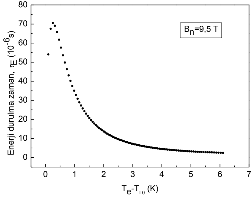
Şekil.6.6. \text{Al}_{0,25}\text{Ga}_{0,75}\text{N}/\text{GaN} heteroeklem örneklerde 2D elektronların enerji durulma zamanının elektron sıcaklığı ile değişimi.
