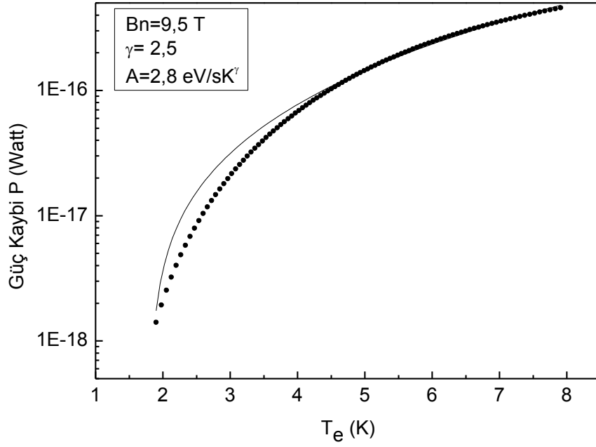
Şekil.6.4. \text{Al}_{0,25}\text{Ga}_{0,75}\text{N}/\text{GaN} heteroeklem örnekte deneysel P(T_e) verilerinin Eş. 2.69'da tanımlanan kuramsal bağıntı ile karşılaştırılması.
