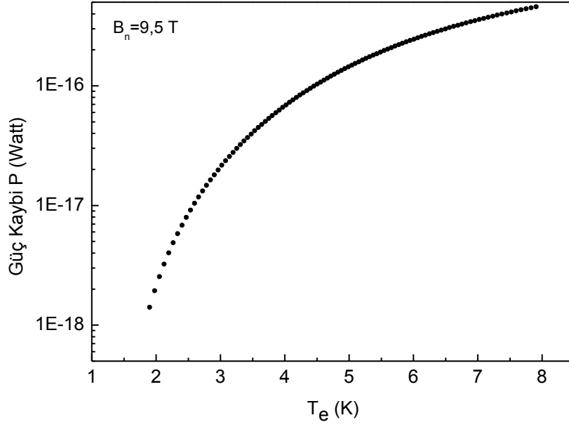
řekil.6.3. \text{Al}_{0,25}\text{Ga}_{0,75}\text{N}/\text{GaN} heteroeklem rnekte 2D elektron g kaybının elektron sıcaklıęı ile deęiřimi. T_{LO} en dřk rg sıcaklıęıdır.
