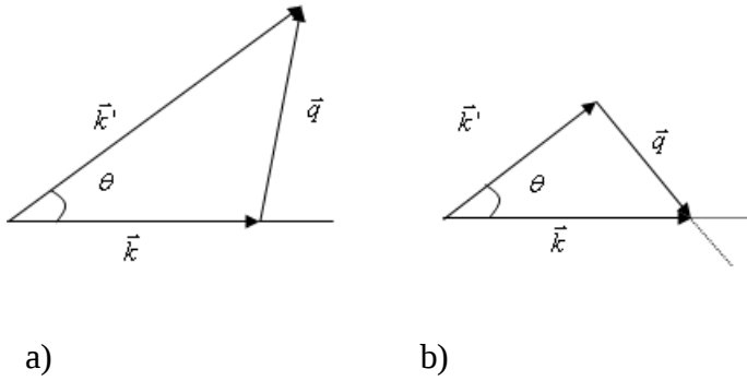
Şekil.2. 7. (a) Fonon soğurulması ve (b) fonon yayılması süreçlerinin şematik gösterimi.
