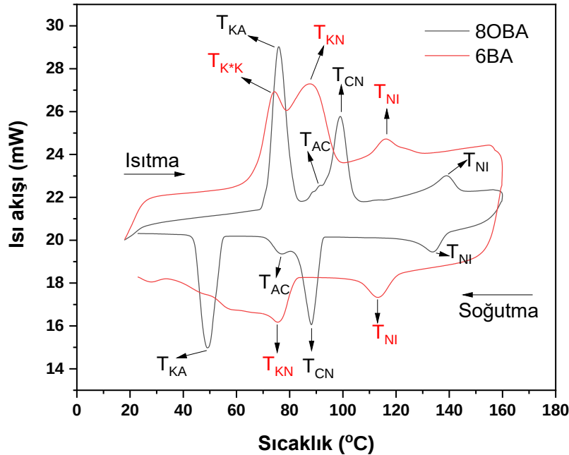
Şekil 4. 11. 8OBA ve 6BA sıvı kristallerinin DSC sonuçları
