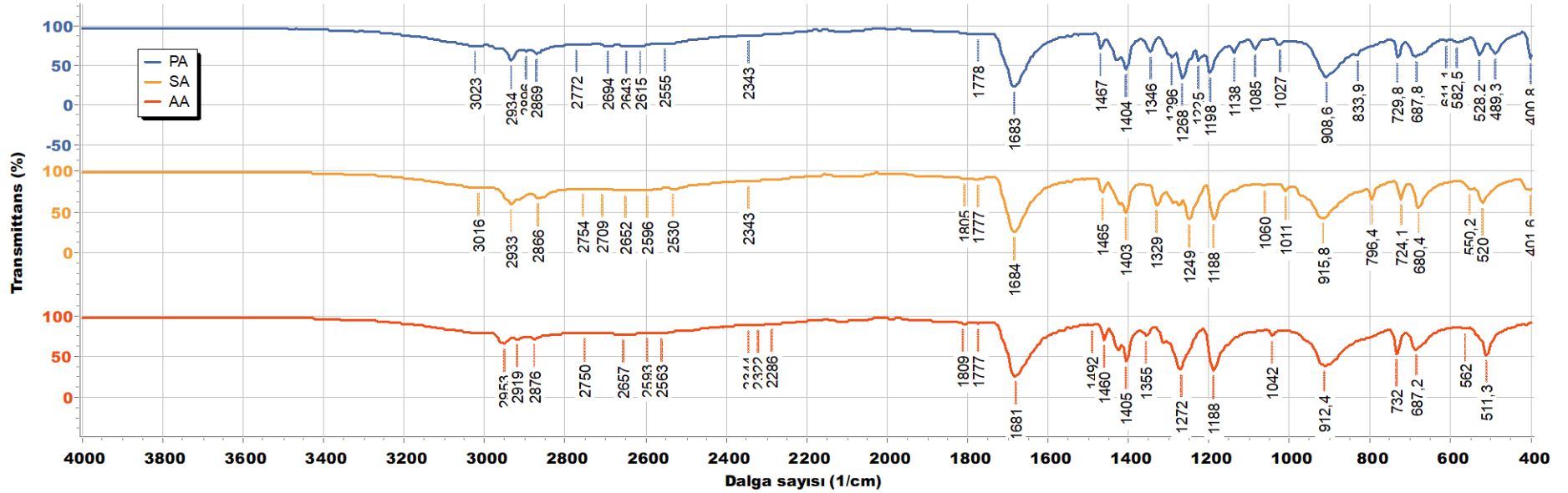
Şekil 4. 2. Sıvı kristal özellik göstermeyen PA, SA ve AA kimyasallarının FTIR spektrumları
