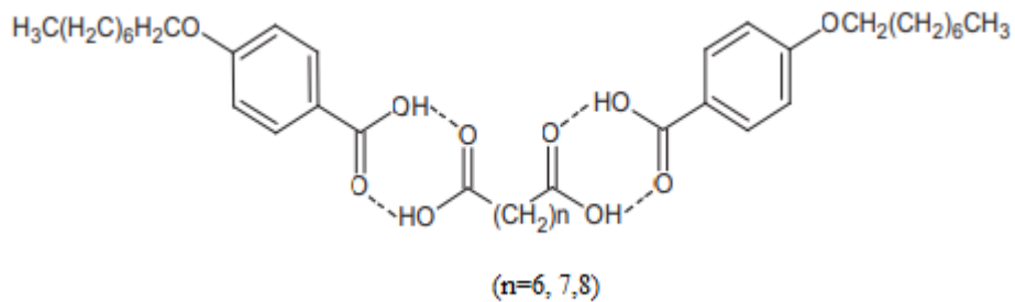
Şekil 3. 1. 8OBA/X komplekslerinin moleküler yapısı (X = AA olduğunda n = 6, X=PA olduğunda n=7, X=SA olduğunda n=8)
