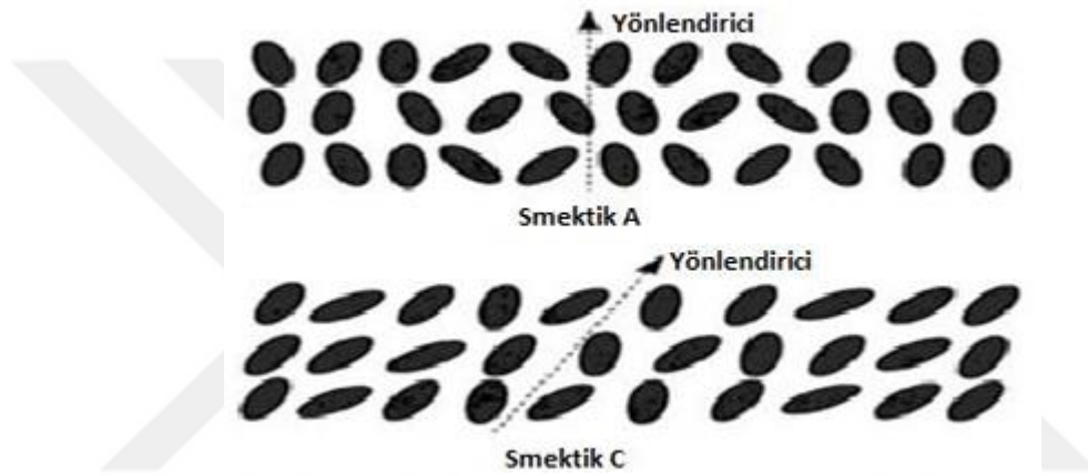
Şekil 1. 5. Smektik-A ve Smektik-C fazları ( Khoo, 2007)
