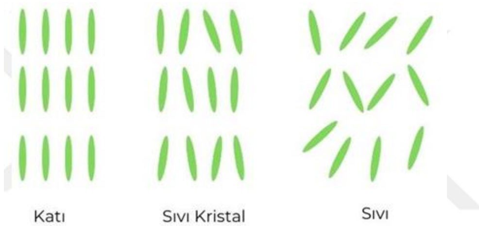
Şekil 1. 1. Moleküllerin katı, sıvı ve sıvı kristal fazları (Emek, 2007)
