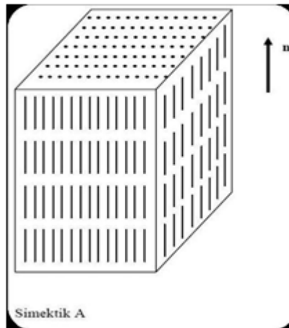
Şekil 1. 7. Smektik-A fazına sahip bir sıvı kristal malzeme yapısı (Ekici, 2014)
