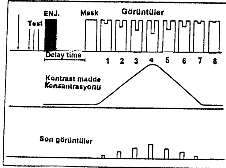
Şekil 5: DSA'da Test Ekspojurları, Enjeksiyon, Delay time, Mask ve Görüntü ilişkisi. Sayılar ile gösterilen görüntülerden, matematiksel olarak "mask" çıkarıldığında, en alttaki son görüntüler elde edilir.
