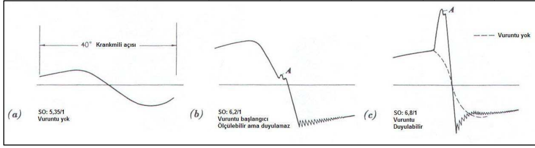
Şekil 2.12. SO artışının vuruntuya etkisi (CFR motoru, 900 min -1 , 32° AA) [19]
