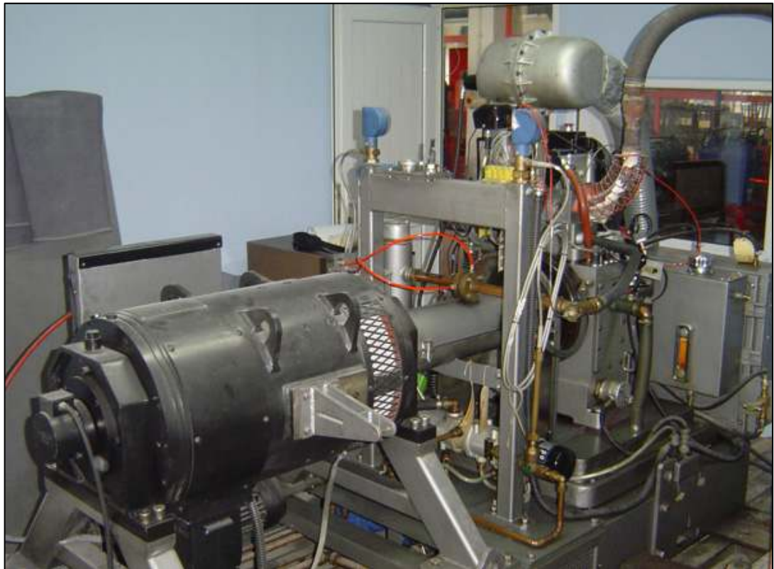
Resim 4.2. Dinamometre
