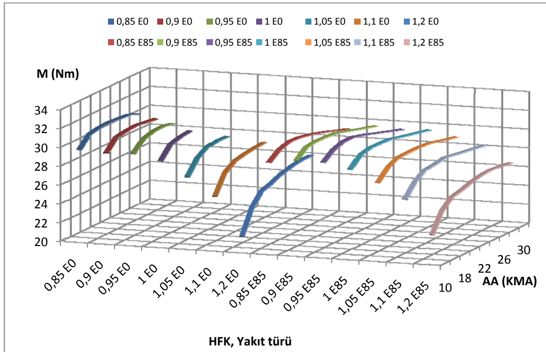
Şekil 5.1. Hava fazlalık katsayısı ve ateşleme avansına bağlı olarak motor momenti değişimi (SO: 10/1, Motor devri: 1500 \text{ min}^{-1} , Yakıt Türü: E0 ve E85)
