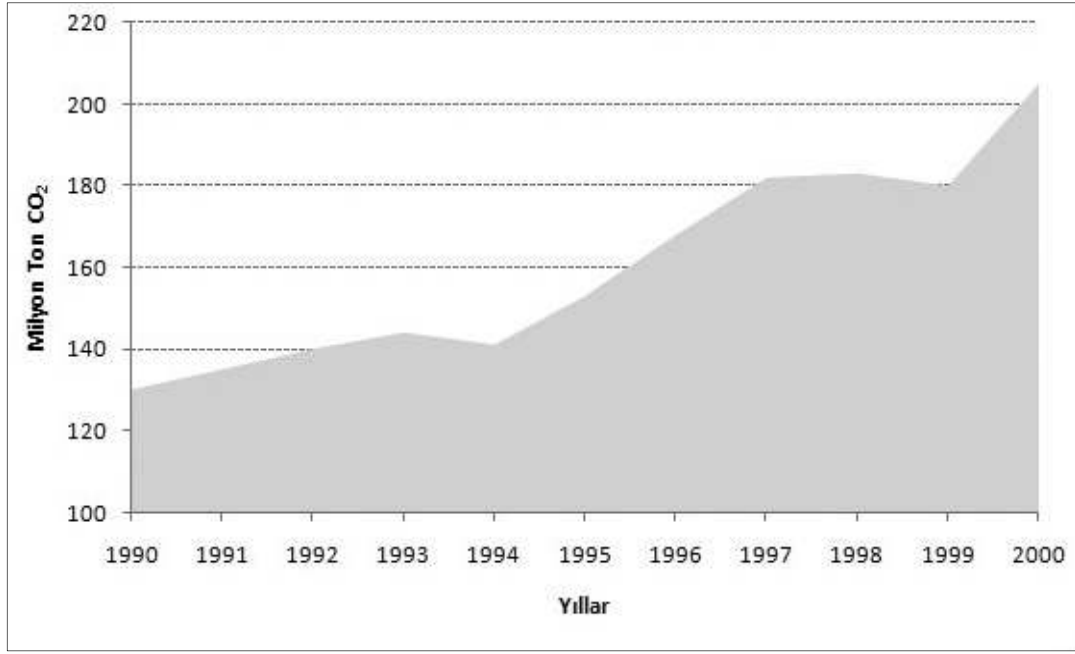
Şekil 2.6. Türkiye’de yıllar itibariyle CO 2 miktarı değişimi [6]
