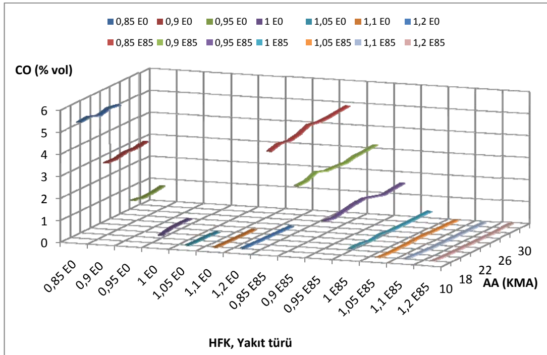
Şekil 5.16. HFK ve ateşleme avansına bağlı olarak CO emisyonlarının değişimi (SO: 11/1, Motor devri: 2000 min -1 , Yakıt Türü: E0 ve E85)
