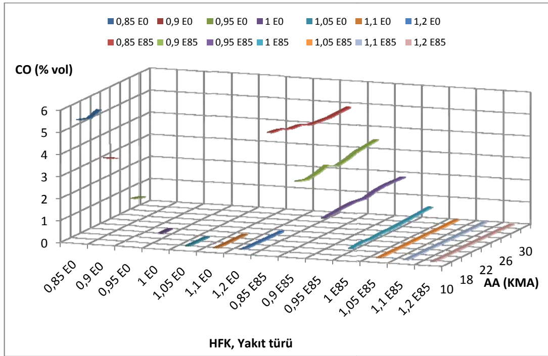
Şekil 5.15. HFK ve ateşleme avansına bağlı olarak CO emisyonlarının değişimi (SO: 11/1, Motor devri: 1500 min -1 , Yakıt Türü: E0 ve E85)
