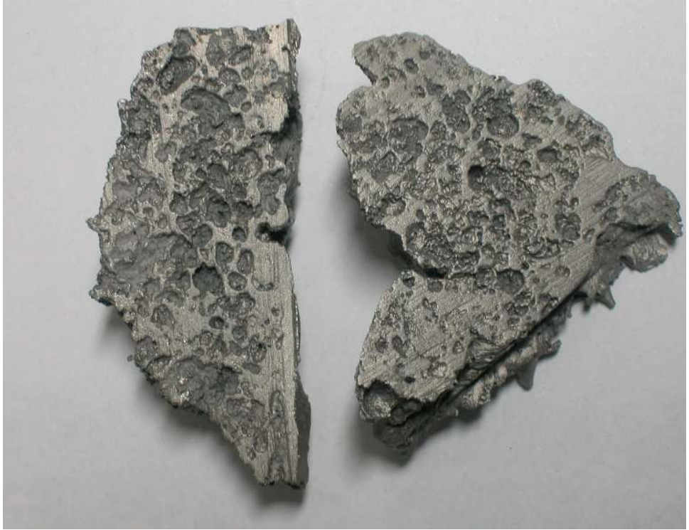
Şekil 5.31 Üretilen köpük metal
