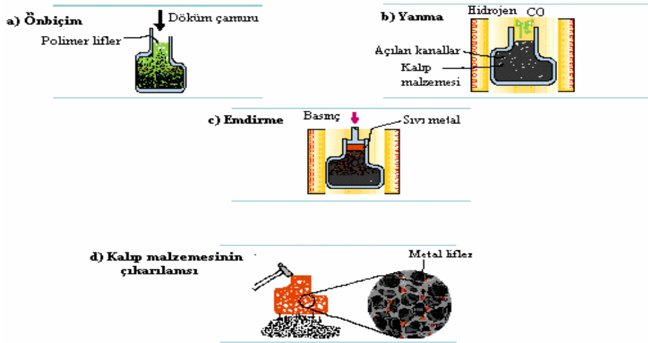
Şekil 2.14 Hassas döküm yöntemi (DUOCEL Yöntemi) ( Amjad, 2000).
