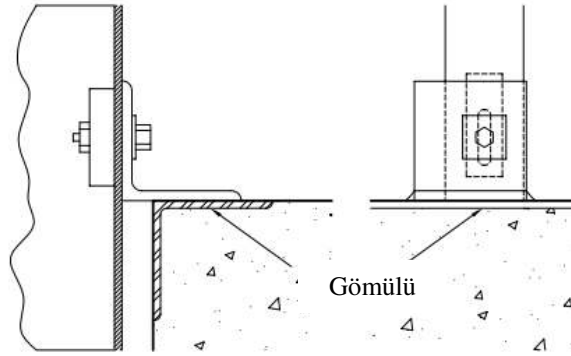
Şekil 3.5. Puyawski bilimsel ve teknoloji parkı binasında kullanılan alüminyum cephe ankraj sistemi (Peter. R. ve Dutton. H. 1995)
