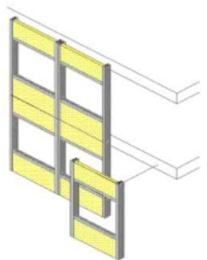
Görsel 2.19. Panel giydirme cephe sisteminin binanın dış cephesinden montajı (Metal Yapı, 2012)
