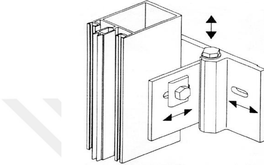
Görsel 2.9. Giydirme cephe alüminyum ankraj elemanı (W.HARTMANN & CO., 2000, Fassaden befestigung Katalog, Hamburg..)
