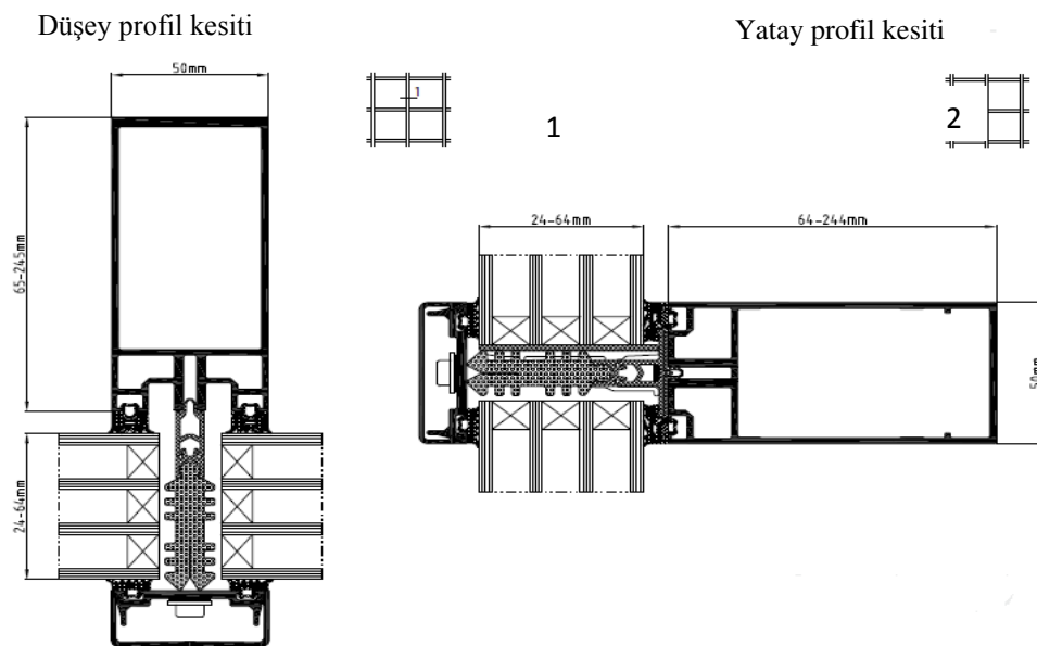
Şekil 3.4. Puyawski Bilim ve Teknoloji Parkı binası alüminyum cephe profili nokta detayları [50]
