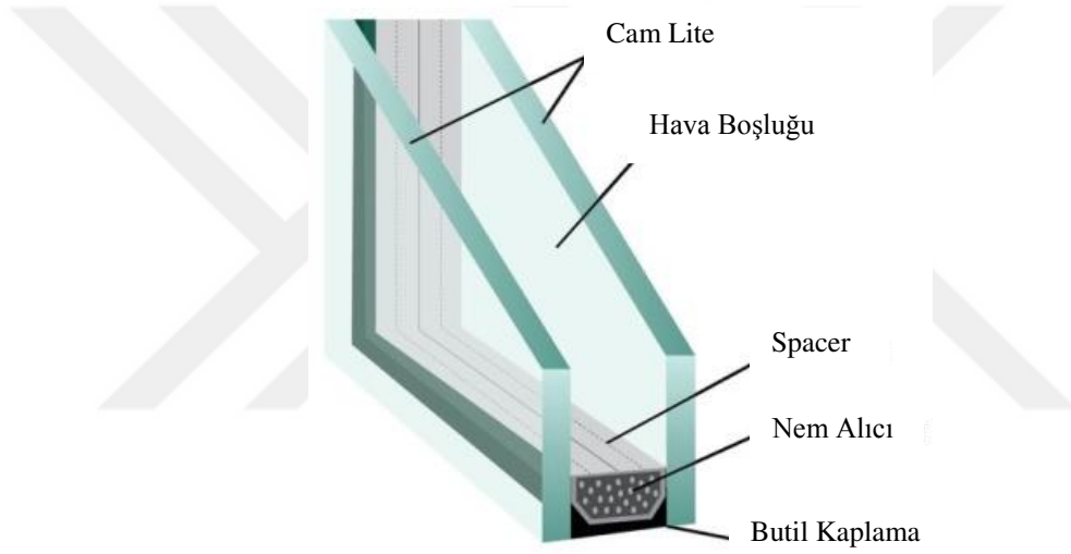
Görsel 2.22. Tipik yalıtımlı cam ünitelerin bir görüntüsü [37]
