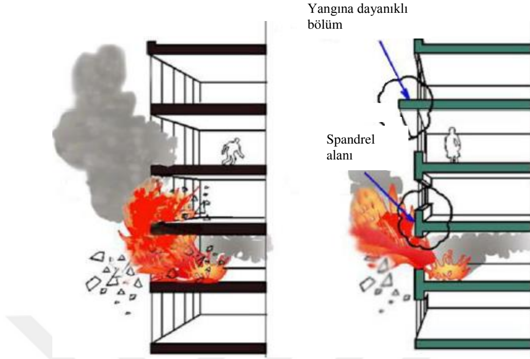
Görsel 2.32. Spandrel alanı olan ve olmayan cephe sistemlerinde yangın iletimi (Kılıç, 2012)
