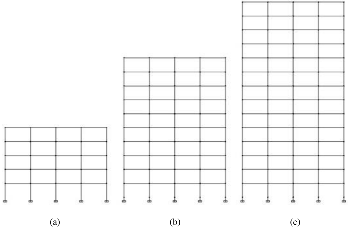
Şekil 2.15. CBP-5 ve CAP-5'e (a), CBP-10 ve CAP-10'a (b), CBP-14 ve CAP-14'e (c) ait B aksı çerçevesi
