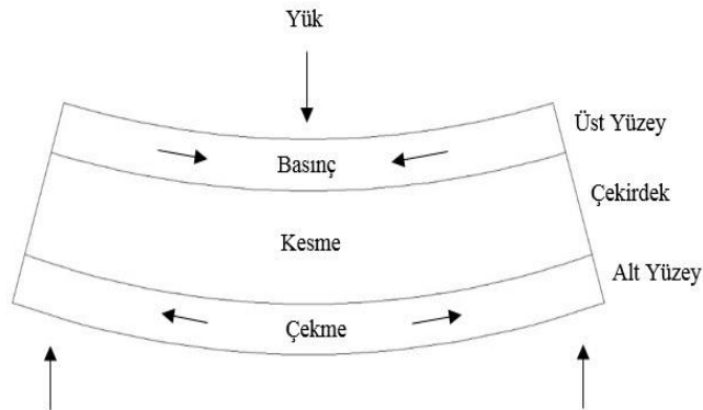
Şekil 1.3. Sandviç kompozitin eğilme durumunda taşıdığı yükler (Kara, 2012)
