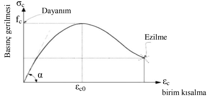
Şekil 1.6. Betonun tipik gerilme-şekildeğiştirme eğrisi
