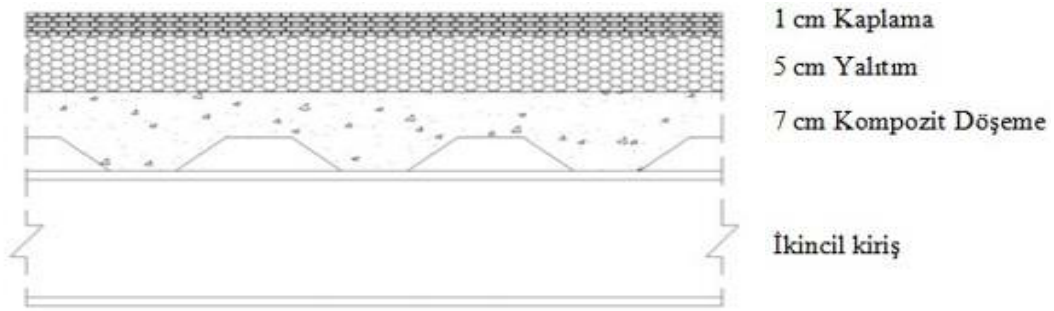
Şekil 2.20. CBP-5, CBP-10 ve CBP-14 modellerine ait çatı katı döşeme kesiti
