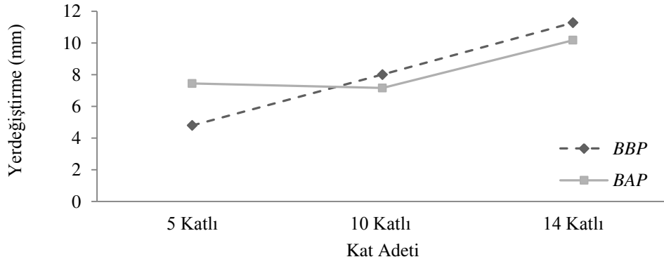
Şekil 3.22. BBP-BAP modelleri için x ve y yönündeki en büyük yerdeğiştirme değerleri (BAP0-5)
