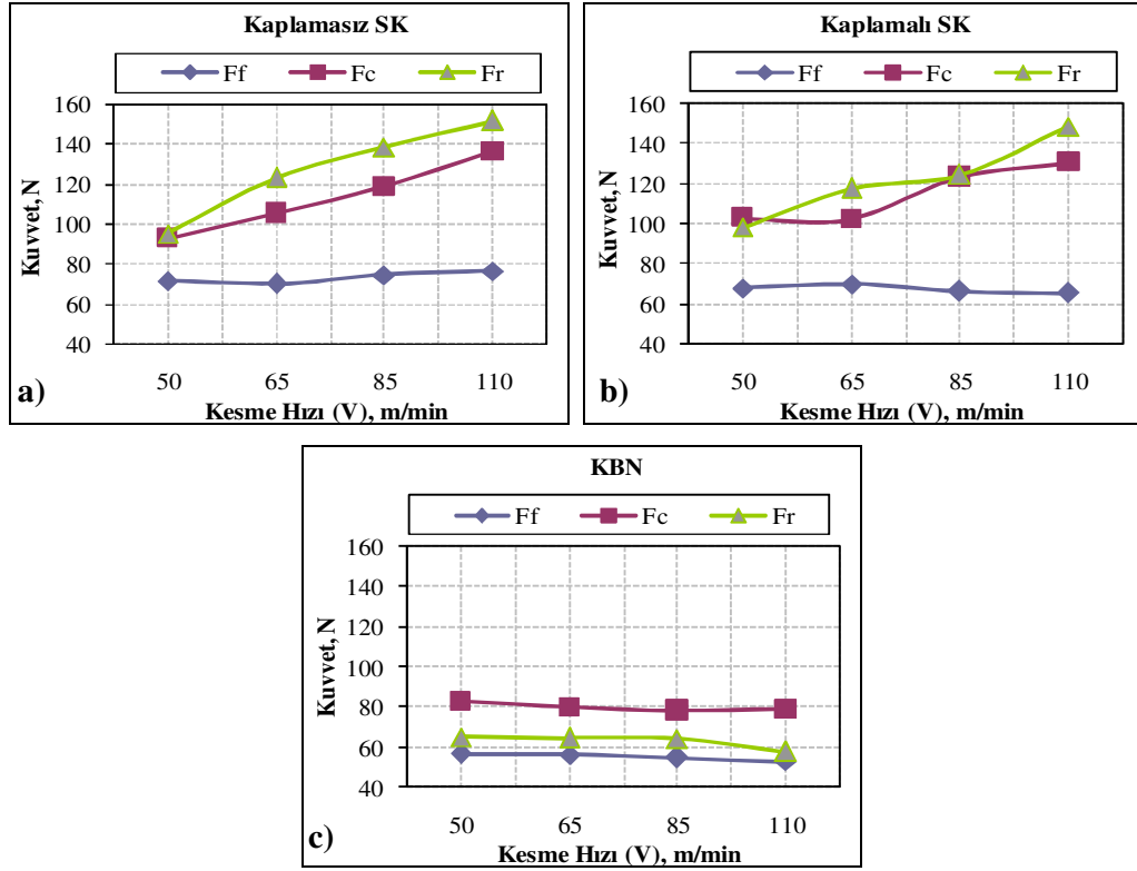
Şekil 7.16. %15 B 4 C takviyeli kompozitin işlenmesinde kesme hızına bağlı olarak ölçülen kesme kuvveti bileşenleri
