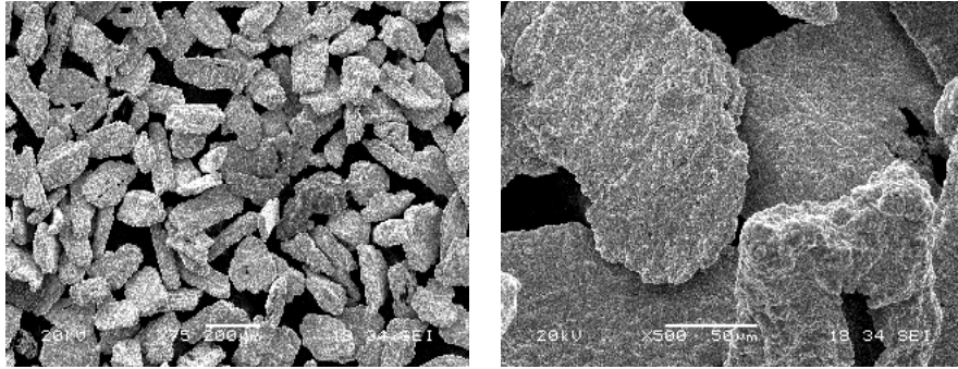
a) b) Resim 7.3. Nikel kaplı grafit parçacıklarının SEM görüntüleri a) x75 büyütme, b) x500 büyütme
