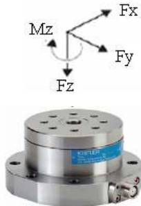
Resim 6.8. Dinamometre ve kuvvet yönleri
