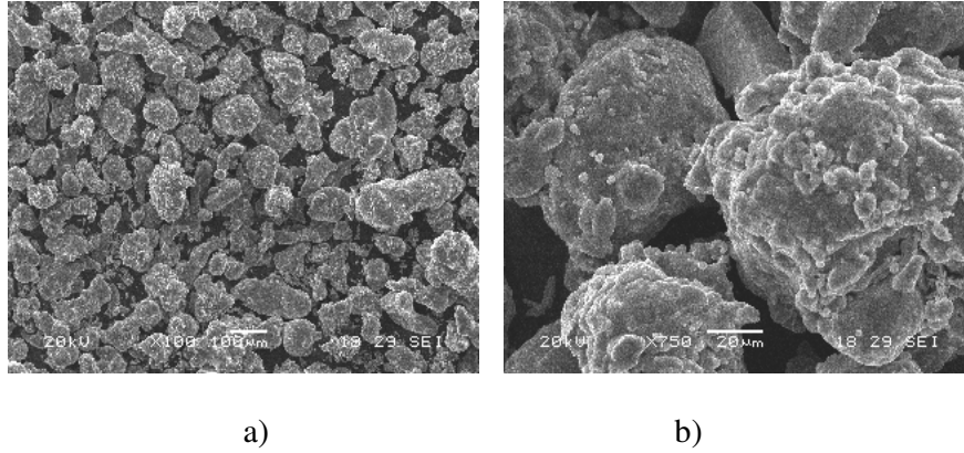
Resim 7.1. Alumix 123 tozunun SEM görüntüleri
