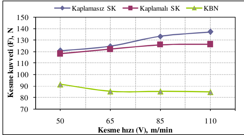
Şekil 7.22. %5 Gr katkılı kompozitin işlenmesinde değişen kesme hızlarında kesme kuvvetinin değişimi
