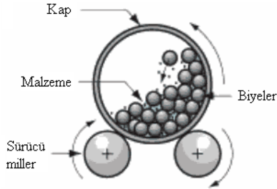
Şekil 4.4. Öğütme yöntemiyle toz üretimi [66]
