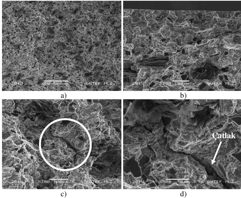
Resim 7.17. %5 Gr katkıli kompozitin kırık yüzey SEM görüntüleri
