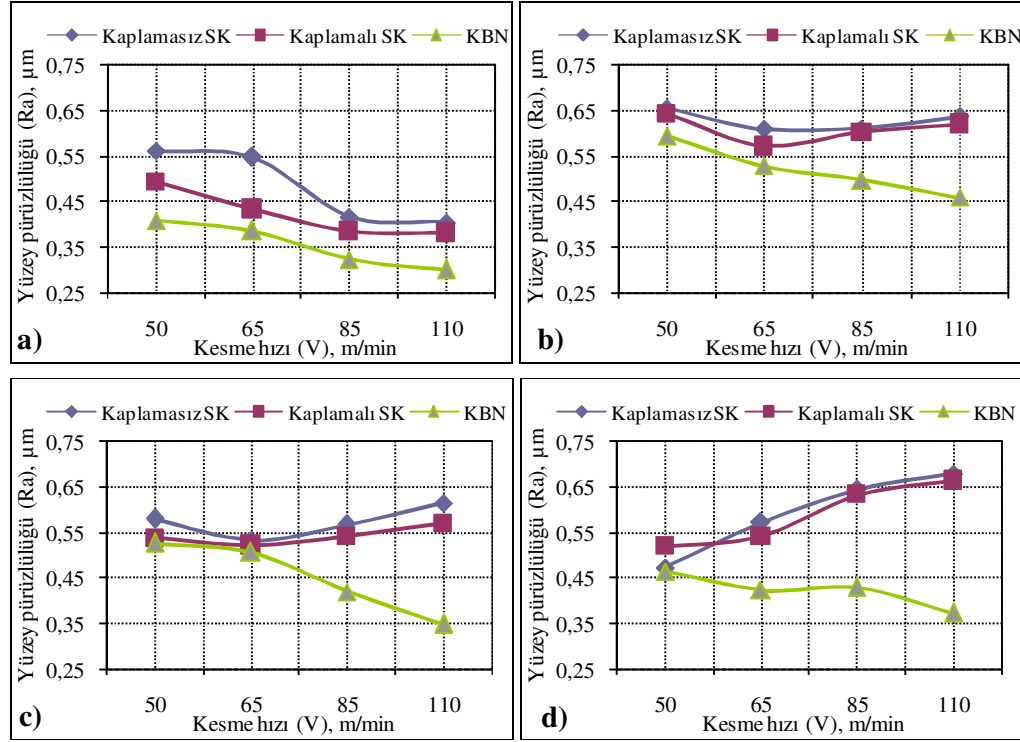
Şekil 7.28. Kesme hızına bağılı olarak B_4C takviyeli kompozitlerin frezelenmesinde ölçülen ortalama yüzey pürüzlülüğü değer grafikleri a) Alumix 123 alaşımı, b) %5 B_4C , c) %10 B_4C , d) %15 B_4C takviyeli
