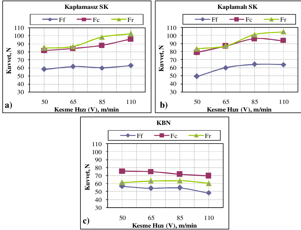
Şekil 7.13. % 10 B 4 C takviyeli kompozitin işlenmesinde kesme hızına bağlı olarak ölçülen kesme kuvveti bileşenleri a)Kaplamaşız SK, b) Kaplamaşlı SK, c) KBN kesici
