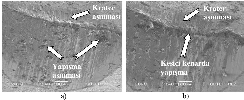
Resim 7.26. %5 Gr katkılı kompozitin kaplamalı kesici takım ile işlenmesi sonrasında çekilen kesici takım SEM fotoğrafları a) Kesme hızı 50 m/min, b) Kesme hızı 110 m/min
