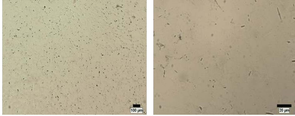
Resim 7.4. Alumix 123 kodlu numunenin mikroyapı grntleri a) x50 bytme, b) x500 bytme
