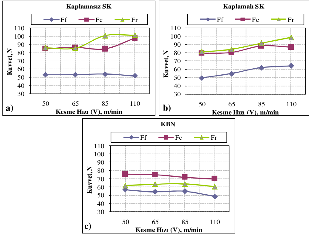
Şekil 7.19. %1 Gr katkılı kompozitin işlenmesinde kesme hızına bağlı olarak ölçülen kesme kuvveti bileşenleri a) Kaplamasız SK, b) Kaplamalı SK, c) KBN kesici
