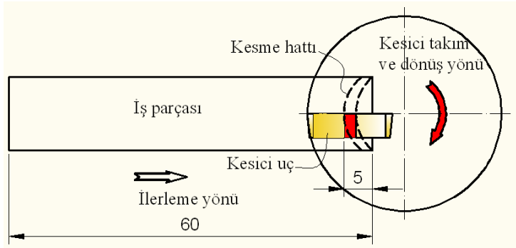
Şekil 6.8. Kararlı bir kesme işleminin başlama mesafesi
