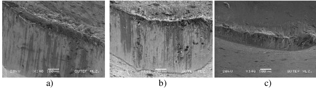
Resim 7.29. %10 B 4 C takviyeli kompozitin 50 m/min kesme hızında işlenmesi sonrasında çekilmiş kesici takım SEM fotoğrafları
