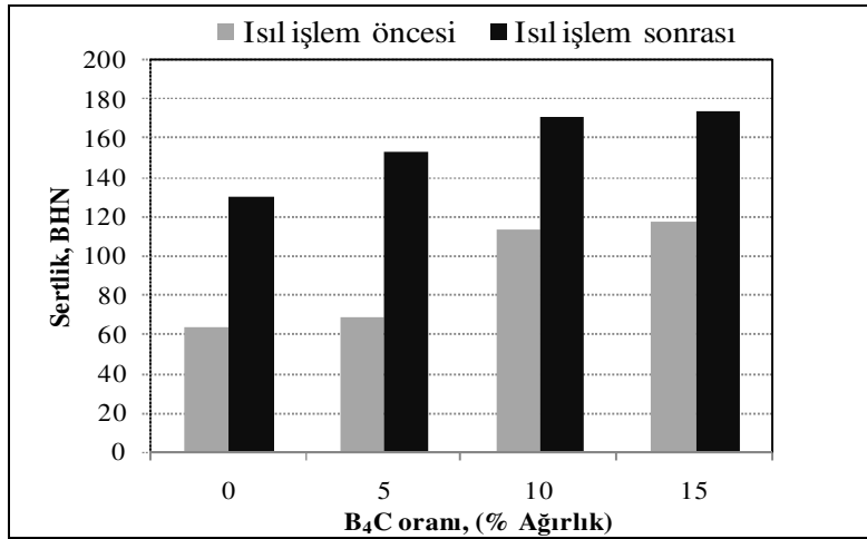
Şekil 7.3. B 4 C miktarına bağlı olarak kompozitlerin sertlik değerleri
