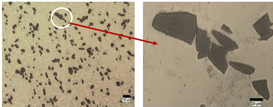
Resim 7.5. %5 \text{B}_4\text{C} kodlu numunenin mikroyapı grntleri a) x50 bytme, b) x500 bytme
