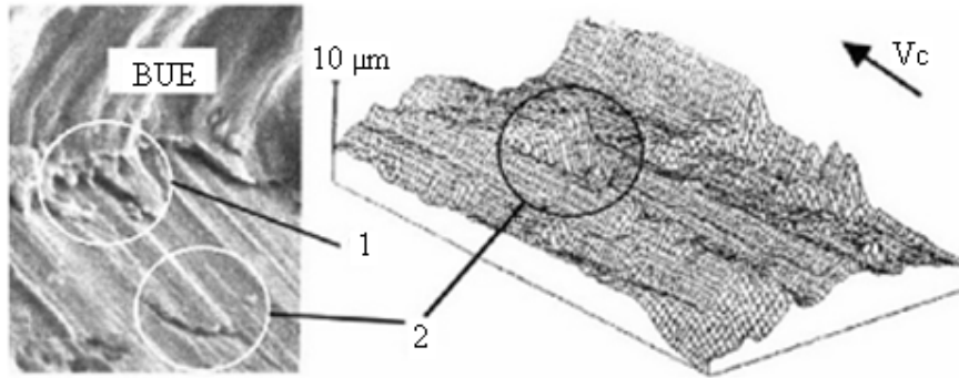
Şekil 5.6. Yığıntı talaş oluşumu ve işlenmiş yüzey üzerinden taşınımı 1) YT'nin kırıldığı yer, 2) İş yüzeyine taşınması [144]
