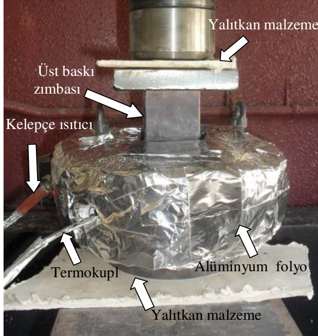
Resim 6.5. Sıcak presleme kalıbı
