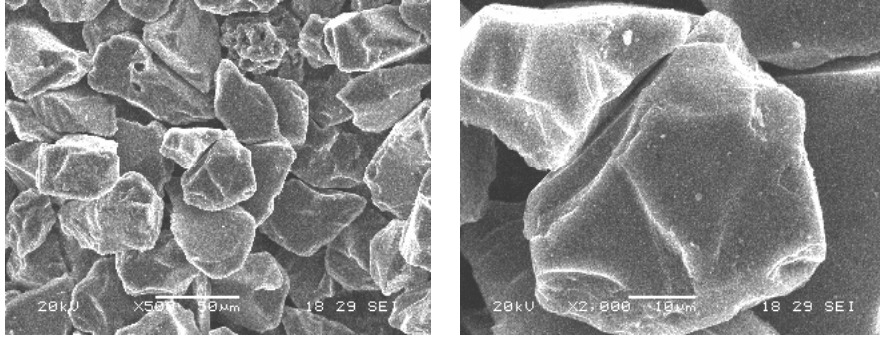
a) b) Resim 7.2. B 4 C parçacıklarının SEM görüntüleri a) x50 büyütme, b) x2000 büyütme
