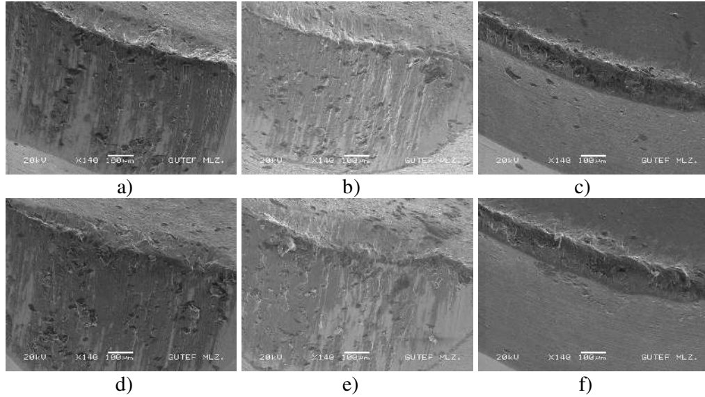
Resim 7.31. %5 Gr katkılı kompozitin 110 m/min kesme hızında işlenmesi sonrasında çekilmiş kesici takım SEM fotoğrafları a)Kapasız SK, b) Kaplamalı SK c) KBN (50 m/min) d) Kapasız SK, e) Kaplamalı SK, f) KBN (110 m/min)
