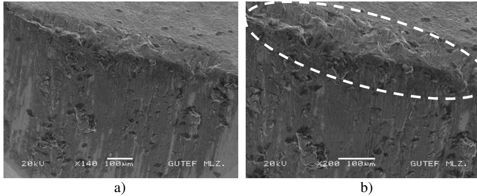
Resim 7.23. %5 Gr katkılı kompozitin kaplamasız SK kesici takımla 110 m/min kesme hızında işlenmesi sonrasında çekilen SEM fotoğrafları a) x140, b) x200 büyütme
