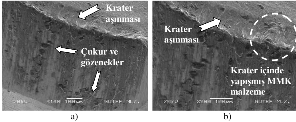
Resim 7.22. %5 Gr katkılı kompozitin kaplamasız SK kesici takımla 50 m/min kesme hızında işlenmesi sonrasında çekilen SEM fotoğrafları a) x140, b) x200 büyütme
