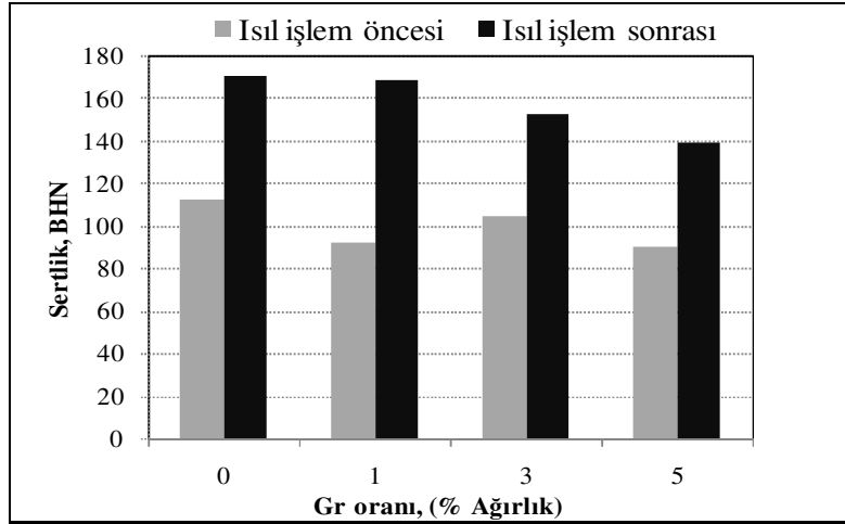
Şekil 7.4. B 4 C+Gr katkılı kompozitlerin Gr miktarına bağlı olarak sertlik değerleri
