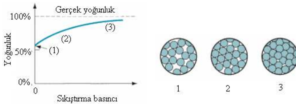
Şekil 4.8. Sıkıştırma sırasında uygulanan basıncın etkisi 1 doldurmadan sonraki gevşek tozlar; 2 yeniden paketleme; ve 3 parçacıkların deformasyonu; ve tozların yoğunluğunun, basınca bağlı olarak değişimi [66]
