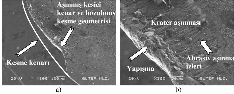
Resim 7.24. %10 B_4C takviyeli kompozitin kaplamalı SK kesici takım ile 50 m/min kesme hızında işlenmesi sonrasında çekilen SEM fotoğrafları a) x100, b) x300 büyütme
