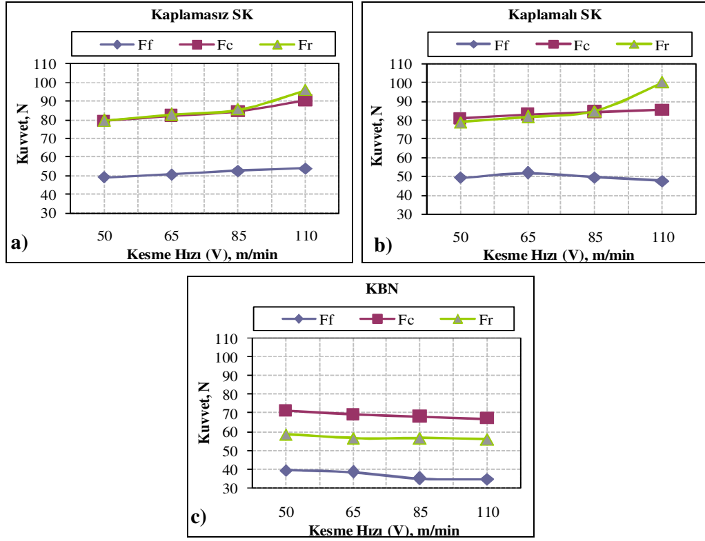
Şekil 7.21. %3 Gr katkıli kompozitin işlenmesinde kesme hızına bağlı olarak ölçülen kesme kuvveti bileşenleri
