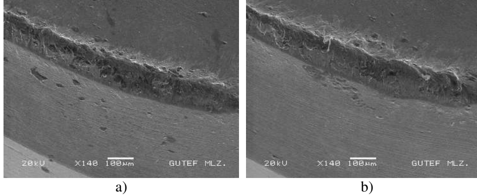
Resim 7.28. %5 Gr katkılı kompozitin KBN kesici takımla işlenmesi sonrasında çekilen kesici takım SEM fotoğrafları
