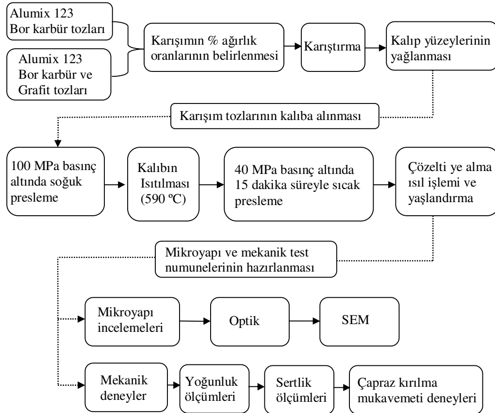
Şekil 6.1. Kompozit numunelerin üretiminde deneysel çalışmanın akış şeması
