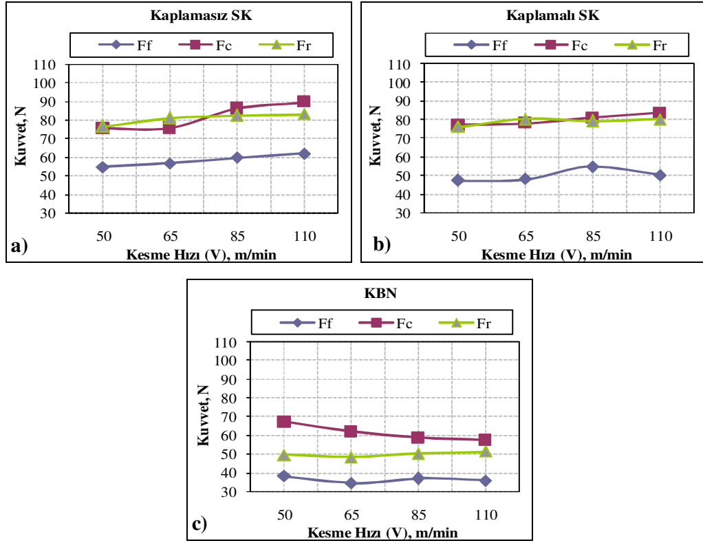
Şekil 7.23. %5 Gr katkılı kompozitin işlenmesinde kesme hızına bağlı olarak ölçülen kesme kuvveti bileşenleri a) Kaplamasız SK, b) Kaplamalı SK, c) KBN kesici
