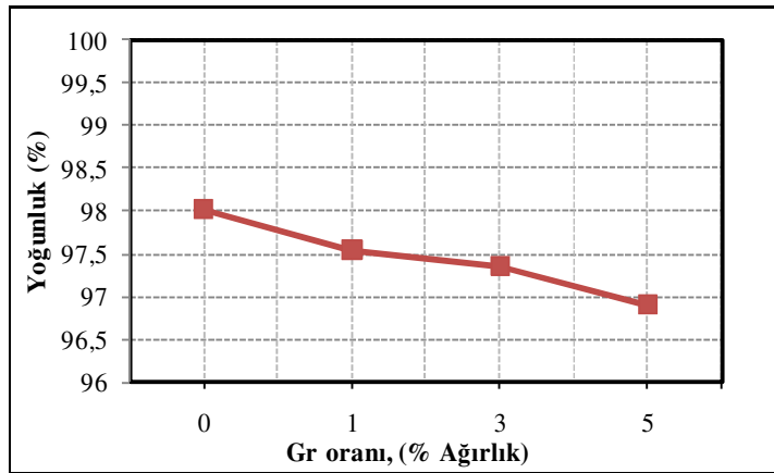
Şekil 7.2. B 4 C+Gr katkılı kompozitlerin Gr miktarına bağlı olarak yoğunluk değerleri
