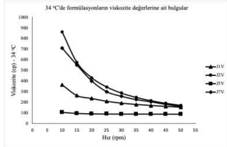
Şekil 4.11 J1V, J2V, J5V ve J7V nolu formülasyonlarında MS miktarının 20 °C ve 34 °C'de viskozite grafikleri
