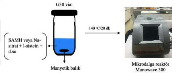
Şekil 3.1 Formülasyonların mikrodalga reaktör cihazında hazırlanmasının şematik gösterimi ve mikrodalga reaktör cihazı
