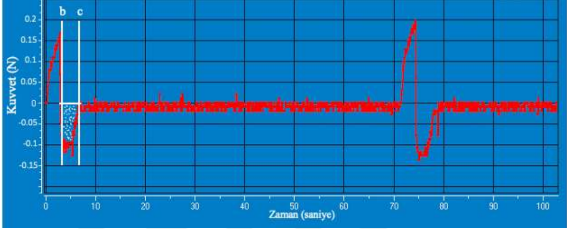
Şekil 3.9 Jellerin adezifliğini gösteren kuvvet-zaman eğrisi
