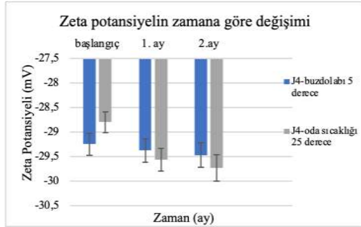
Şekil 4.30 J4 formülasyonlarına ait zaman bağlı zeta potansiyel değişim grafiği
