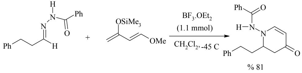
N -(4-okso-2-fenetil-3,4-dihidropiridin-1(2H)-il)benzamid
