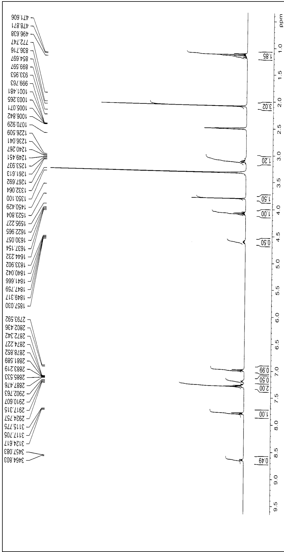
Şekil 2. Bileşik (1)'in ^1\text{H} NMR spektrumu ( \text{DMSO}-d_6 )
