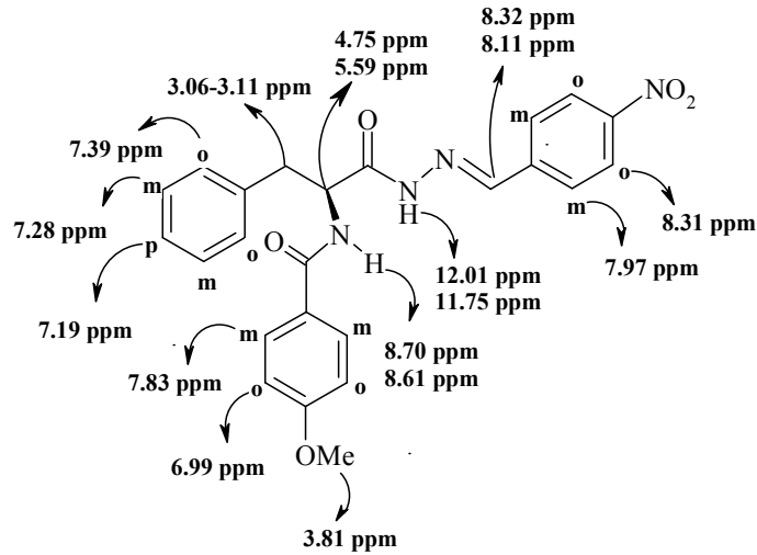
Şekil 37. Bileşik ( 3b )'nin 1 H NMR kimyasal kayma değerleri
