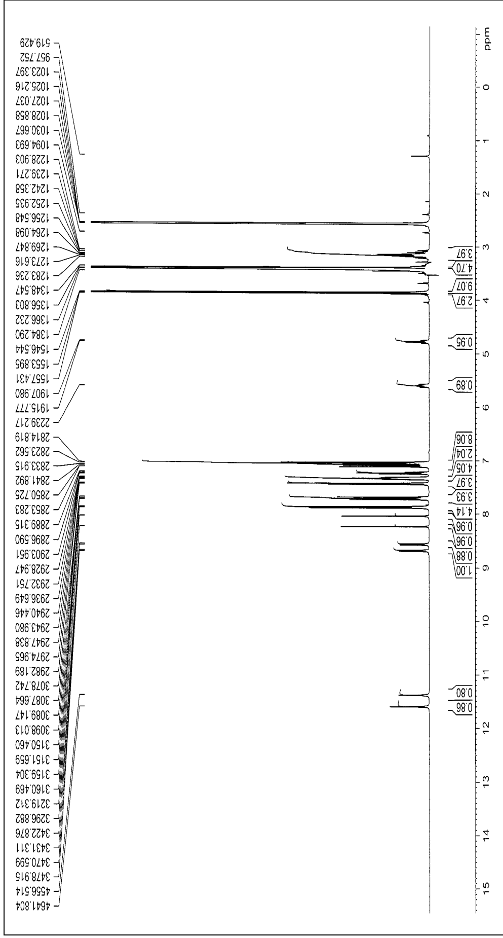
Şekil 12. Bileşik (3d) 'nin ^1\text{H} NMR spektrumu ( \text{DMSO}-d_6 )
