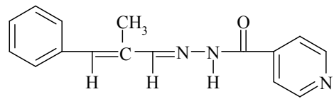
N' -(2-metil-3-fenilaliliden)izonikotinohidrazit
