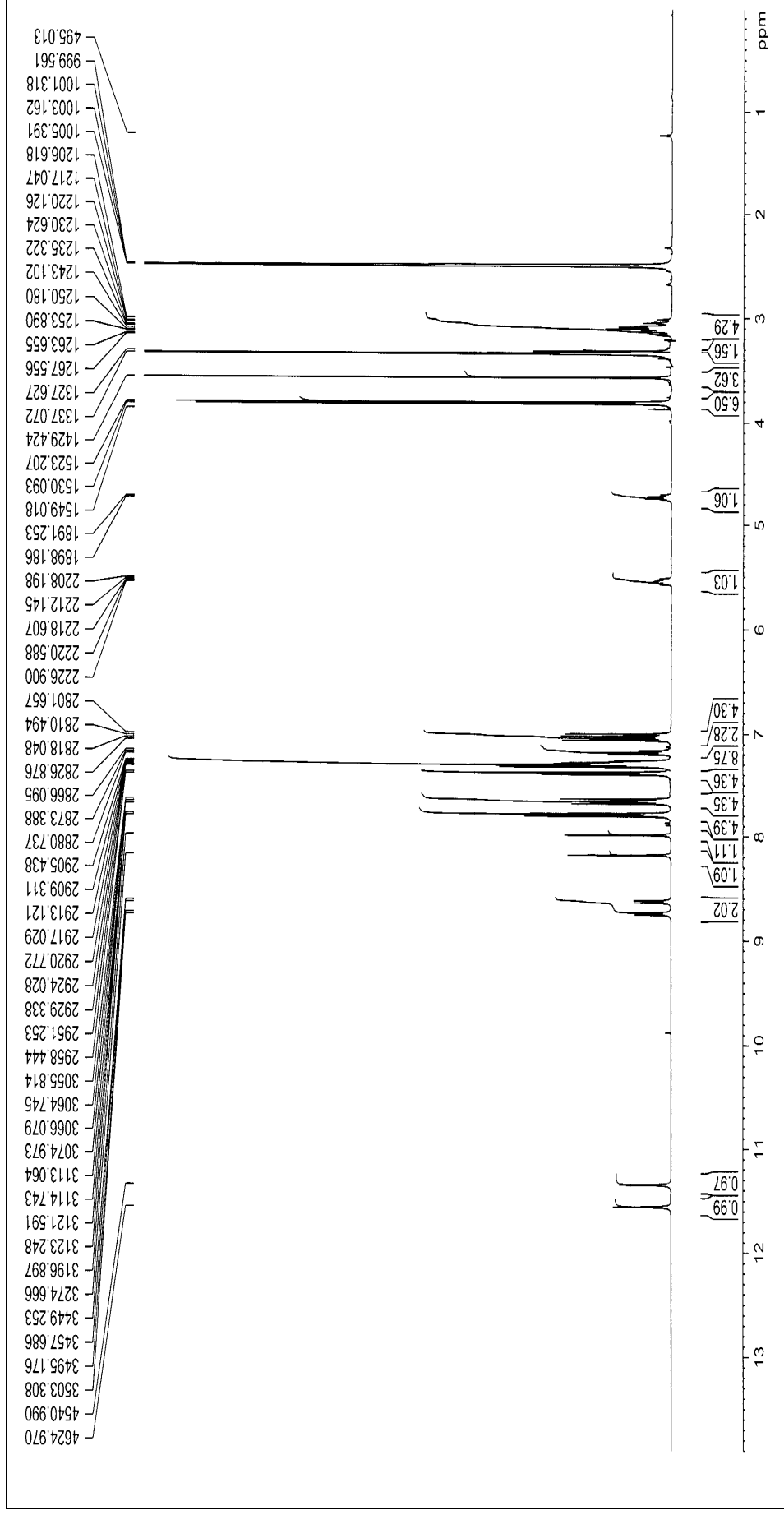
Şekil 24. Bileşik (6d)'nin ^1\text{H} NMR spektrumu ( \text{DMSO}-d_6 )
