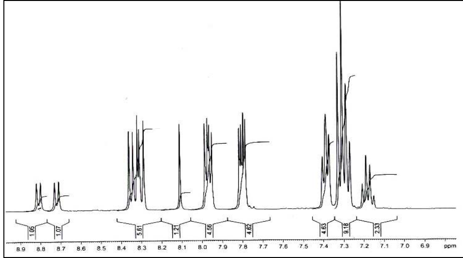
Şekil 40. Bileşik (6b)'in N=CH ve aromatik bölgesine ait ^1\text{H} NMR spektrumu
