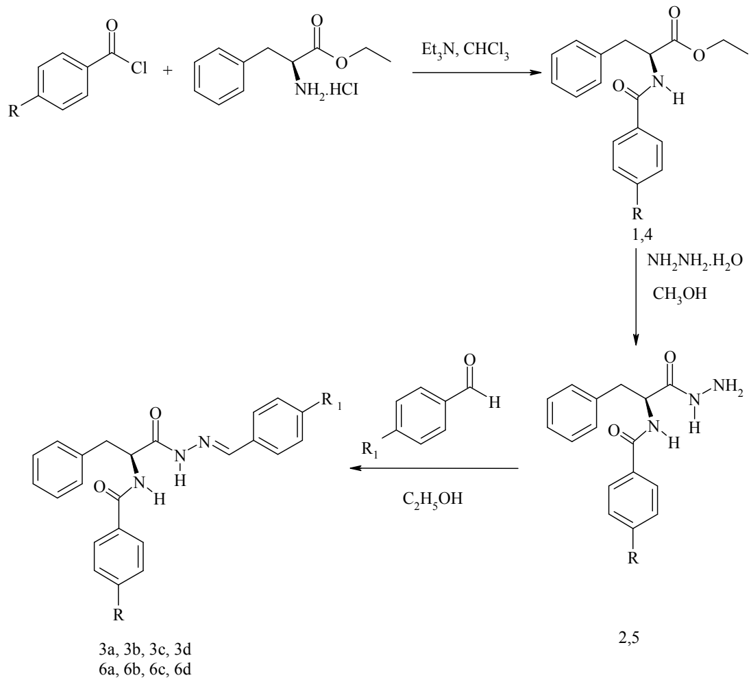
Şema 3. Hidrazon türevlerinin genel sentez şeması
