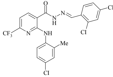
(E)-N'(2,6-Diklorobenziliden)-2-(4-kloro-2-metilfenilamino)-6-(triflorometil)nikotinohidrazit
