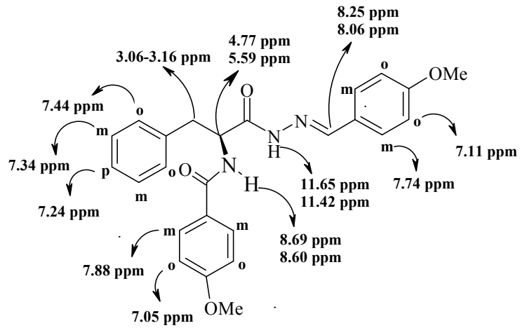
Şekil 45. Bileşik ( 3d )’in ^1\text{H} NMR kimyasal kayma değerleri
