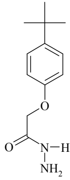
2-(4- tert -bütilfenoksi)asetohidrazit
