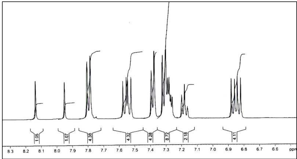
Şekil 36. Bileşik (6a)'in \text{N}=\text{CH} ve aromatik bölgesine ait ^1\text{H} NMR spektrumu
