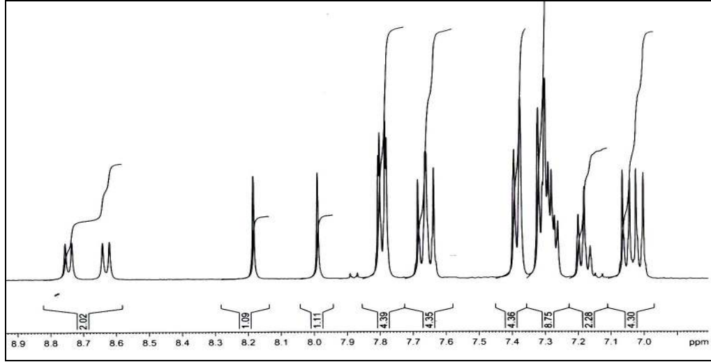
Şekil 48. Bileşik (6d)'in N=CH ve aromatik bölgesine ait ^1\text{H} NMR spektrumu
