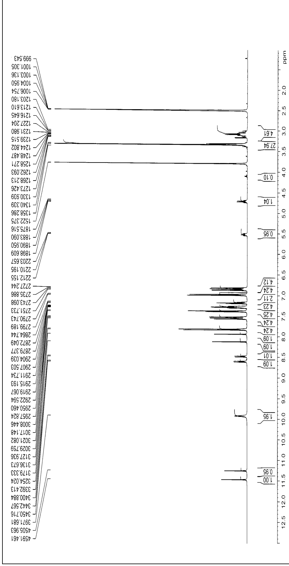
Şekiln 6. Bileşik (3a) 'nın 1 H NMR spektrumu (DMSO- d 6 )
