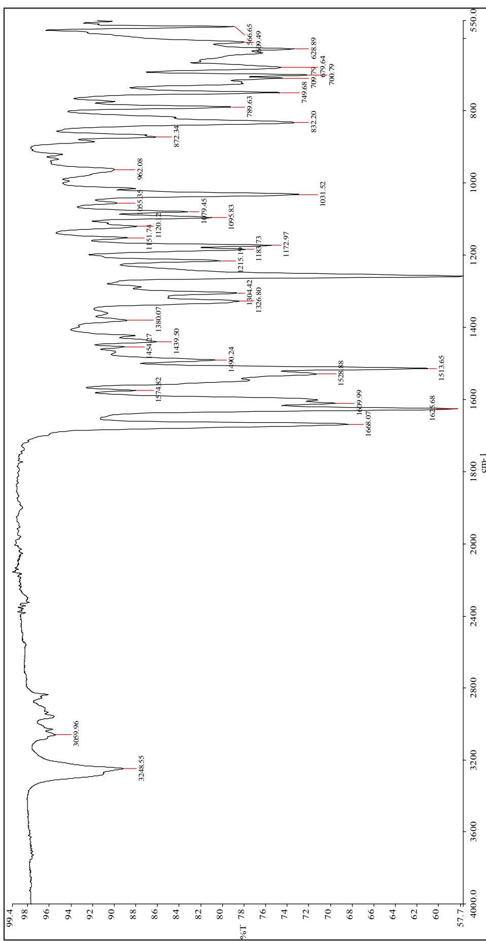
Şekil 23. Bileşik (6d)'nin IR spektrumu
