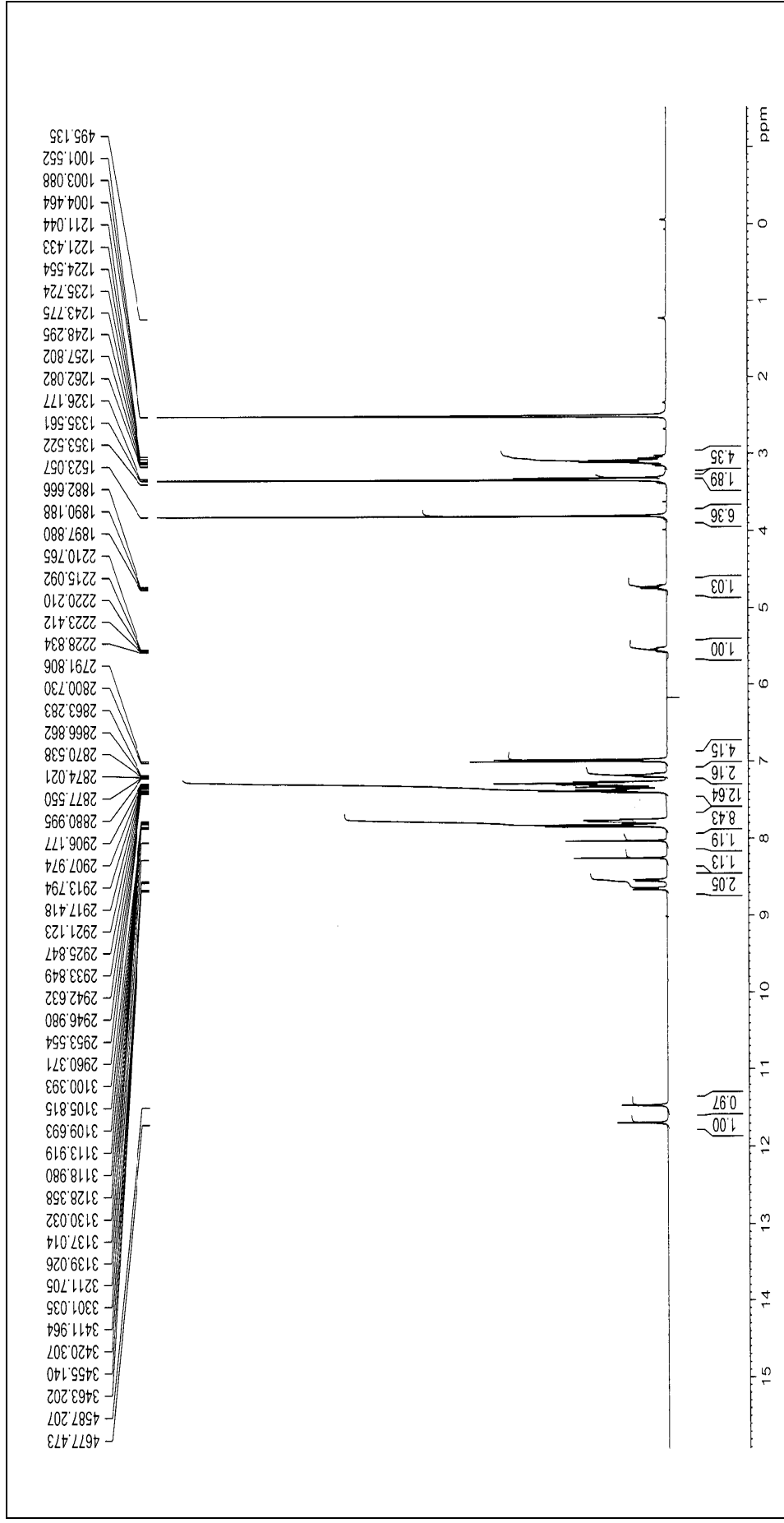
Şekil 10. Bileşik (3c) 'nin 1 H NMR spektrumu (DMSO- d 6 )
