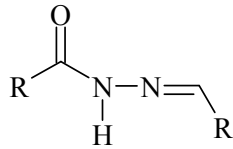
Hidrazon
