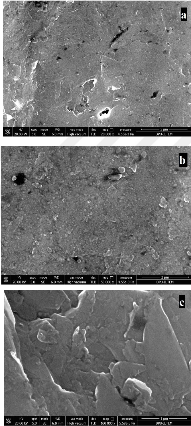
Şekil 4.18. P2AB kaplanmış PGE nin (a) 20000x (b)50000x (c)100000x ölçeklendirilmiş FESEM görüntüleri.
