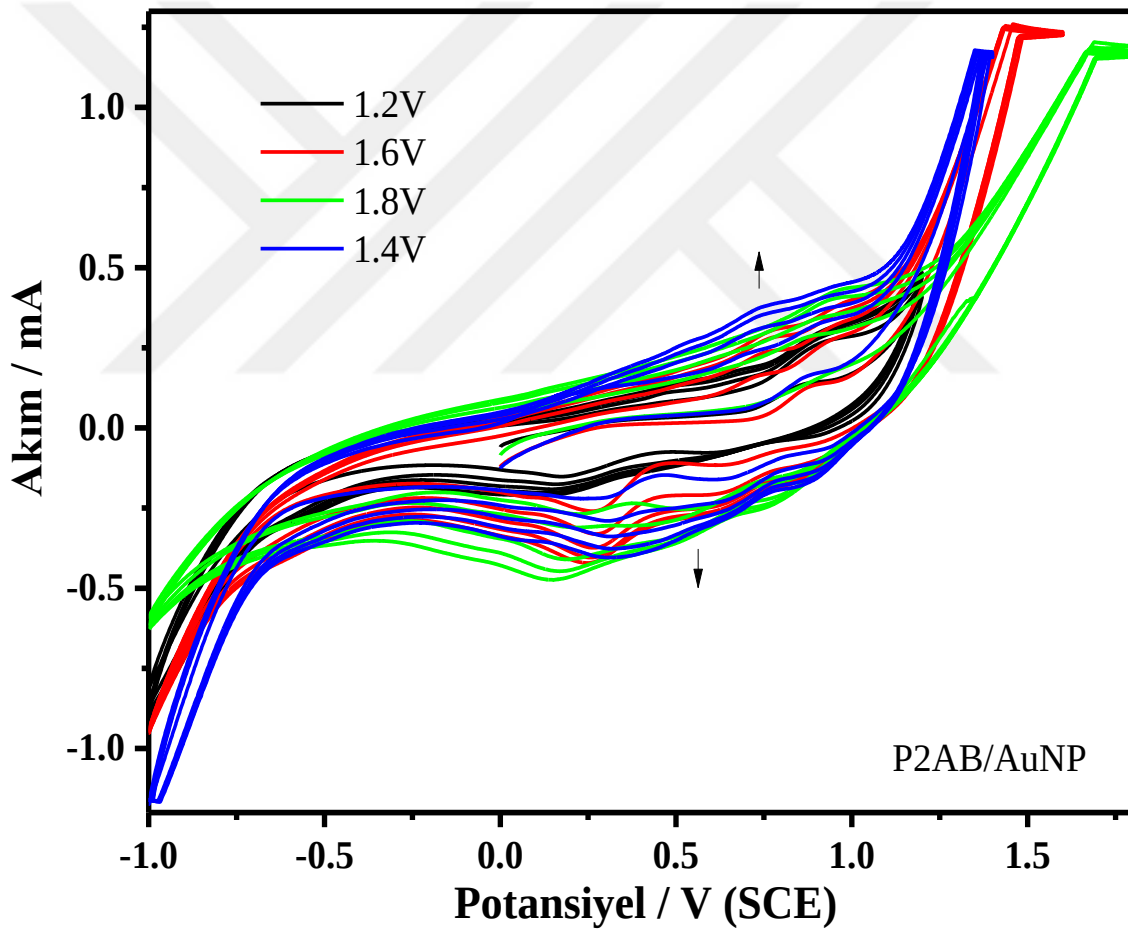
Şekil 4.11. 100 mM 2AB / 100 mM TBAP / 75 mM HClO 4 ve 10 mM HAuCl 4 içeren asetonitril çözeltisinde 5 döngü tarama yapılarak biriktirilen P2AB filmlerinin sentezi esnasında alınan çok döngülü voltamogramları, ( v = 100 \text{ mV s}^{-1} ).
