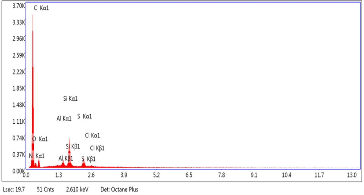
Şekil 4.19. Nötral P2AB kaplanmış PGE'nin EDX spektrumu.
