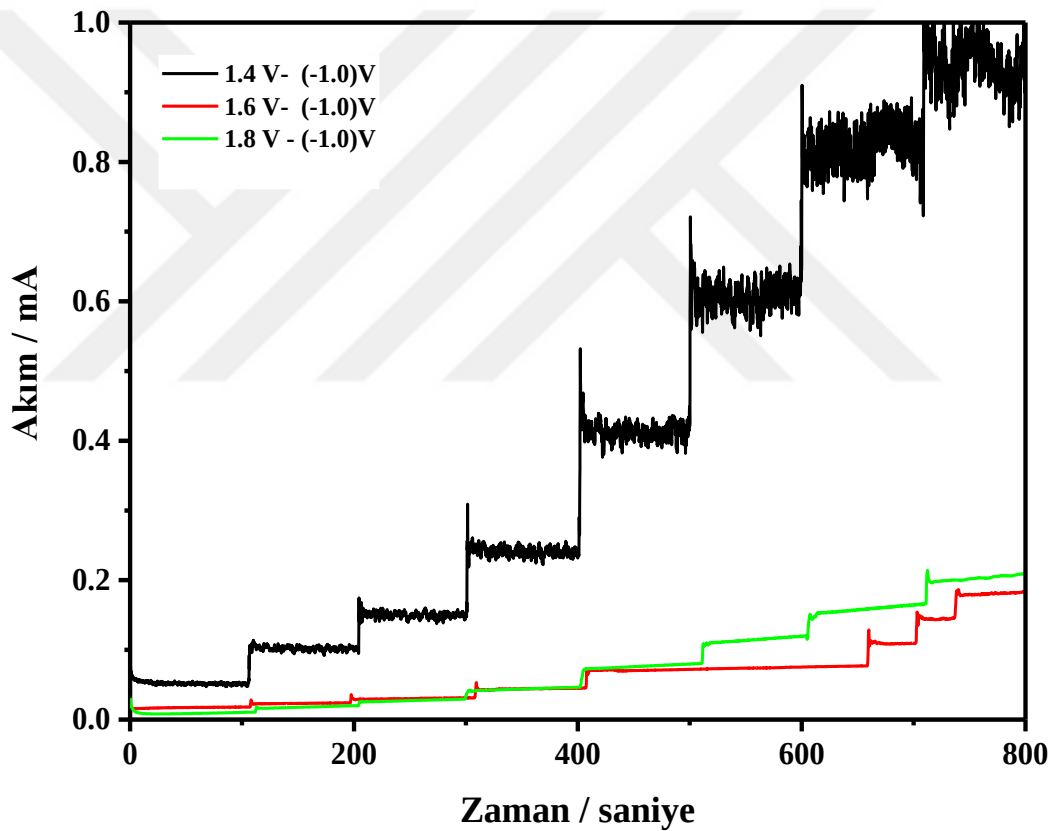
Şekil 4.30. -1.0 V ile 1.4 V, 1.6 V, 1.8 V arasında değişen potansiyel aralıklarında dönüşümlü voltametri kullanılarak PGE yüzeyine biriktirilen P2AB/AuNP filminin giderek artan derişimde (0.5 mM-10 mM) H_2O_2 ilavesiyle elde edilen amperometrik i-t eğrileri.
