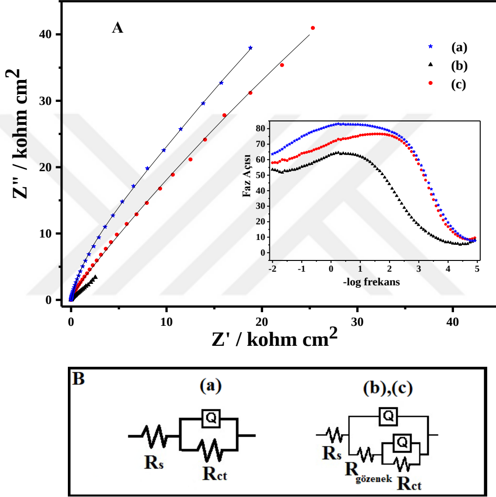
Şekil 4.24. (a) Çıplak (b) P2AB ve (c) P2AB/AuNP kaplanmış elektrotların A) açık devre potansiyellerinde pH 6.5 fostat tampon çözeltisinde alınan Nyquist eğrileri ve eşdeğer devre modelinden türetilen teorik eğriler (içindeki şekil faz açısı-log(frekans) (Bode eğrileri)) B) empedans davranışına uygun olan eşdeğer devre modelleri.
