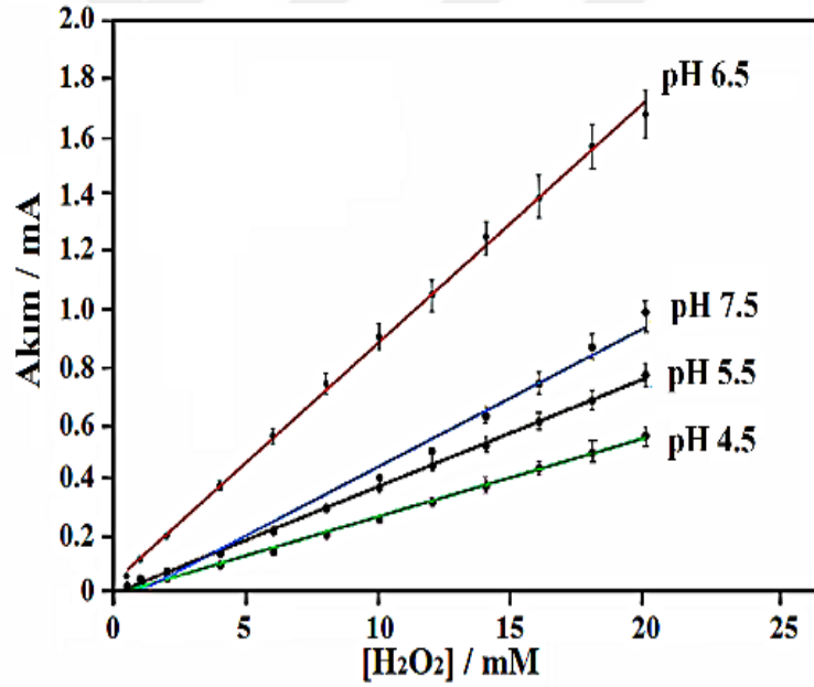
Şekil 4.29. -0.1 V ile 1.4 V arasında 5 döngü potansiyel taraması ile biriktirilen P2AB/AuNP kaplanmış PGE üzerinden -0.8 V da 0.5–20 mM arasında giderek artan derişimlerde H_2O_2 ekleyerek elde edilen amperometrik i-t eğrilerindeki akım deęerlerinin fosfat tamponunun pH sına göre deęişimi.
