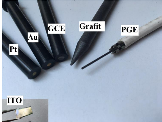
 ekil 3.3. Kullanılan  eřitli  alışma elektrotları
