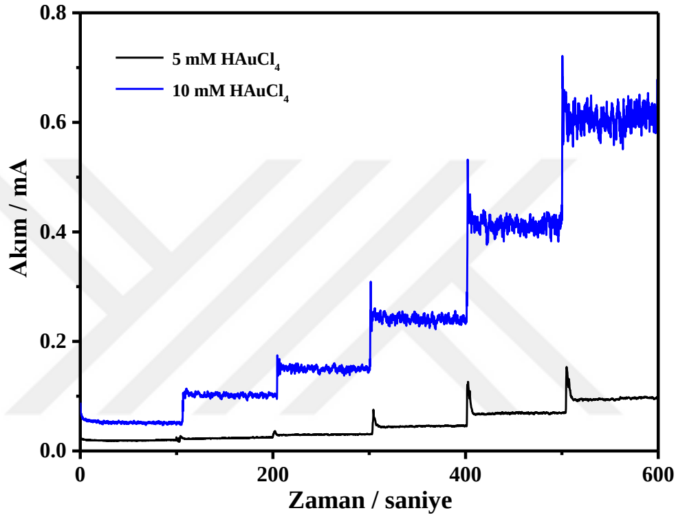
Şekil 4.31. 100 mM 2AB, 100 mM TBAP, 75 mM HClO_4 ile 5 mM ve 10 mM HAuCl_4 varlığındaki polimerizasyon çözeltileri kullanılarak hazırlanan polimer filmlerin -0.8 V da filminin giderek artan derişimde 0.5 mM–6.0 mM H_2O_2 ilavesiyle elde edilen amperometrik i-t eğrileri.
