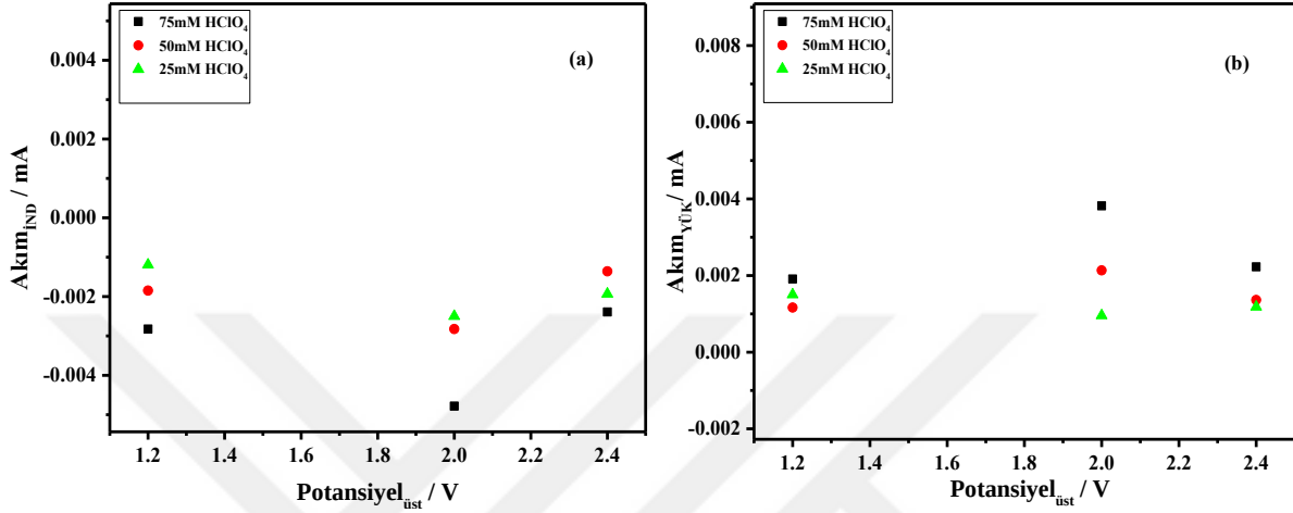
Şekil 4.2. 50 mM 2AB / 100 mM TBAP ile 25, 50, 75 mM HClO 4 içeren çözeltilerin -1.0 V ile 1.2, 2.0, 2.4 V potansiyel aralıklarında biriktirilen P2AB filmlerinin boş çözelti voltamogramları kullanılarak oluşturulan üst potansiyele karşı (a) akım ind ve (b) akım yük grafikleri.
