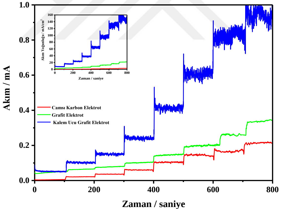
Şekil 4.28. Kalem ucu grafit elektrot, camısı karbon elektrot ve grafit elektrot yüzeyine kaplanmış P2AB/AuNP filmi ile modifiye edilmiş elektrotlar üzerinde pH 6.5 PBS, -0.8 V da
