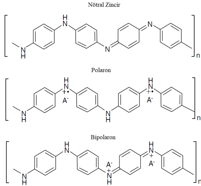
Şekil 2.2. PPy ve PANI nin nötral, polaron ve bipolaron moleküler yapıları [45].
