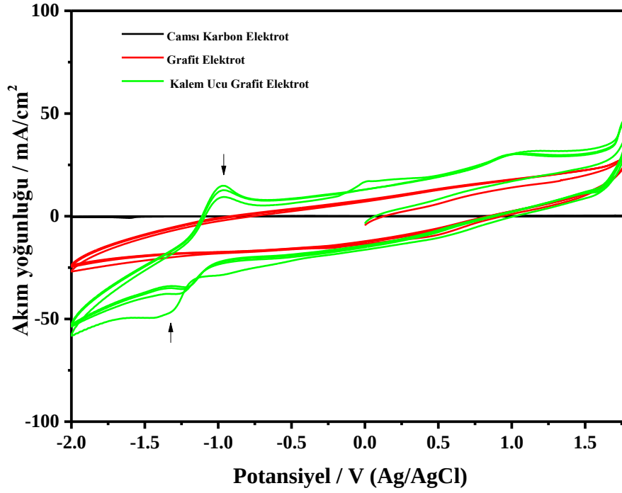
Şekil 4.9. Şekil 4.8 de verilen P2AB kaplanmış elektrotların boş çözeltide, -1.0 ile 1.9 V arasında alınan çok döngülü voltamogramları ( v = 100 \text{ mV s}^{-1} ).
