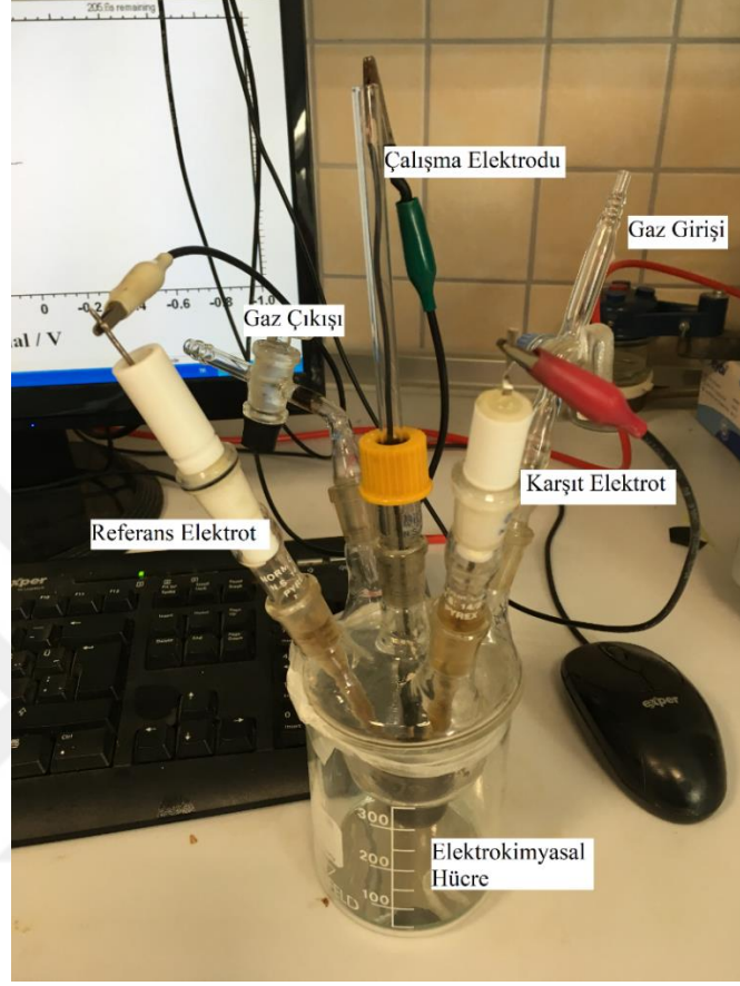
 ekil 3.2.    elektrotlu elektrokimyasal h cre.
