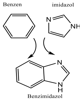
Şekil 2.4. Benzimidazolün molekül yapısı.
