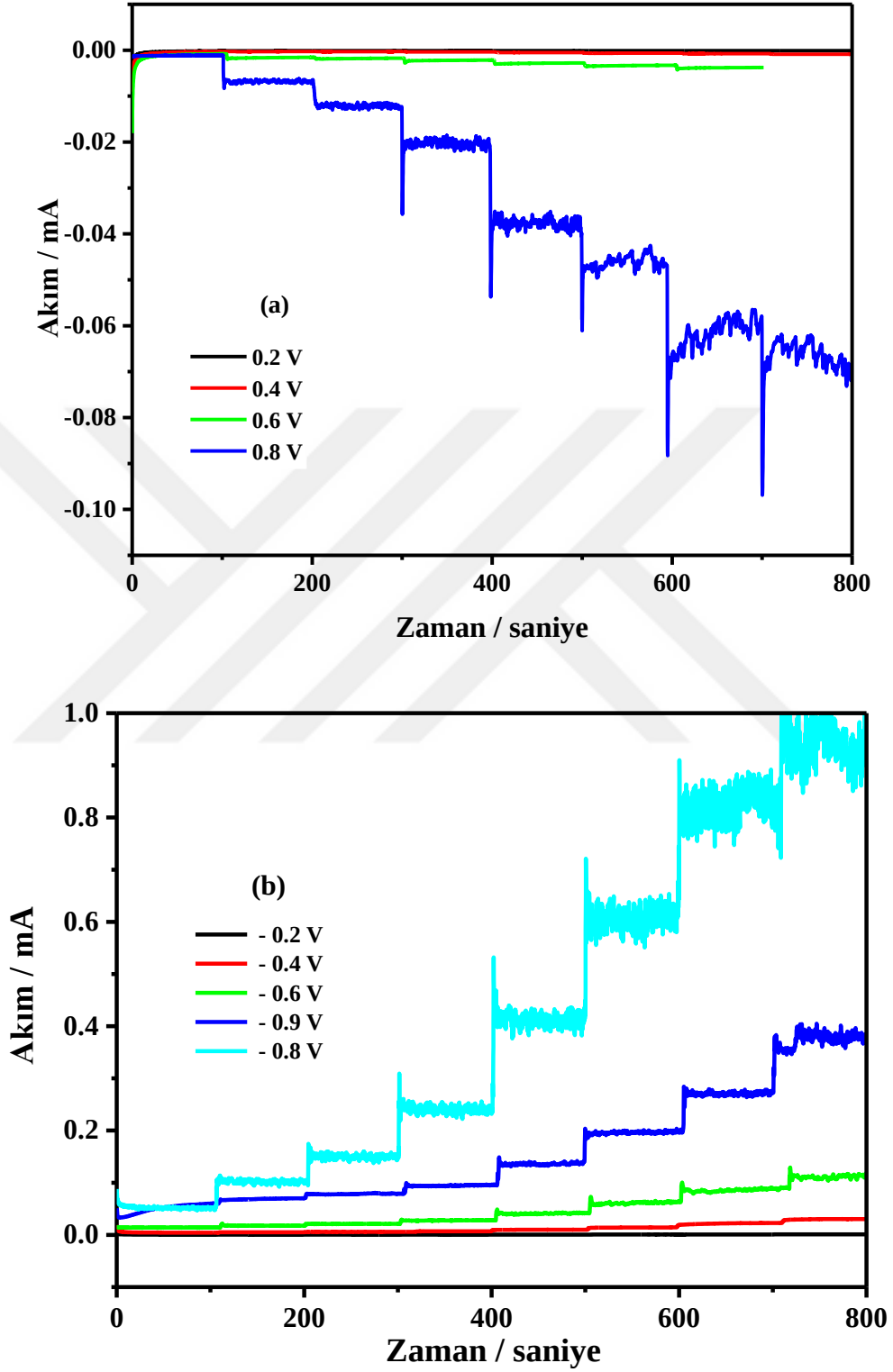
Şekil 4.32. Optimum koşullarda P2AB/2AB kaplanmış kalem ucu grafit elektrodu ile 100 mM pH 6.5 PBS de a) 0.2 V, 0.4 V, 0.6 V, 0.8 V ve (b) -0.2 V, -0.4 V, -0.6 V, -0.8 V, -0.9 V da giderek artan derişimlerde H 2 O 2 ilavesiyle elde edilen amperometrik i-t eğrileri.
