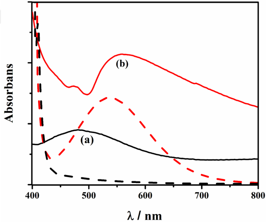
Şekil 4.13. 100 mM 2AB / 75 mM HClO 4 / 100 mM TBAP ve (a) H 2 AuCl 4 içermeyen (b) 10 mM H 2 AuCl 4 içeren polimerizasyon çözeltilerinden sırasıyla P2AB ve P2AB/AuNP kaplanmış ITO elektrotların UV-Vis spektrumları (Karşılaştırmak için Şekil 4.10 de sunulan polimerizasyon çözeltilerine ait spektrumlar aynı renk ve kesik çizgili gösterimle verilmiştir.)
