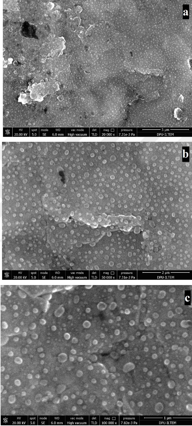
Şekil 4.17. Nötral P2AB kaplanmış PGE nin (a) 20000x (b) 50000x (c) 100000x ölçeklendirilmiş FESEM görüntüleri.
