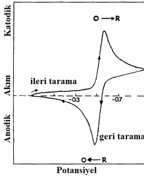
Şekil 2.8. Dönüşümlü voltametri tipik voltamogram gösterimi [157]
