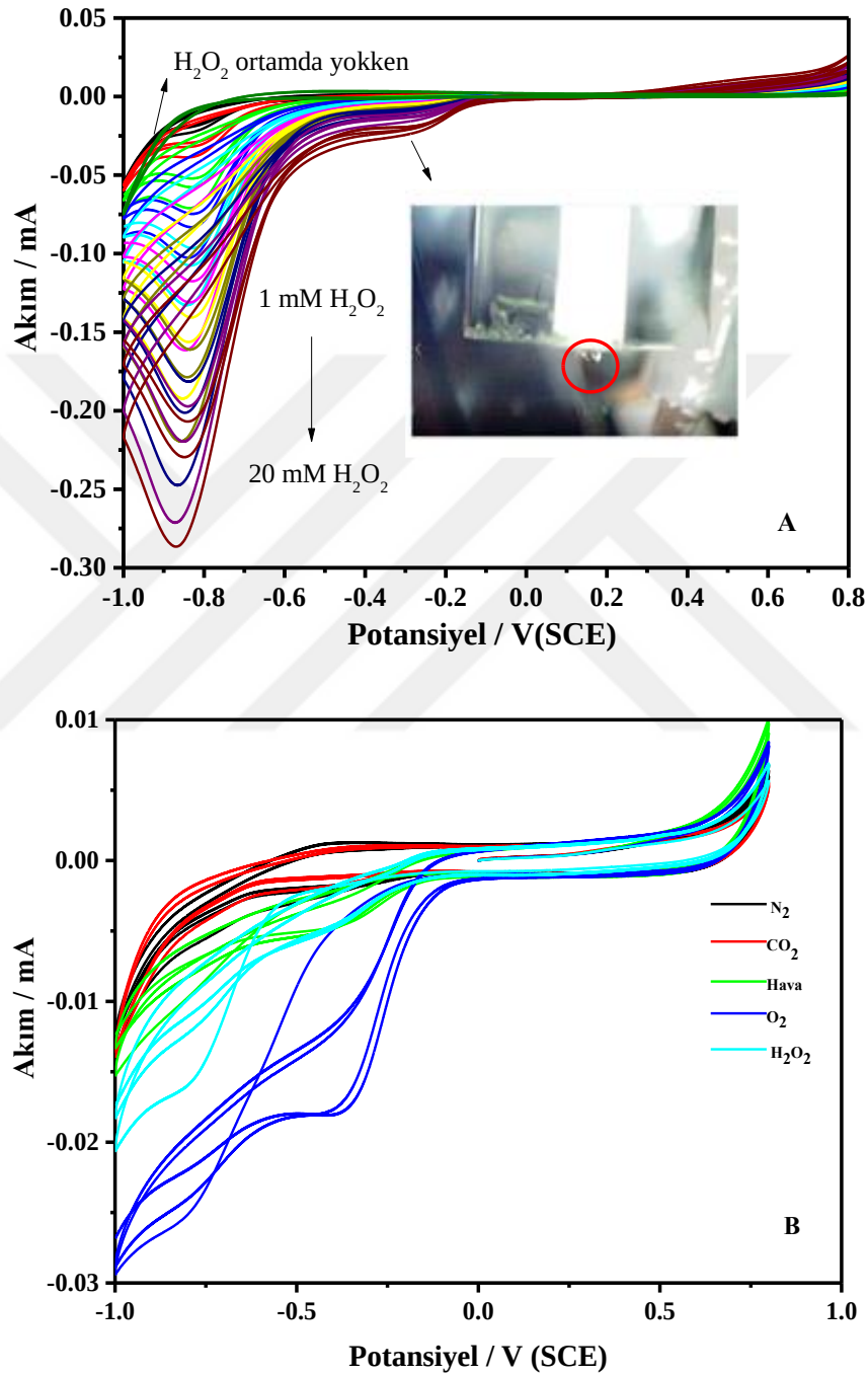
Şekil 4.26. Çıplak Altın elektrodun pH 6.5 PBS de A) 1.0 mM dan 20.0 mM a kadar artan derişimde \text{H}_2\text{O}_2 eklendikten sonra alınan B) 5 dk \text{N}_2 , \text{CO}_2 , kuru hava ve \text{O}_2 geçirildikten sonra ve azot atmosferinde 1.0 mM \text{H}_2\text{O}_2 ilave edildikten sonra alınan voltamogramlar, ( v=100 \text{ mVs}^{-1} )
