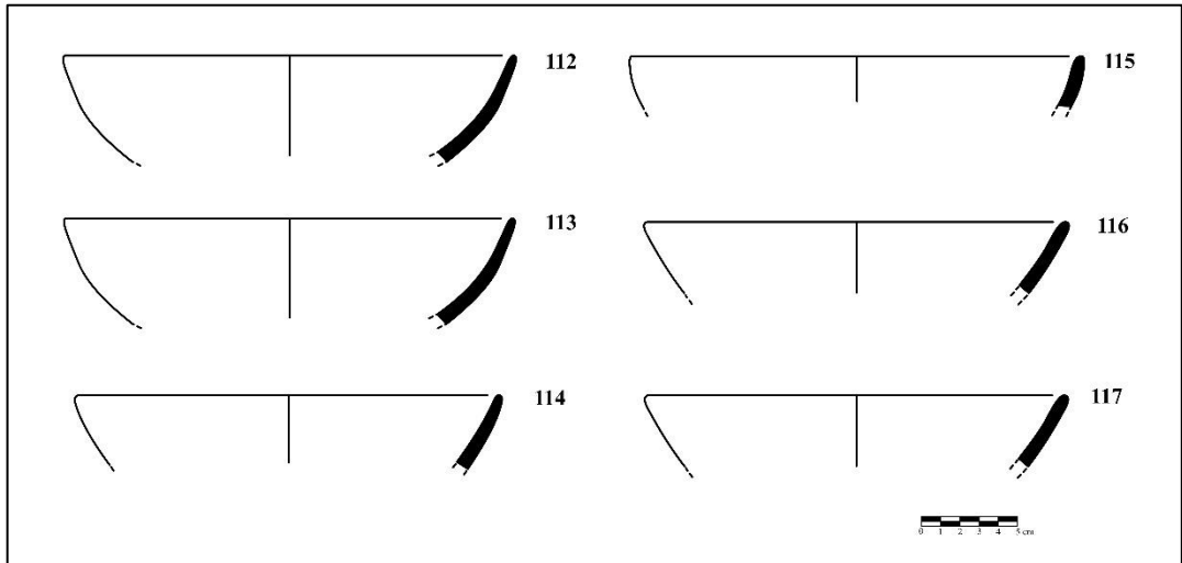
Çizim 15. Turkuaz renk sırlı, yarı-küresel gövdeli çanak örnekleri (Kat.112-117)
