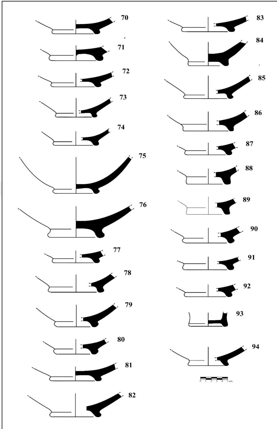
Çizim 13. Yeşil renk sırlı yüksek halka kaide örnekleri (Kat.70-94)
