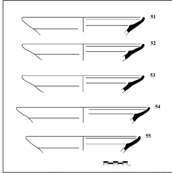
Çizim 10. Yeşil renk sırlı, yayvan gövdeli, dışa çekik ve iç bükey ağız profilli tabak örnekleri (Kat.51-55)
