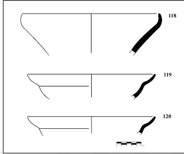
Çizim 16. Turkuaz renk sırlı, yarı-küresel gövdeli iç bükey ağız profilili (Kat.118) ve yarı-küresel gövdeli dışa çekik ağız profilili çanak örnekleri (Kat.119-120)
