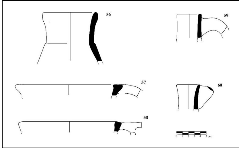
Çizim 11. Yeşil renk sırlı sıvı kaplarına ait örnekler (Kat.56-60)
