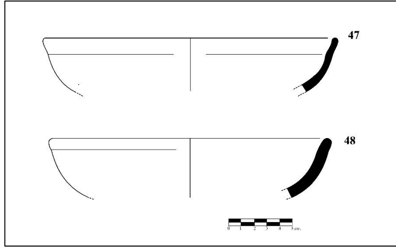
Çizim 8. Yeşil renk sırlı, yayvan gövdeli çanak örnekleri (Kat.47-48)
