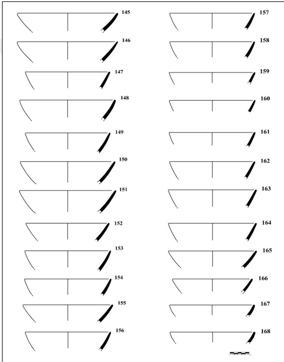
Çizim 20. Çok renkli sgraffito bezemeli, yarı-küresel gövdeli çanak örnekleri (Kat.145-168)
