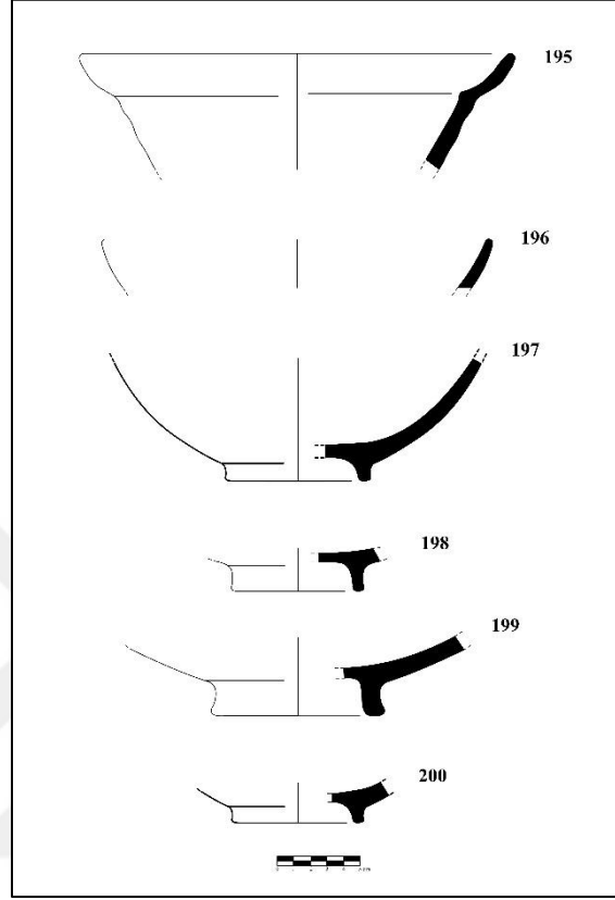
Çizim 26. Milet İşi yarı-küresel gövdeli ağız ve yüksek halka kaide örnekleri (Kat.195-200)
