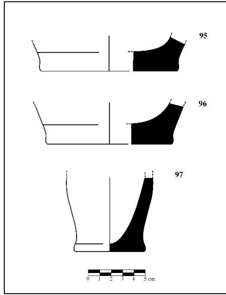
Çizim 14. Yeşil renk sırlı düz dipli kaide örnekleri (Kat.95-97)
