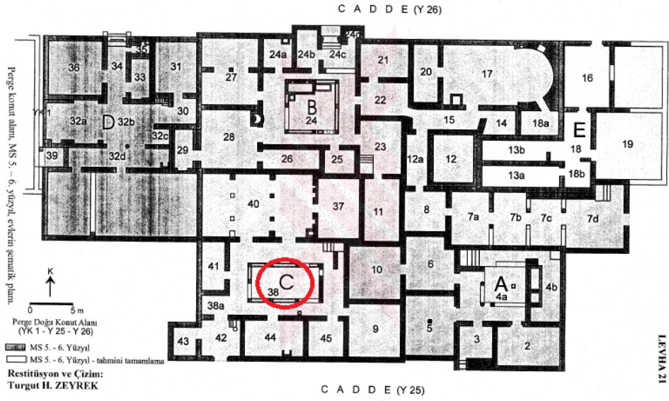
Şekil 69: Perge C Evi Planı (zeyrek, 2002.).
