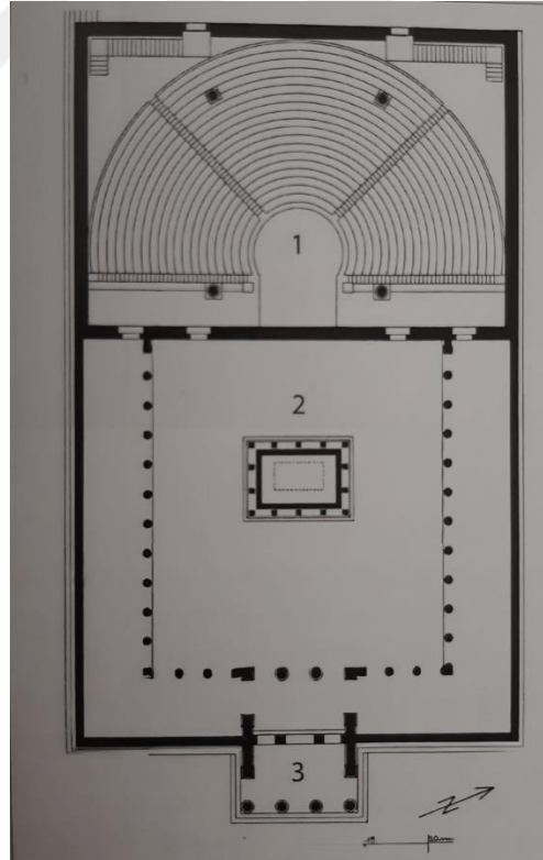
Şekil 28: Miletos Bouleuterion'u (Emme, 2016: 91.).
