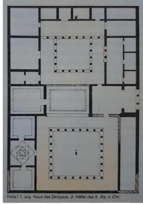
Şekil 13: Pella Kenti Peristyl'li Konut Planı ( Emme, 2013: 238.).
