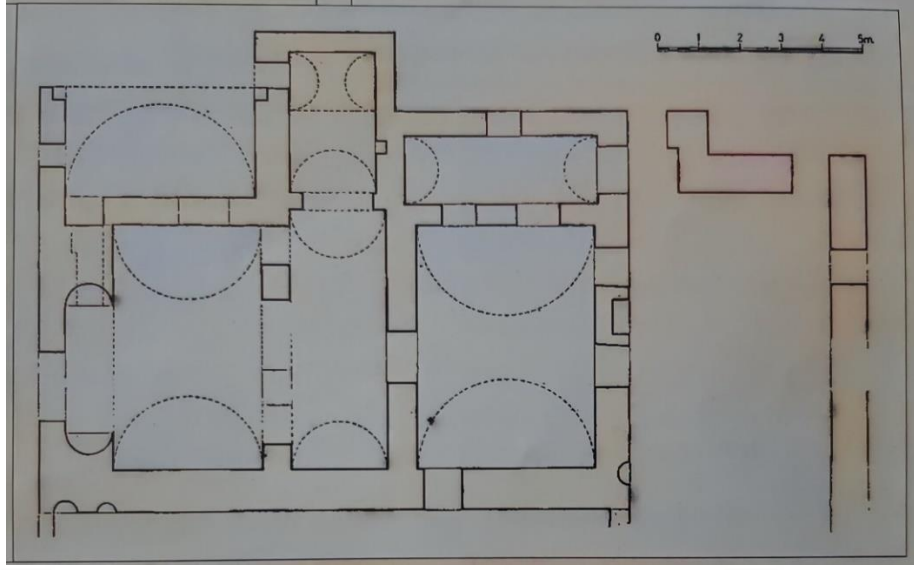
Şekil 79: Side de Bir Bizans Evi Planı (Eyice, 1999: 209.).
