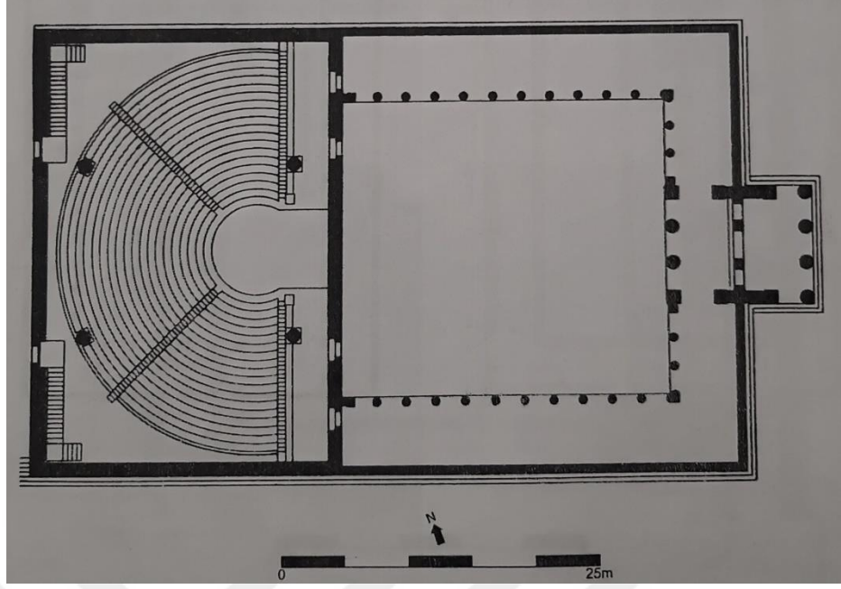
Şekil 11: Miletos Bouleuterion'u Planı (Emme, 2013: 460.).
