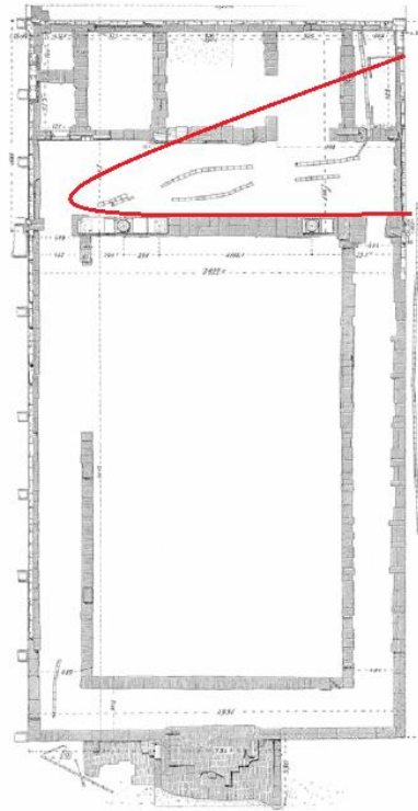
Şekil 26: Miletos Hellenistik Peristyl Su Boruları Sistemi (emme, 2013: 461.).
