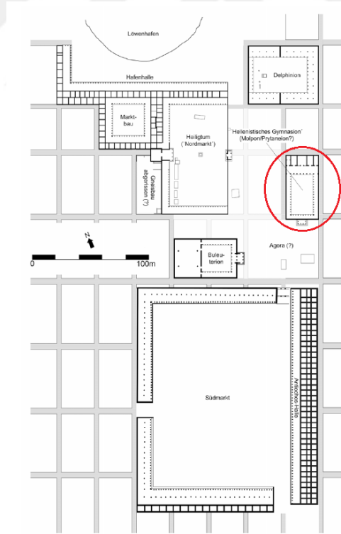
Şekil 24: Miletos Hellenistik Peristyl (Emme, 2013: 453.).
