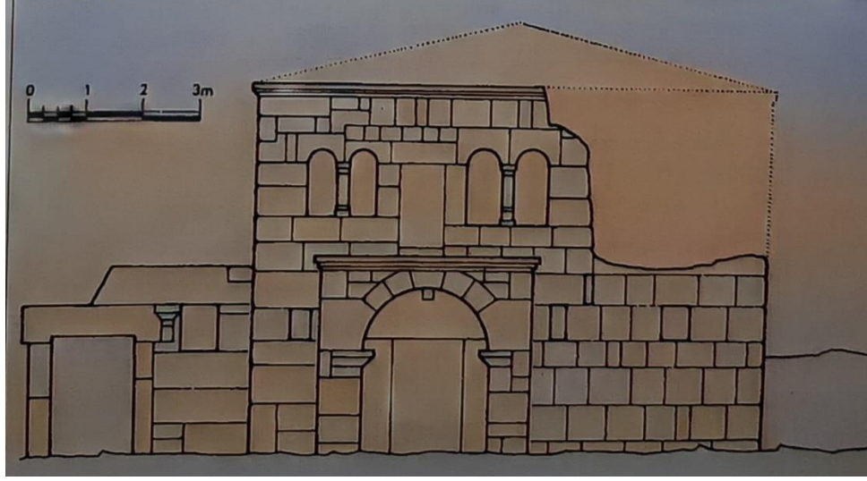
Şekil 81: Silifke Gökale de Bir Bizans Konutu (Eyice, 1999: 213.).
