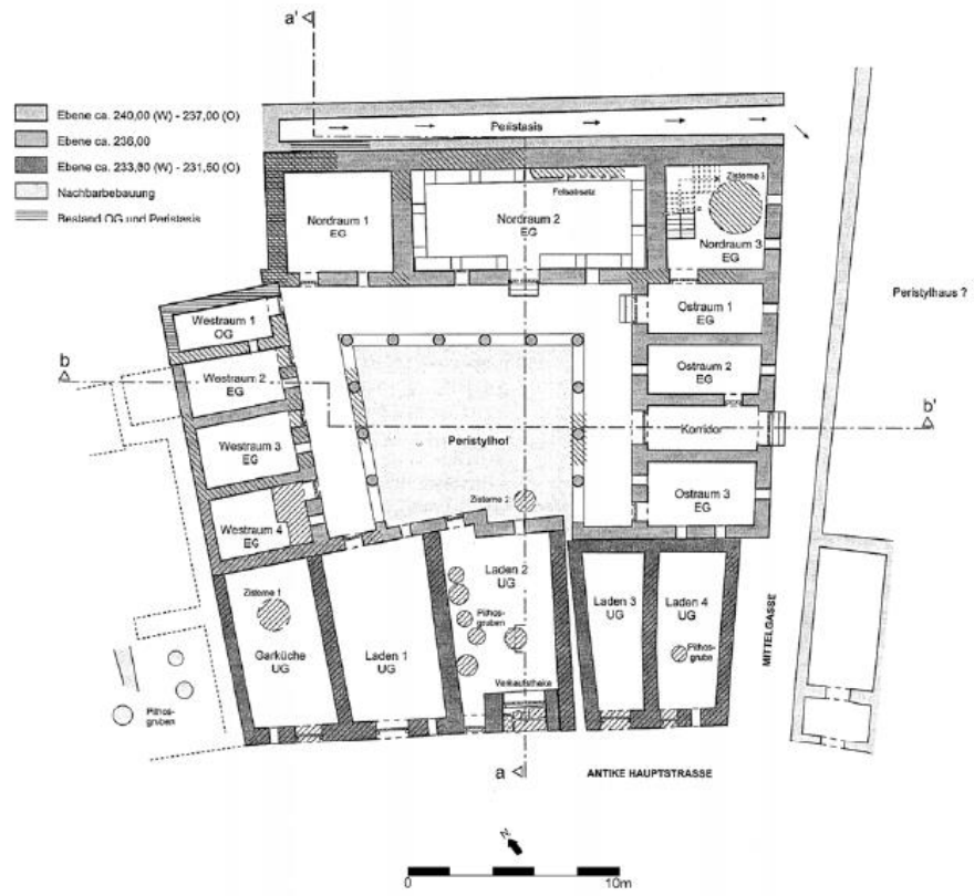
Şekil 30: Pergamon Podium Salonlu Bina Planı (Emme, 2013: 186.).
