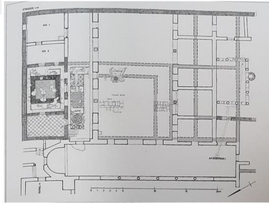
Piskoposluk Sarayı Plan
