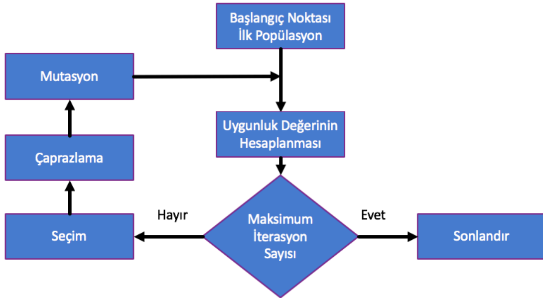
Şekil 13. Genetik algoritma akış şeması
