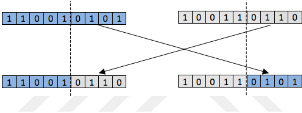
Şekil 14. Genetik aprazlama örneęi
