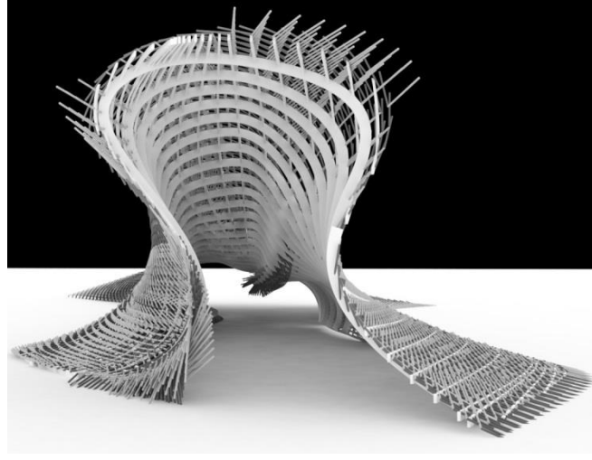
Şekil 5.93 : Strüktür ve örgü birleşimi.
