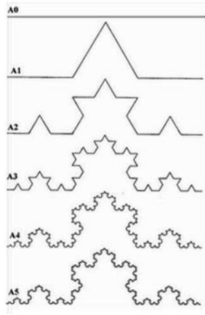
Şekil 3.5 : Koch eğrisi, (Koçak, 2014).
