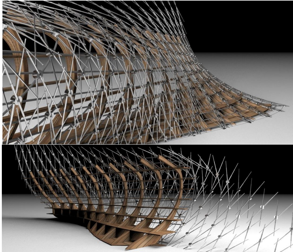
Şekil 5.101 : Ahşap taşıyıcı sistemi, çelik kablo ve örüntüyü oluşturan mekanik modüller.
