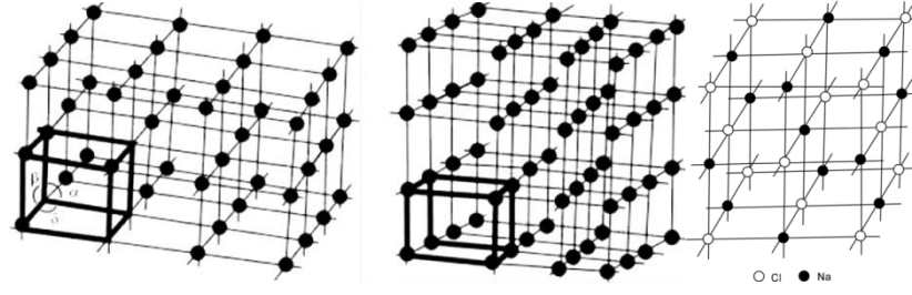
Şekil 4.3 : Kristallerde kafes yapısı, (Yalçın, 2001).
