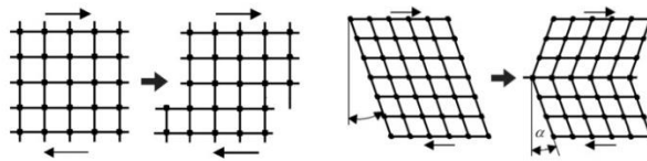
Şekil 4.8 : Tek kristalin plastik şekil değiştirmesi, (Erişir, 2012).
