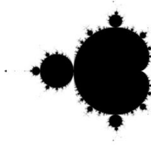
Şekil 3.6 : Mandelbrot kümesi, (URL-3).
