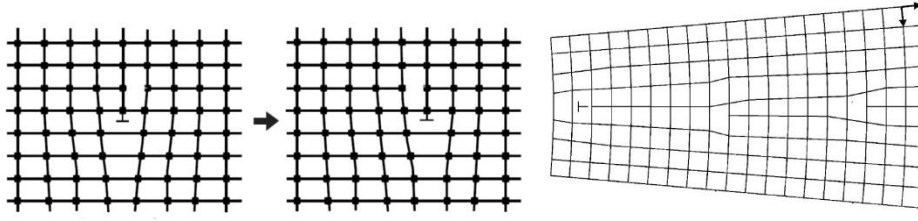
Şekil 4.9 : Dislokasyon, (Erişir, 2012).
