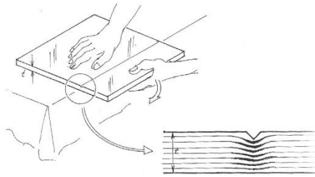
Şekil 4.11 : Camın çizilerek koparılma işlemi (kuvvet çizgilerinin yoğunlaşması), (Çakmak, 2011).
