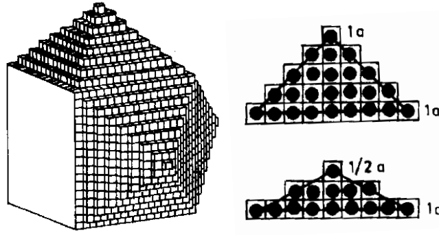
Şekil 4.5 : Birimde düzenli kafes hacim yapısı, (Yalçın, 2001).
