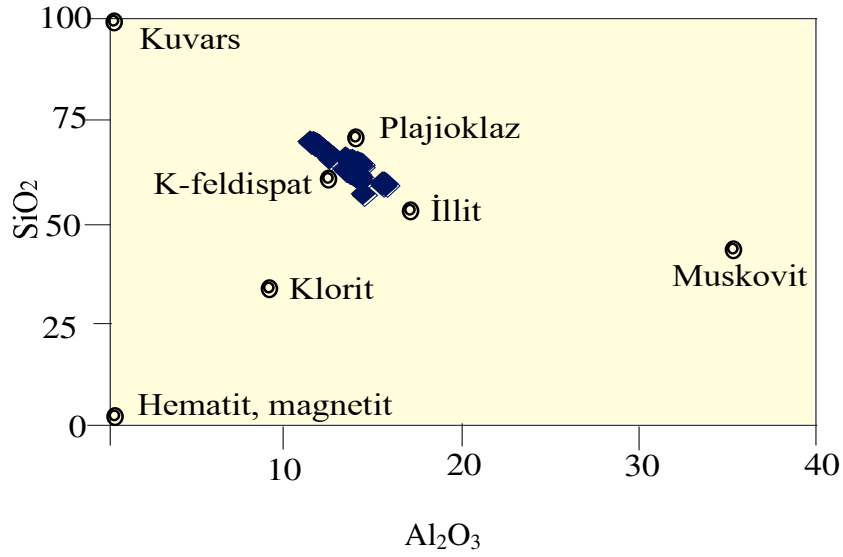
Şekil 3.4. İncelenen örneklerin Al 2 O 3 ve SiO 2 konsantrasyonu (Kuvars, plajiolaz, K-feldispat, illit, muskovit, klorit ve hematit, magnetitin diyagramdaki konumları (Cullers ve Podkovyrov, 2002'den alınmıştır.)
