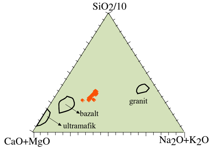
Şekil 3.6. İncelenen örneklerin (CaO+MgO)+SiO_2/10+(Na_2O+K_2O) diyagramı kullanılarak sınıflandırılması
