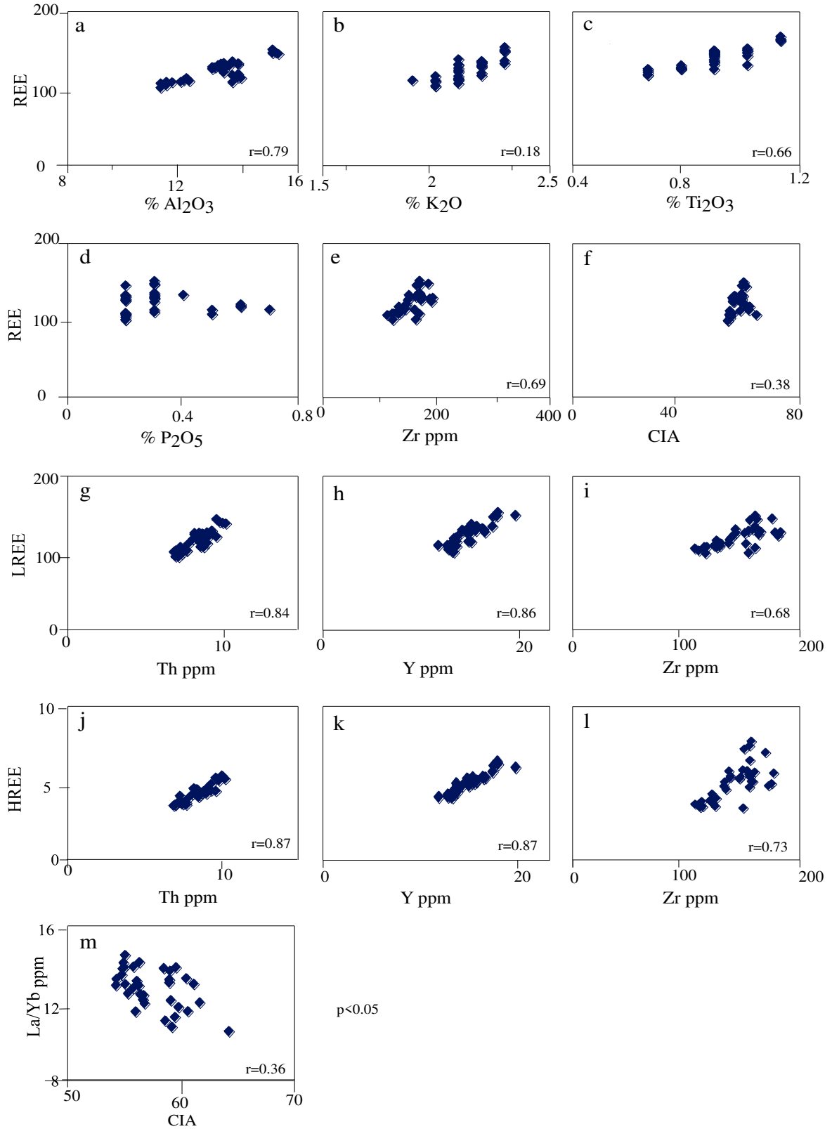
Şekil 3.12. İncelenen örneklerin N.T.E içeriği ile (a) \text{Al}_2\text{O}_3 , (b) \text{K}_2\text{O} , (c) \text{Ti}_2\text{O}_3 , (d) \text{P}_2\text{O}_5 , (e) Zr, (f) CIA, H.N.T.E içeriği ile (g) Th, (h) Y, (i) Zr, A.N.T.E içeriği ile (j) Th, (k) Y, (l) Zr ve La/Yb içeriği ile (m) CIA içeriği arasındaki ilişki
