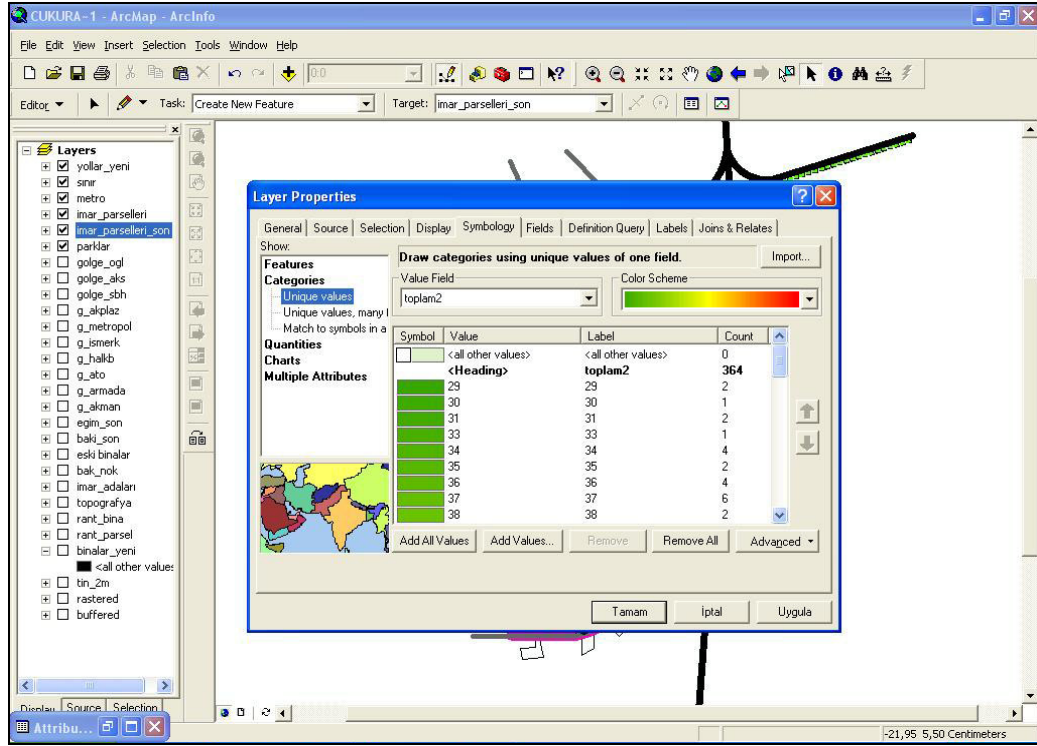
Şekil 4.25. ArcGIS 9.0 ArcMap içinden çıktıya hazırlanan verilerin gösterim tekniğinin (symbology) hazırlanması.
