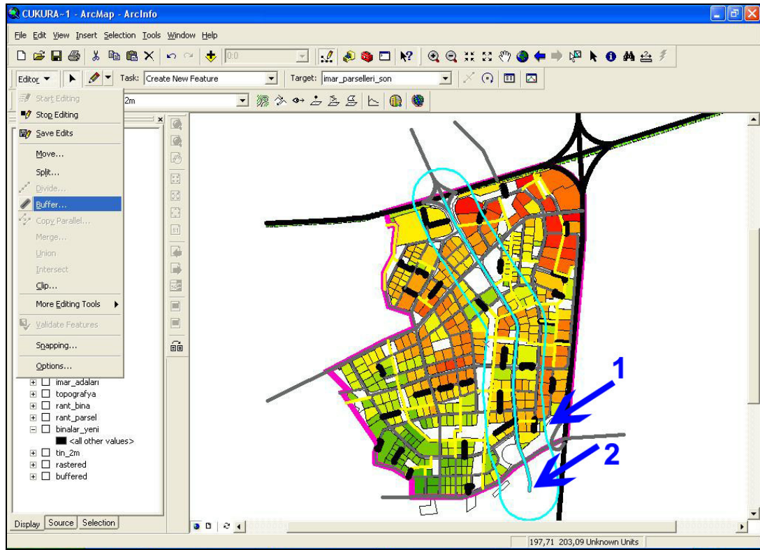
Şekil 4.20. ArcGIS 9.0 ArcMap içinden tampon “buffer” analizinin çalıştırılması
