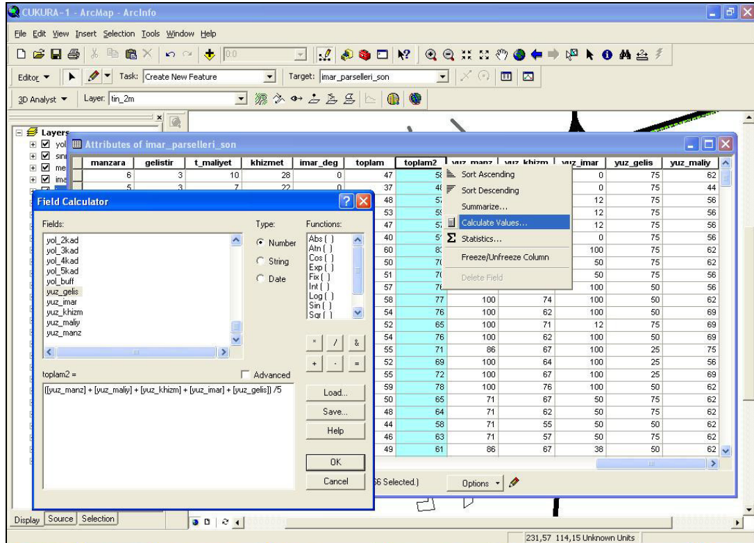
Şekil 4.24. ArcGIS 9.0 ArcMap içinden veritabanında bulunan farklı kolonların puanlarının toplanarak yeni bir sentez (toplam etkilenme) kolonuna aktarılışı
