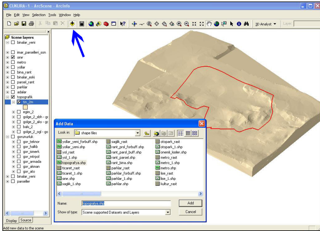
Şekil 4.5. ArcGIS 9.0 ArcScene'e program dışından veritabanları ile ilişkili vektörel veri çağırma işlemi
