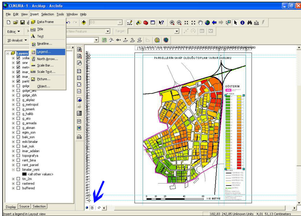
Şekil 4.26. ArcGIS 9.0 ArcMap içinden çıktıya hazırlanan verilerin “layout” ile harita olarak düzenlenerek çıktıya gönderilmesi
