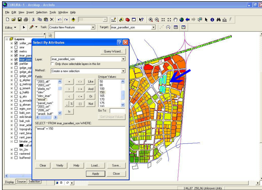
Şekil 4.22. ArcGIS 9.0 ArcMap içinden veritabanındaki ortak niteliklere göre obje sorgusu (select by attributes) işleminin yapılışı
