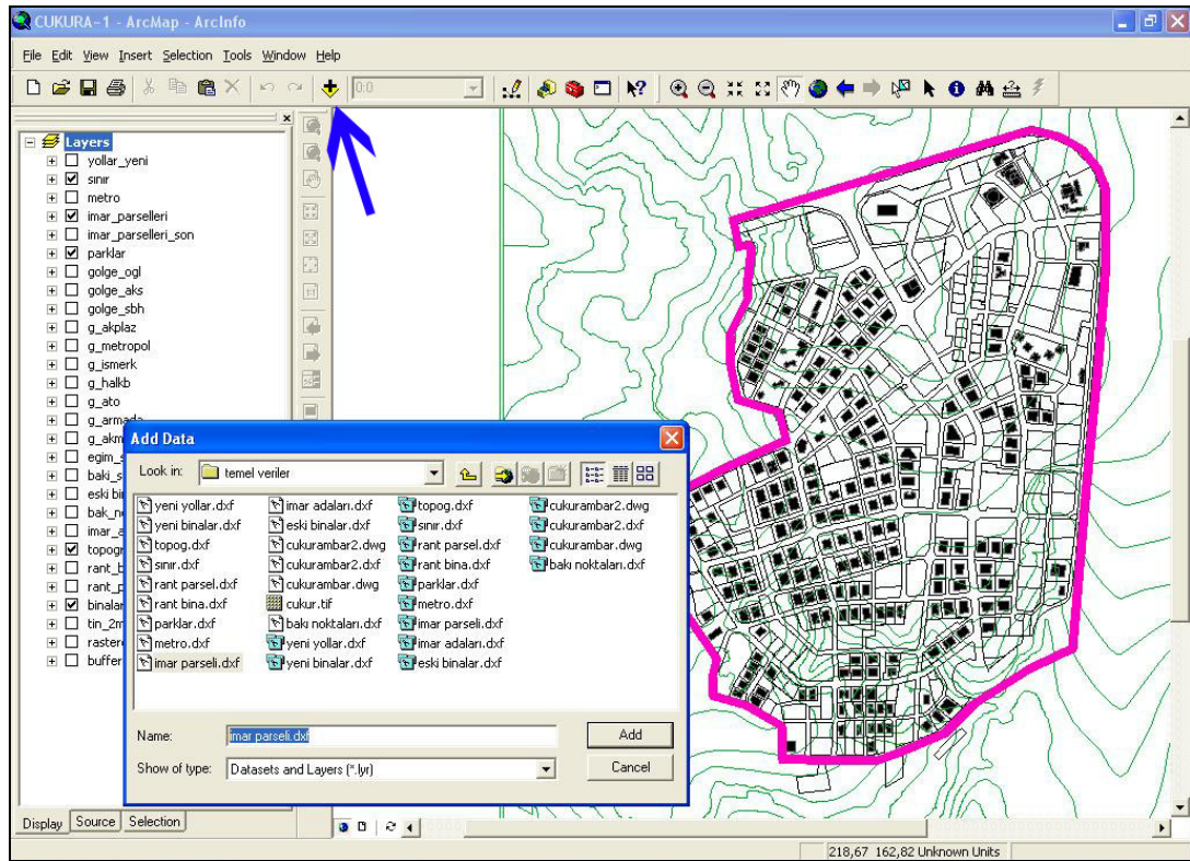
Şekil 4.1. ArcGIS 9.0 ArcMap'e program dışından vektörel veri çağırma işlemi
