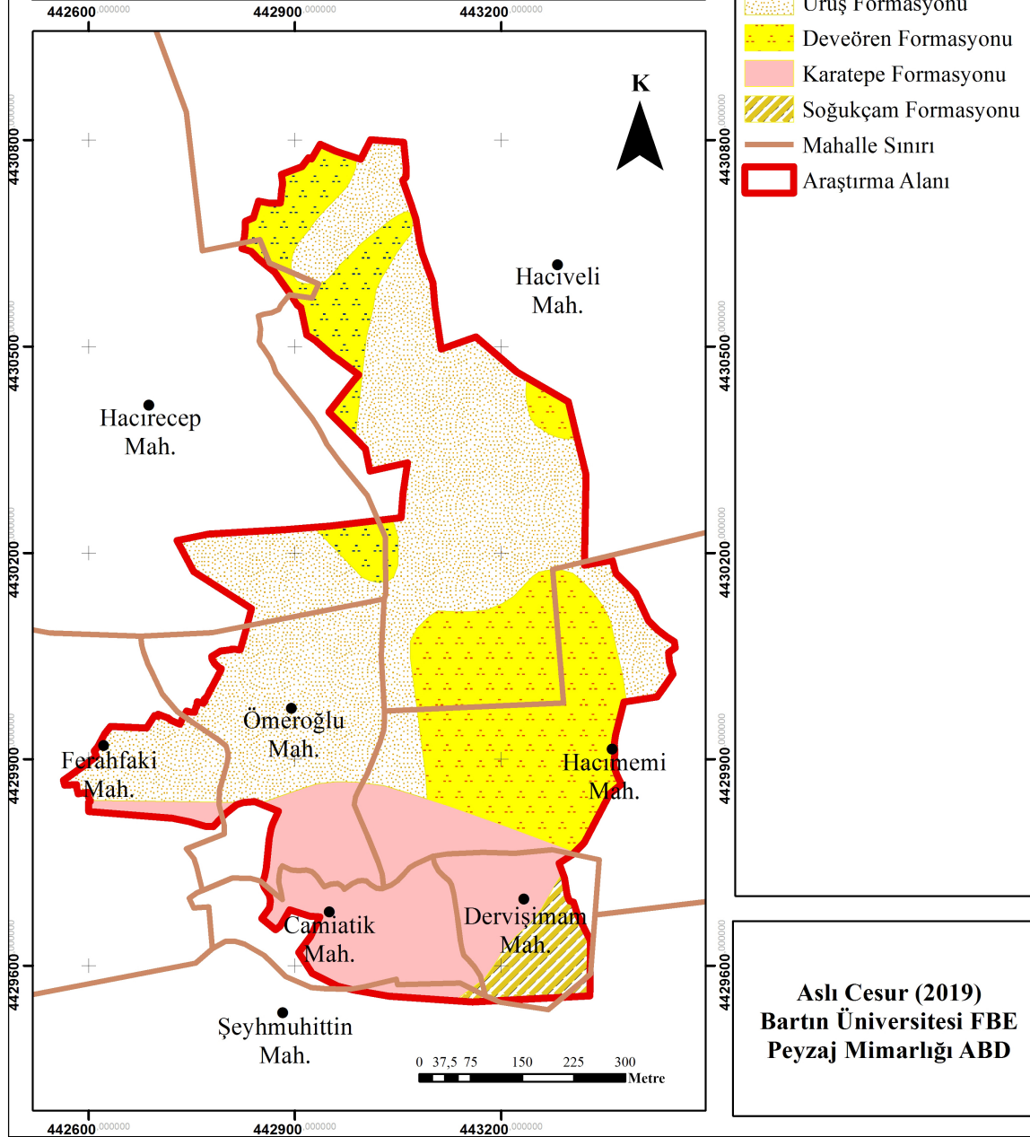
Şekil 4.4: Çalışma alanına ait jeoloji haritası.
