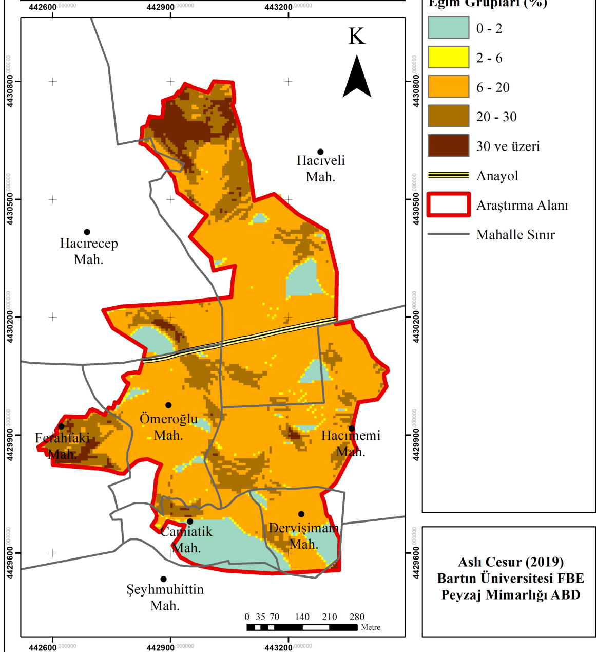
Şekil 4.1: Çalışma alanına ait eğim grupları haritası.
