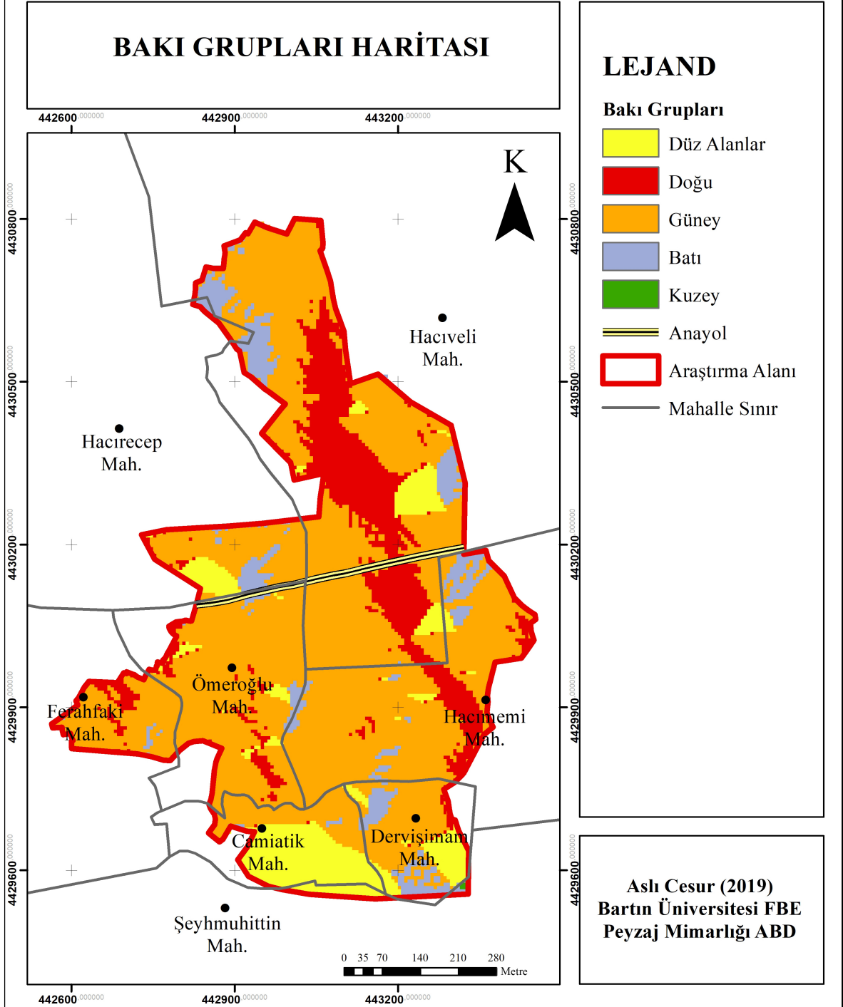
Şekil 4.2: Çalışma alanına ait bakı grupları haritası.
