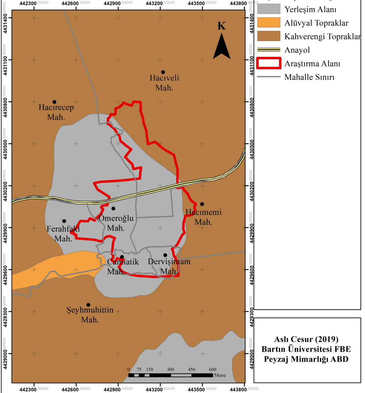
Şekil 4.6: Çalışma alanı ve yakın çevresine ait büyük toprak grupları haritası.
