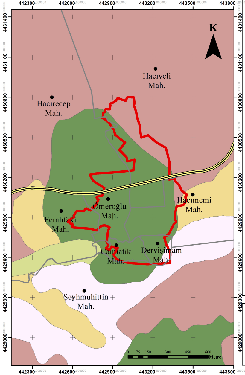
Şekil 4.7: Çalışma alanı ve yakın çevresine ait arazi yetenek sınıfları haritası.
